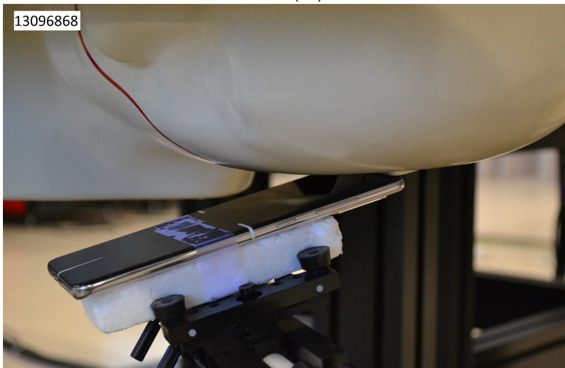
Left Tilt (15°)
