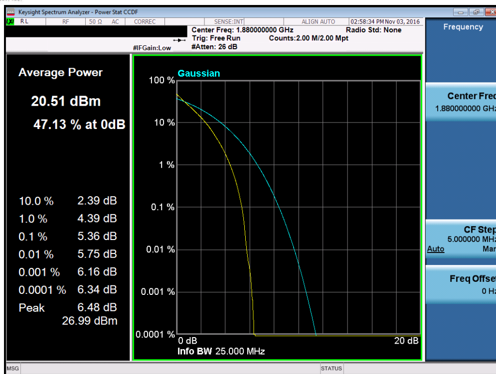
Plot 7-174. PAR Plot (Band 2 – 15.0MHz QPSK – RB Size 75)
