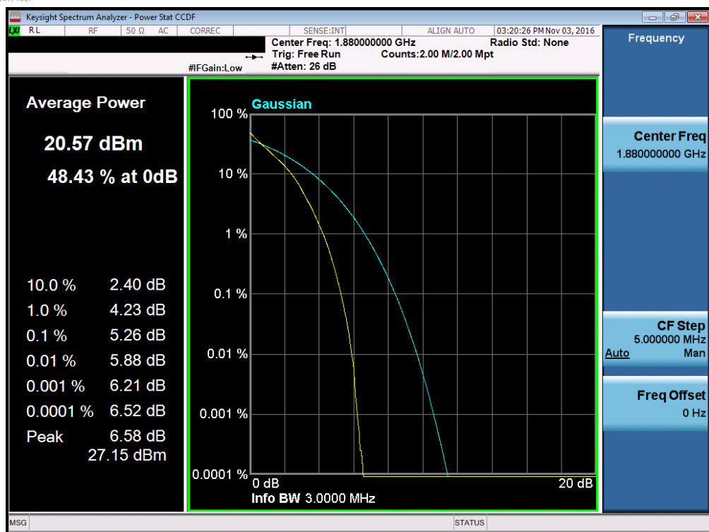
Plot 7-168. PAR Plot (Band 2 – 3.0MHz QPSK – RB Size 15)
