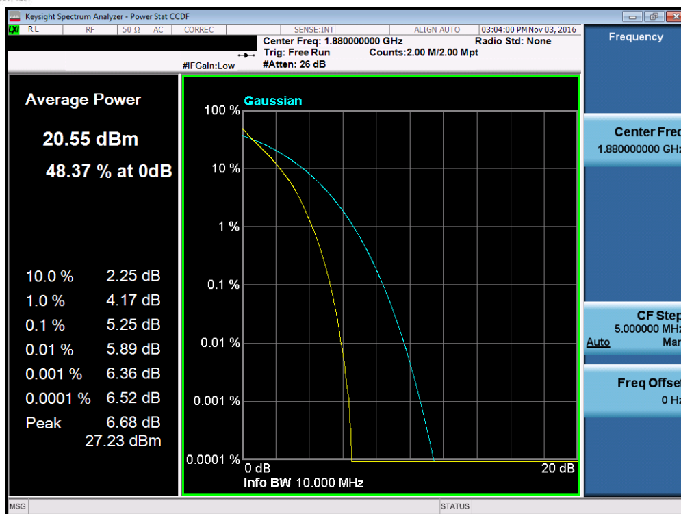
Plot 7-172. PAR Plot (Band 2 – 10.0MHz QPSK – RB Size 50)
