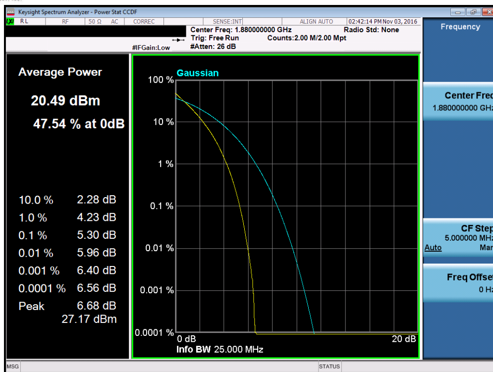
Plot 7-176. PAR Plot (Band 2 – 20.0MHz QPSK – RB Size 100)
