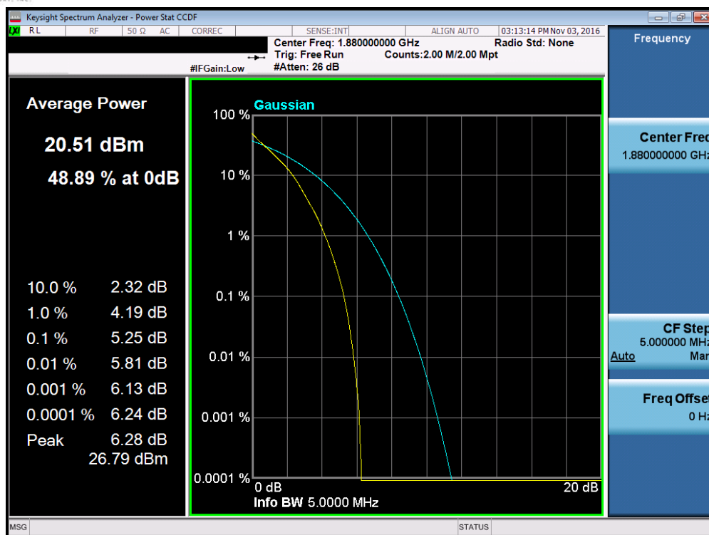
Plot 7-170. PAR Plot (Band 2 – 5.0MHz QPSK – RB Size 25)
