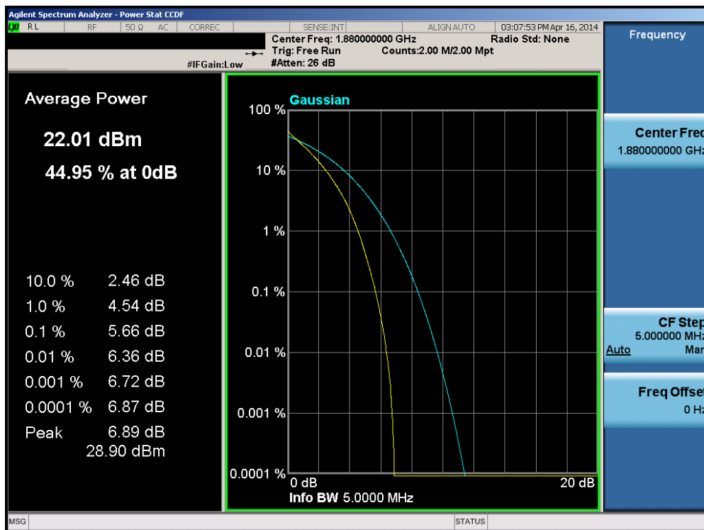
Plot 6-230. PAR Plot (Band 2 – 5.0MHz QPSK – RB Size 25)
