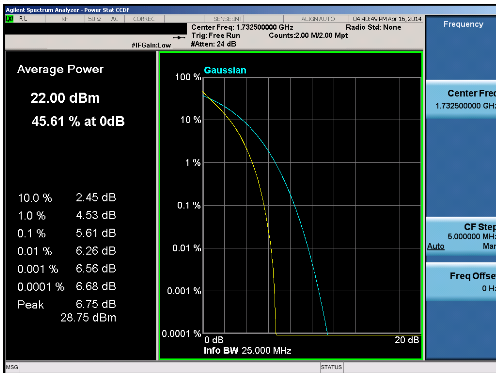
Plot 6-224. PAR Plot (Band 4 – 20.0MHz QPSK – RB Size 100)
