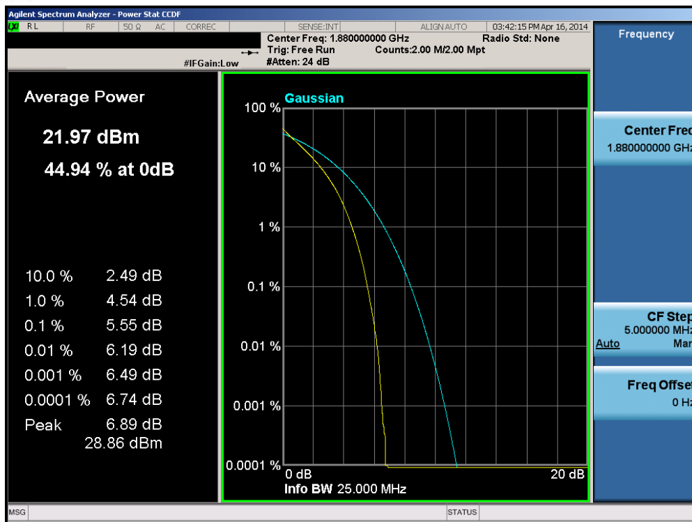
Plot 6-236. PAR Plot (Band 2 – 20.0MHz QPSK – RB Size 100)
