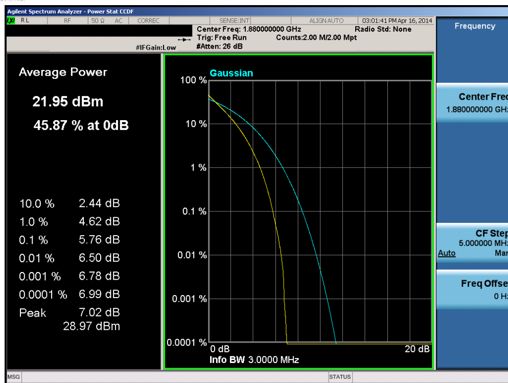
Plot 6-228. PAR Plot (Band 2 – 3.0MHz QPSK – RB Size 15)
