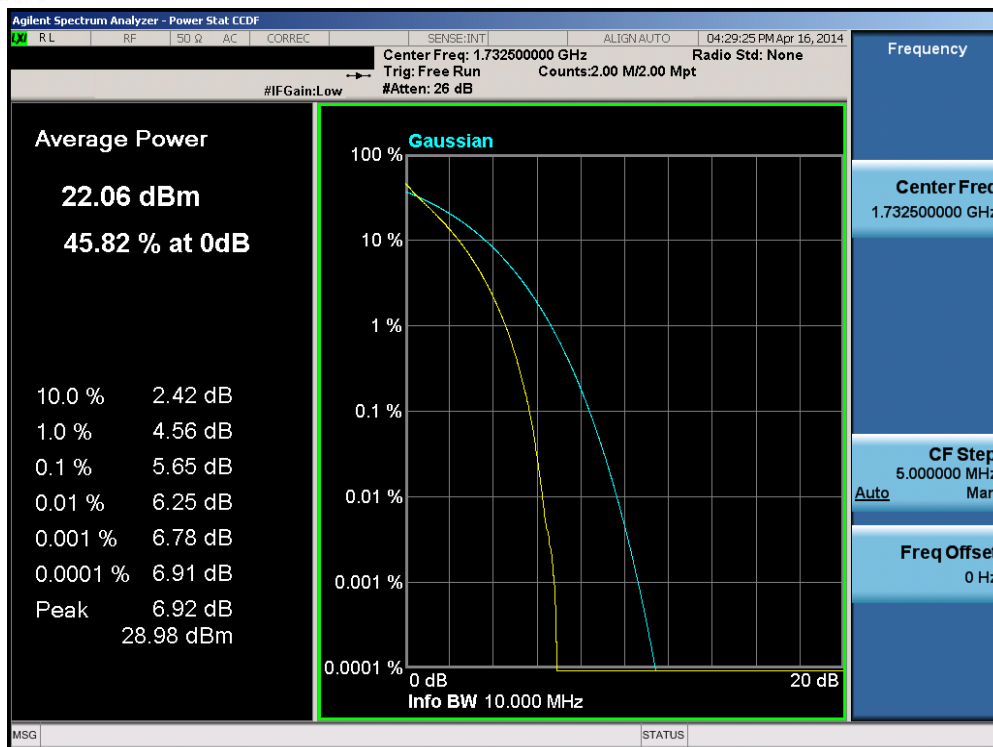
Plot 6-220. PAR Plot (Band 4 – 10.0MHz QPSK – RB Size 50)
