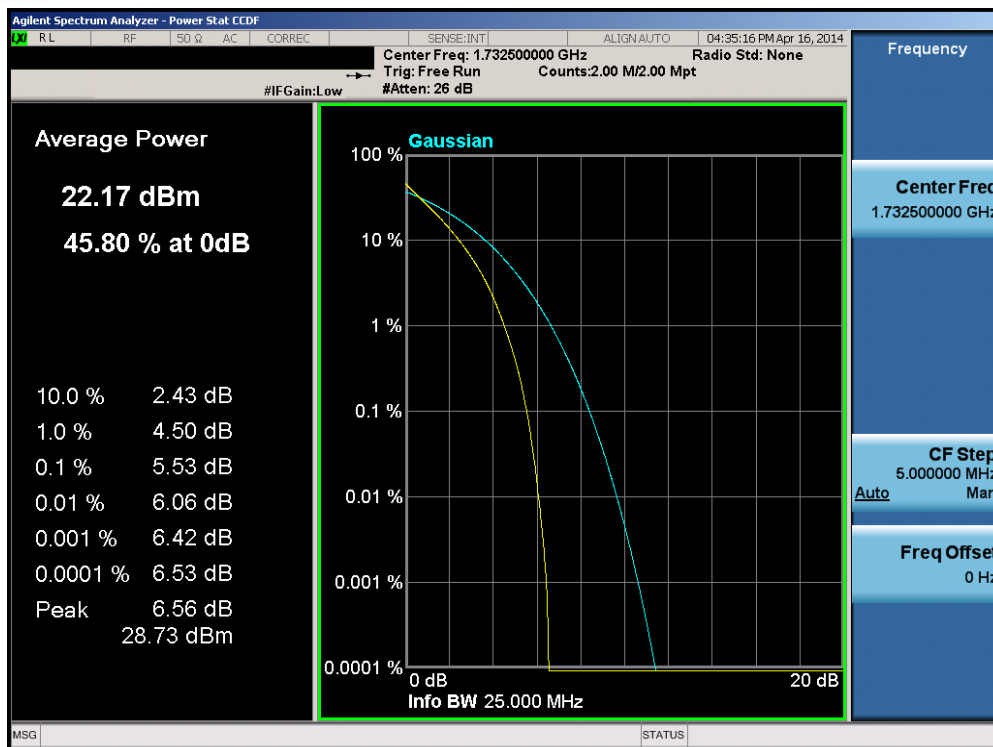
Plot 6-222. PAR Plot (Band 4 – 15.0MHz QPSK – RB Size 75)
