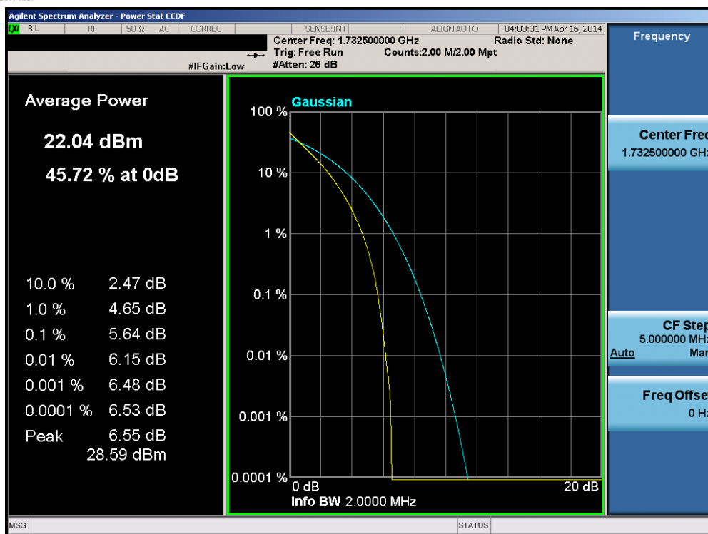
Plot 6-214. PAR Plot (Band 4 – 1.4MHz QPSK – RB Size 6)
