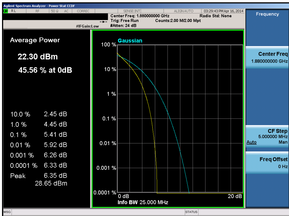
Plot 6-234. PAR Plot (Band 2 – 15.0MHz QPSK – RB Size 75)
