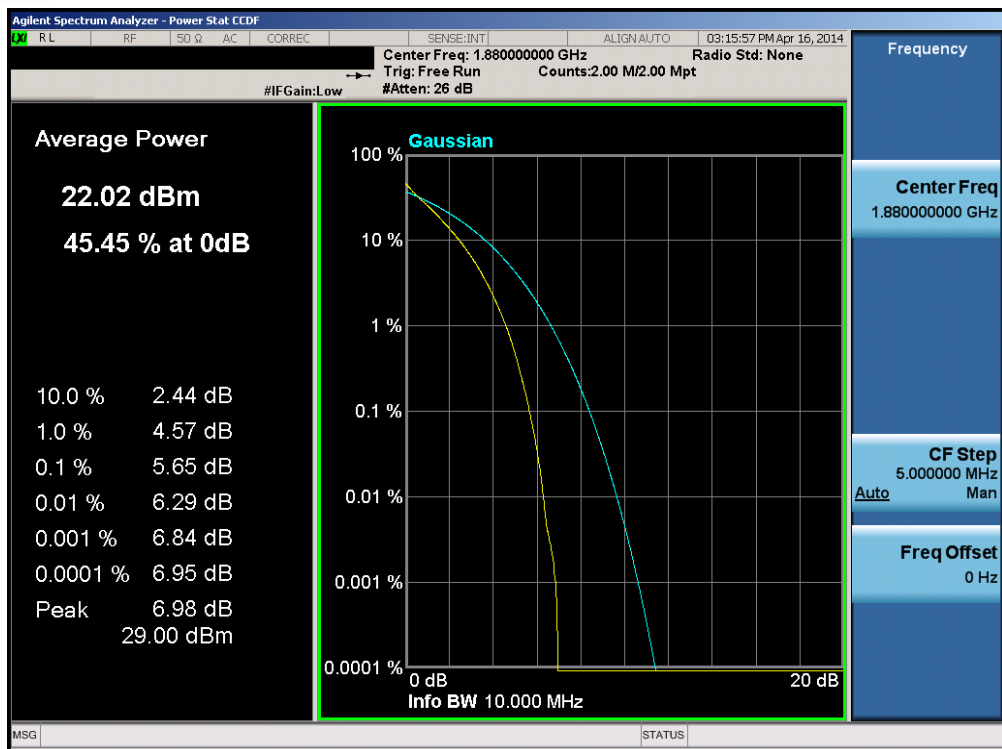
Plot 6-232. PAR Plot (Band 2 – 10.0MHz QPSK – RB Size 50)
