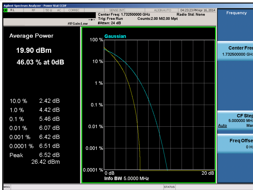
Plot 6-218. PAR Plot (Band 4 – 5.0MHz QPSK – RB Size 25)
