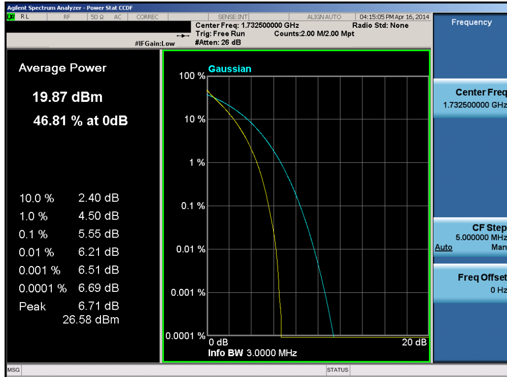
Plot 6-216. PAR Plot (Band 4 – 3.0MHz QPSK – RB Size 15)
