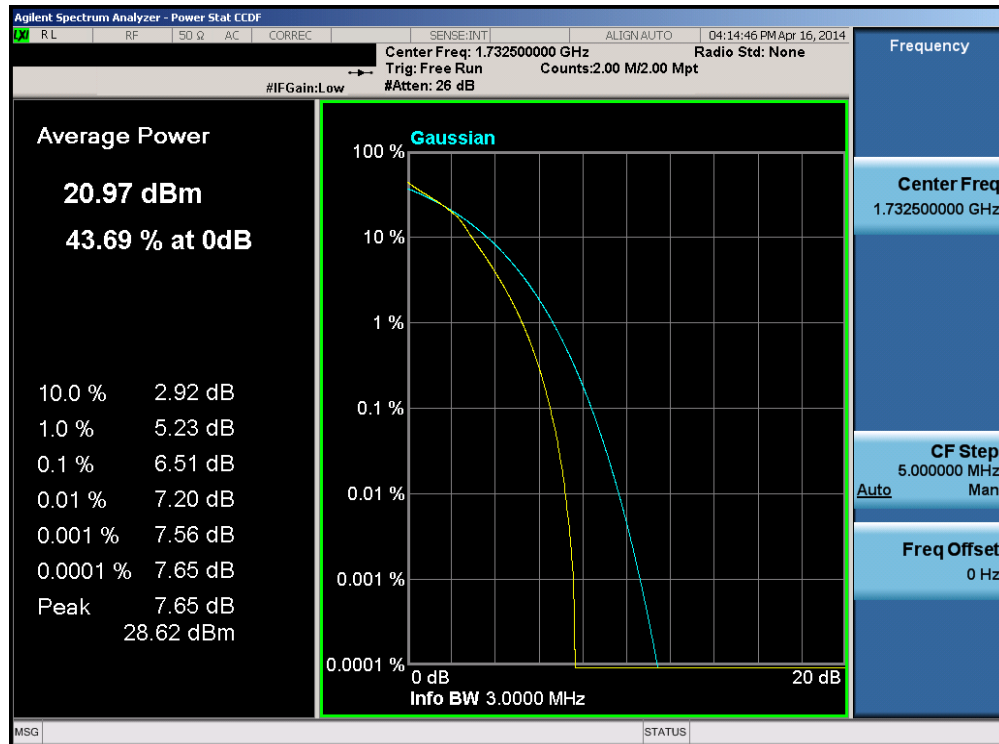
Plot 6-217. PAR Plot (Band 4 – 3.0MHz 16-QAM – RB Size 15)
