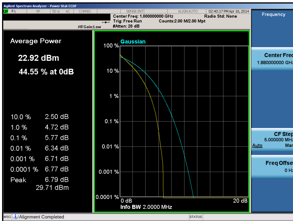
Plot 6-226. PAR Plot (Band 2 – 1.4MHz QPSK – RB Size 6)
