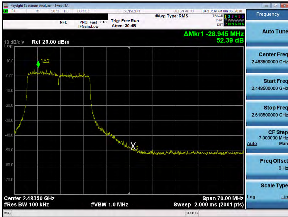
Plot 7-64. Band Edge Plot SISO ANT1 (802.11ax SU – Ch. 11)
