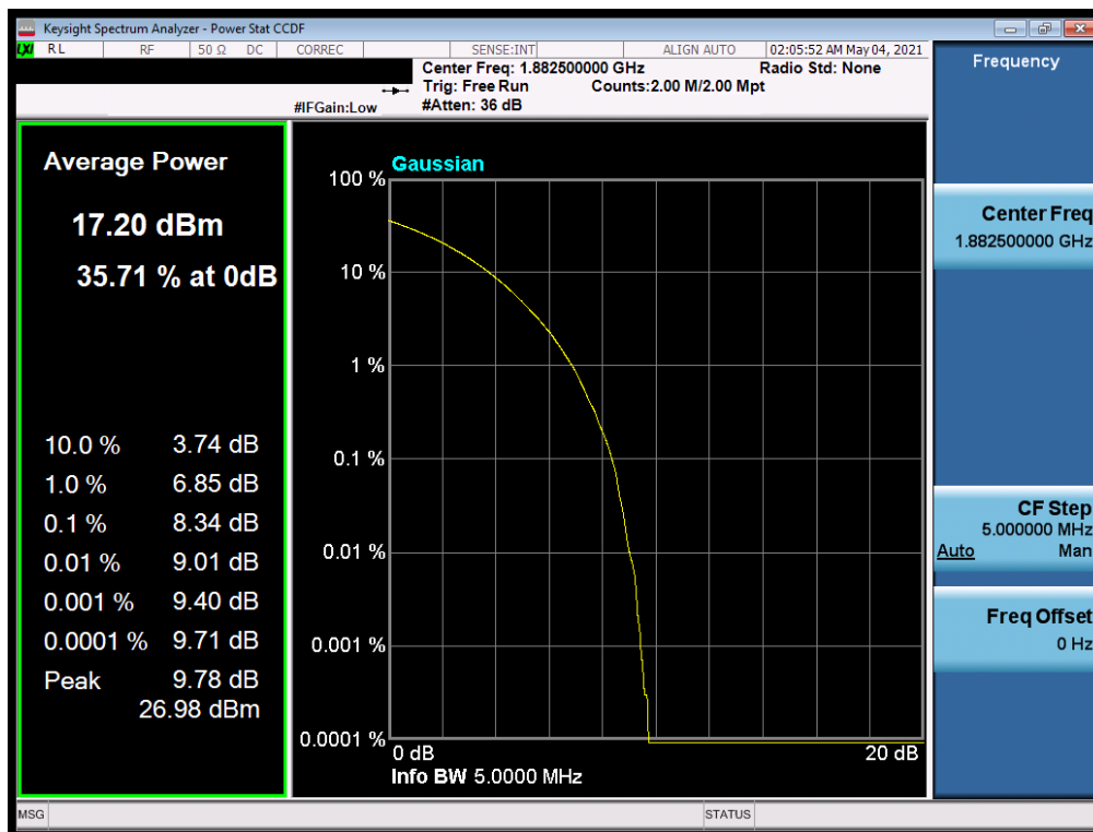
Plot 7-284. PAR Plot (NR Band n25/2 - 5.0MHz CP-OFDM 256-QAM - Full RB)
