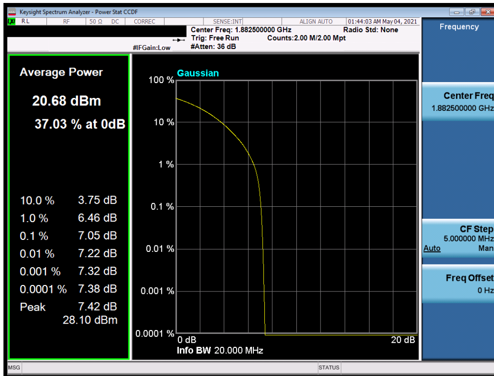
Plot 7-274. PAR Plot (NR Band n25/2 - 20.0MHz CP-OFDM QPSK - Full RB)
