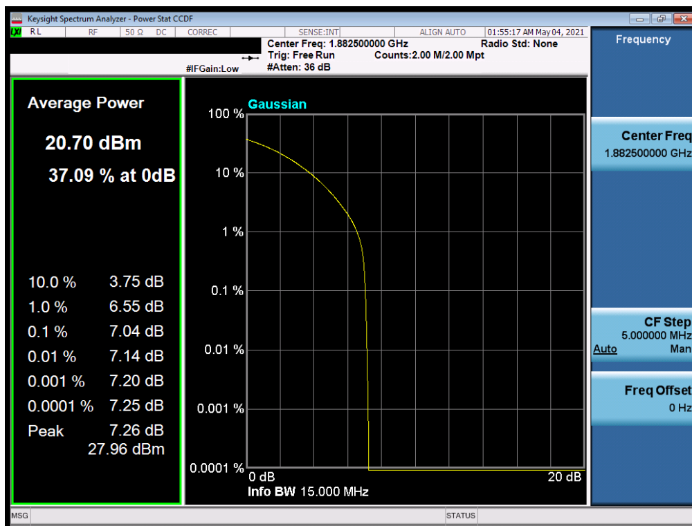
Plot 7-277. PAR Plot (NR Band n25/2 - 15.0MHz CP-OFDM QPSK - Full RB)
