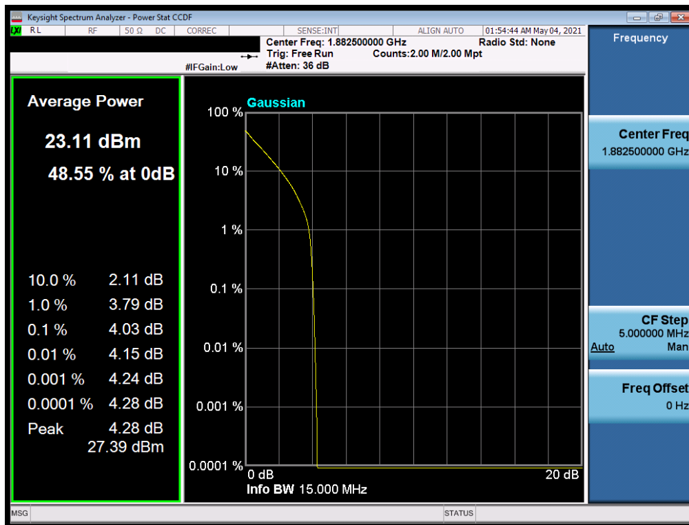
Plot 7-276. PAR Plot (NR Band n25/2 - 15.0MHz DFT-s-OFDM BPSK - Full RB)
