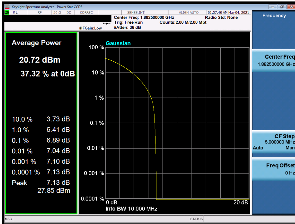
Plot 7-280. PAR Plot (NR Band n25/2 - 10.0MHz CP-OFDM QPSK - Full RB)
