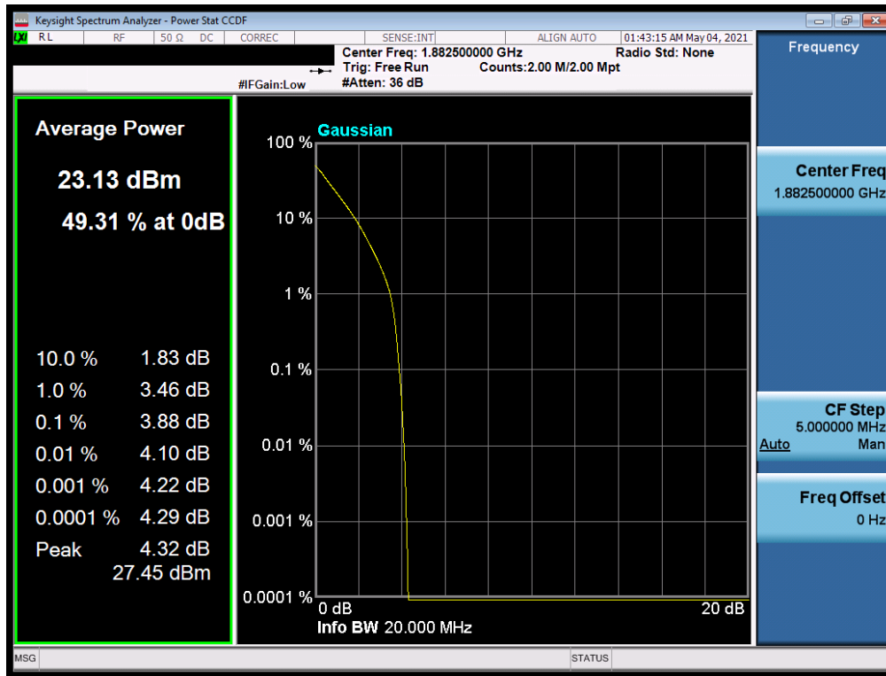
Plot 7-273. PAR Plot (NR Band n25/2 - 20.0MHz DFT-s-OFDM BPSK - Full RB)
