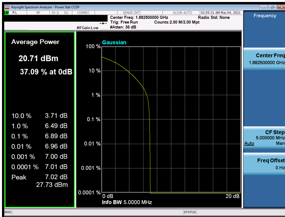
Plot 7-283. PAR Plot (NR Band n25/2 - 5.0MHz CP-OFDM QPSK - Full RB)
