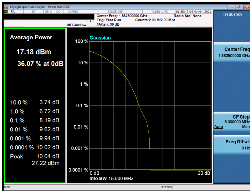
Plot 7-278. PAR Plot (NR Band n25/2 - 15.0MHz CP-OFDM 256-QAM - Full RB)
