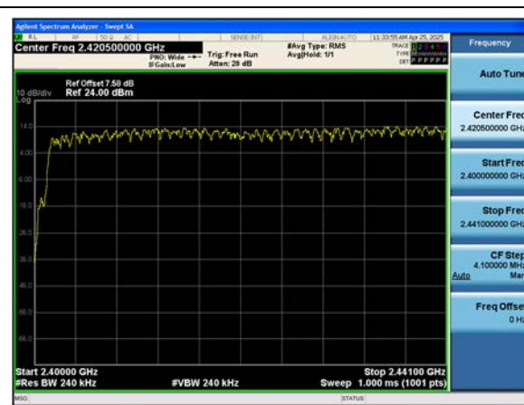
Dual ANT.1 \pi /4DQPSK (2.4 GHz - 2.441 GHz)
