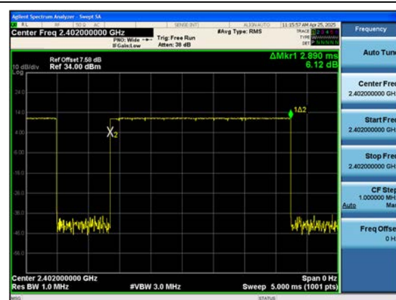
Dual ANT.1 \pi/4 DQPSK : Dwell Time(Ch. 0)
