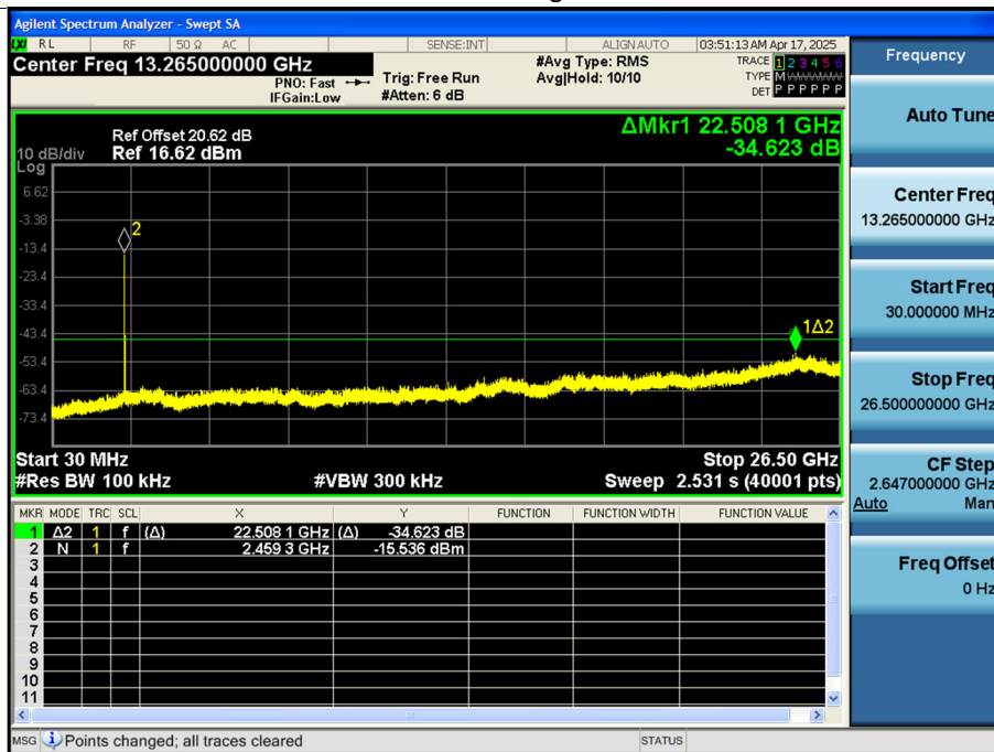
[ANT. 2] 802.11g_Ch.12
