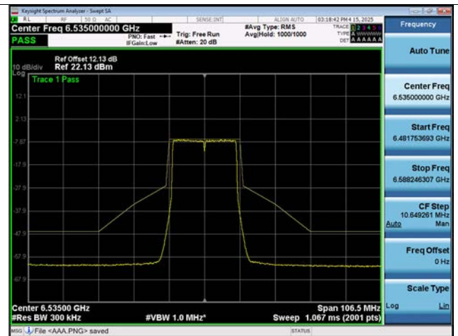
802.11ax HE20M Ch.117(6535 MHz) 242 Tones 61 RU
