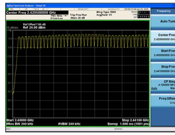
ANT.1 8DPSK (2.4 GHz - 2.441 GHz)
