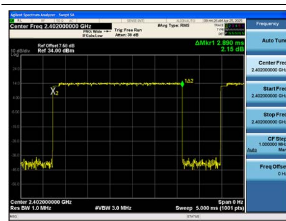
ANT.1 \pi/4 DQPSK : Dwell Time(Ch. 0)
