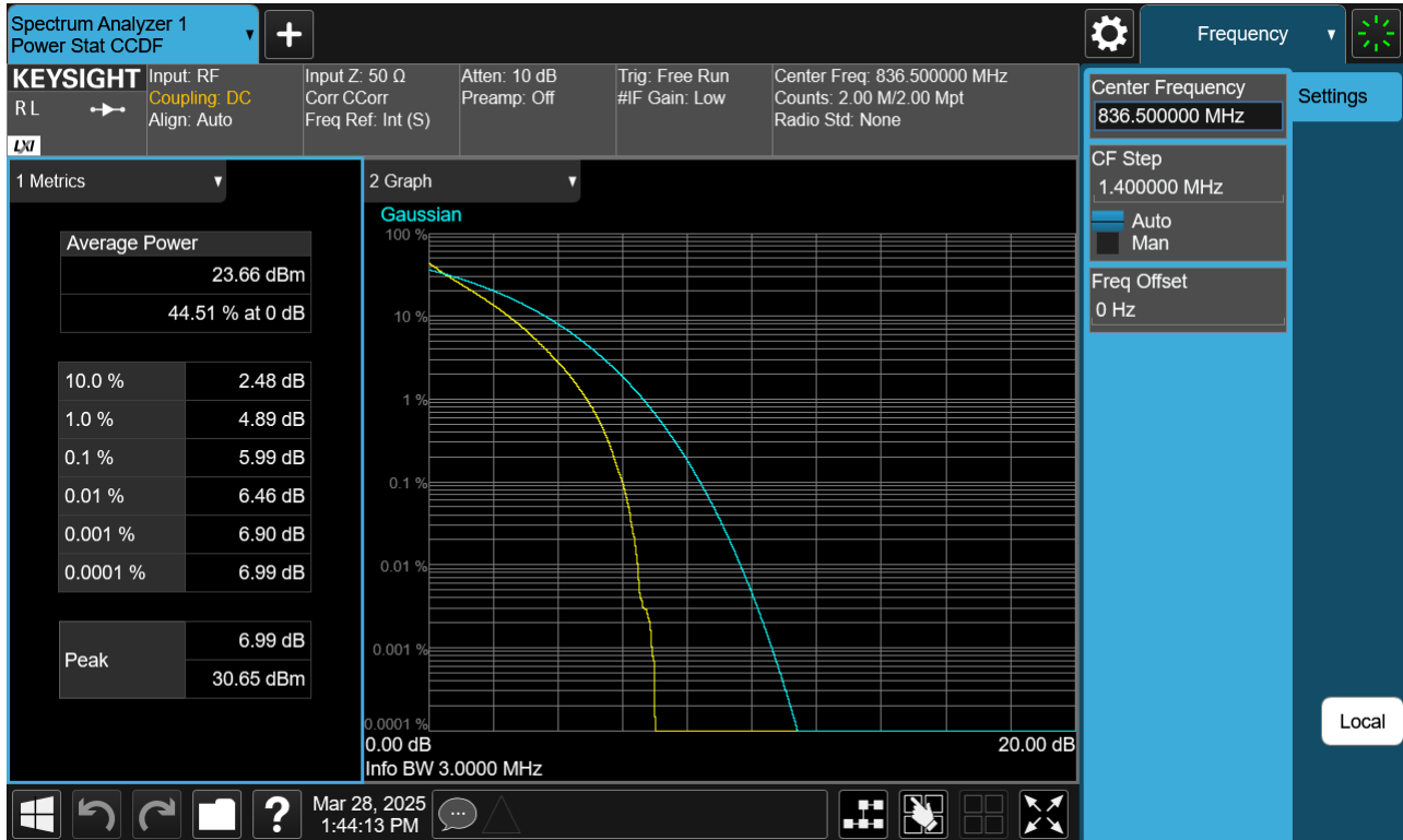
BAND 26. PAR Plot (3 M BW Ch.26915 QPSK_RB15_0)
