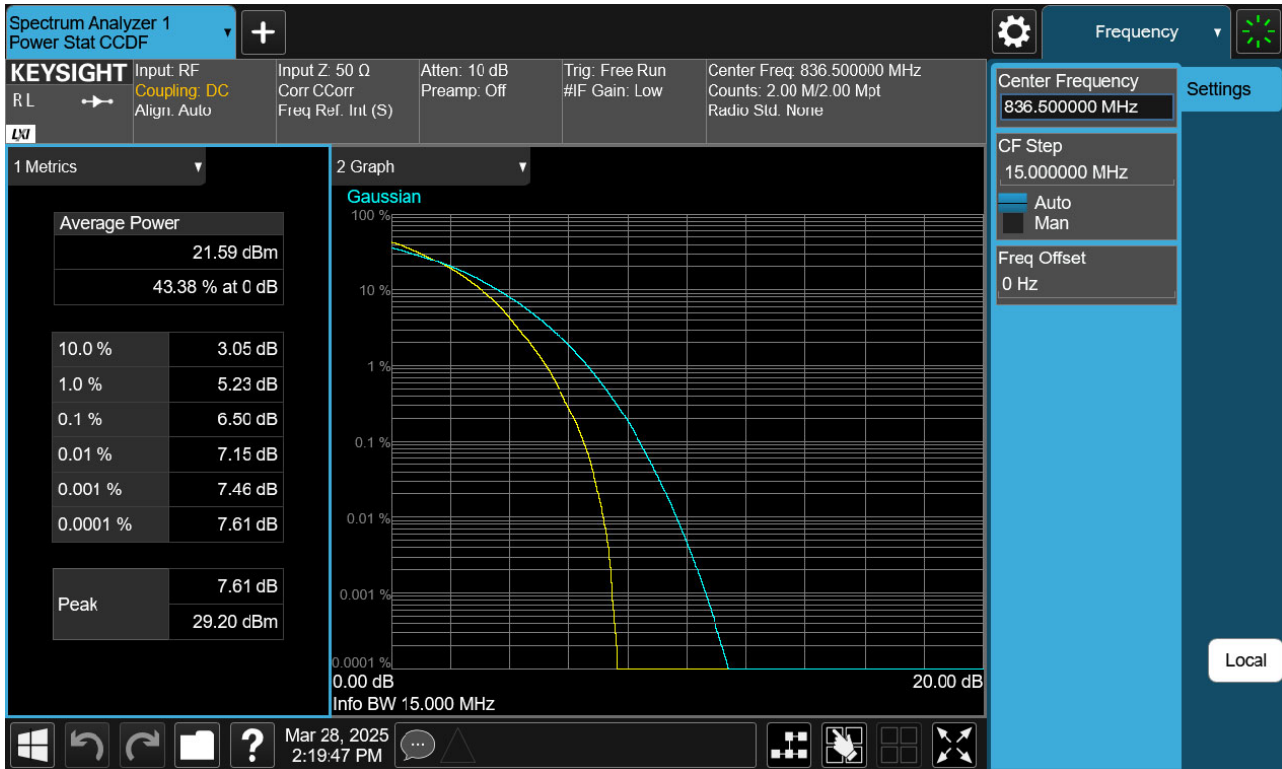
BAND 26. PAR Plot (15 M BW Ch.26915 64QAM RB 75_0)
