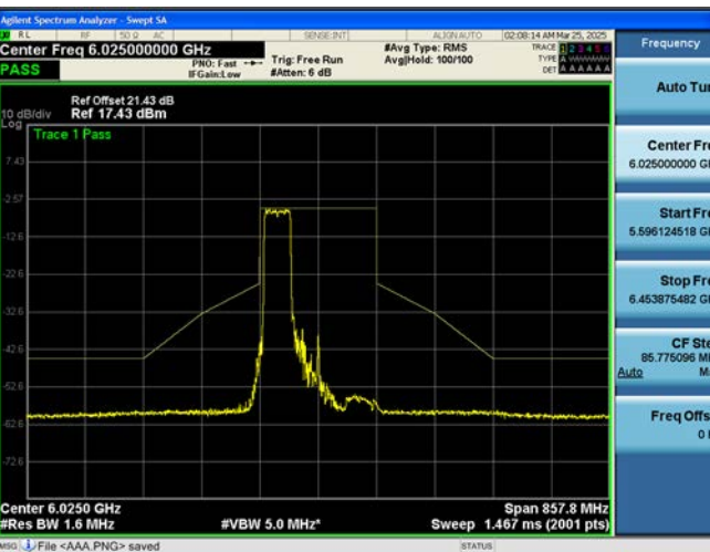
802.11be EHT160M Ch.Ch.15(6025 MHz) 484 Tones 65 RU
