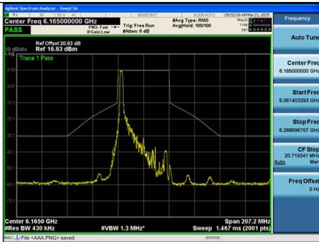
802.11be EHT40M Ch.43(6165 MHz) 106 Tones 53 RU
