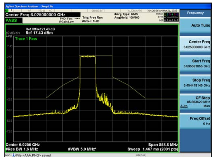
802.11be EHT160M Ch.Ch.15(6025 MHz) 996 Tones 67 RU
