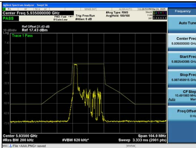
802.11be EHT20M Ch.2(5935 MHz) 106 Tones 53 RU
