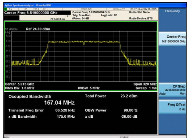
Bandwidth 160M 2x996Tone Ch.163(5815 MHz) SU
