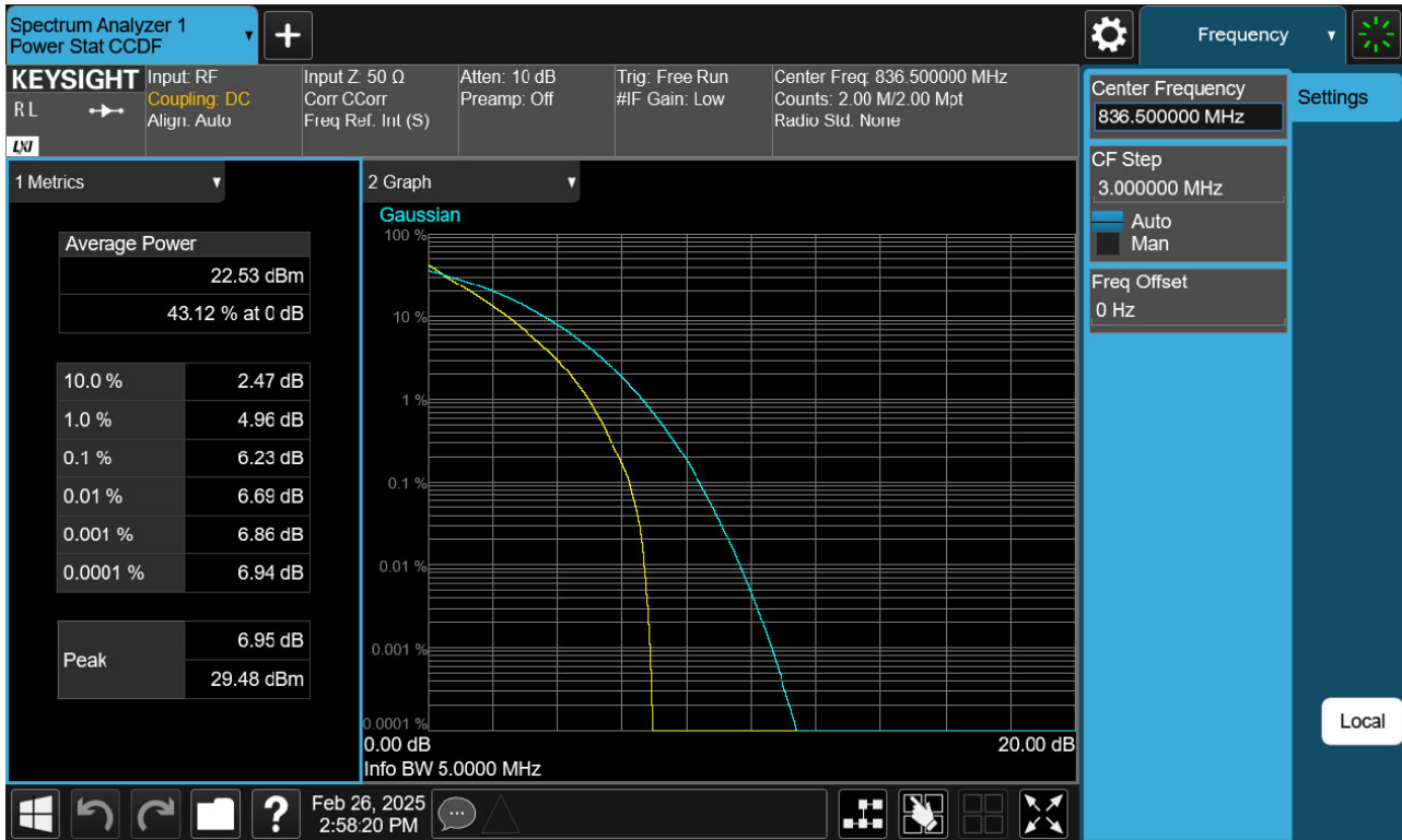
BAND 26. PAR Plot (5 M BW Ch.26915 QPSK_RB25_0)
