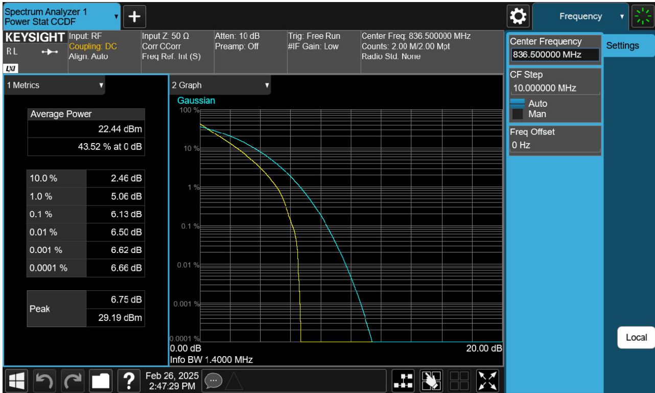
BAND 26. PAR Plot (1.4 M BW Ch.26915 QPSK_RB6_0)
