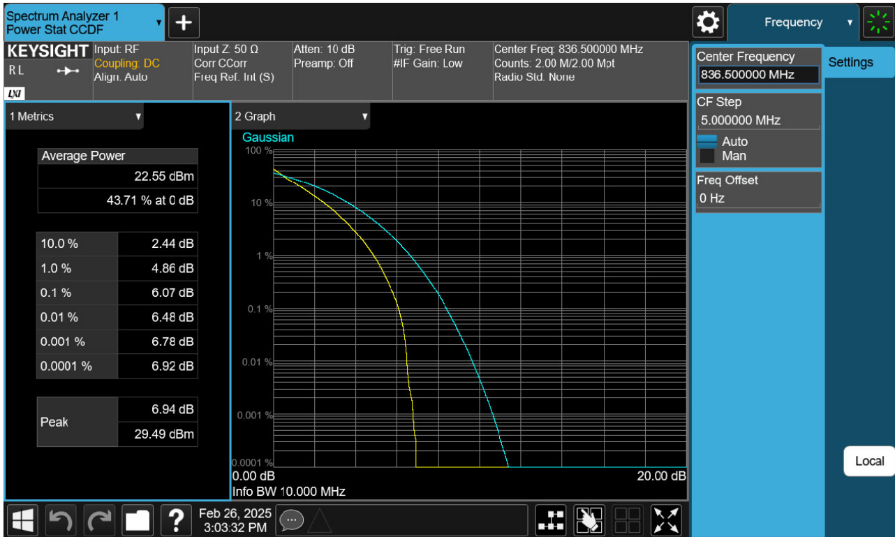
BAND 26. PAR Plot (10 M BW Ch.26915 QPSK_RB50_0)
