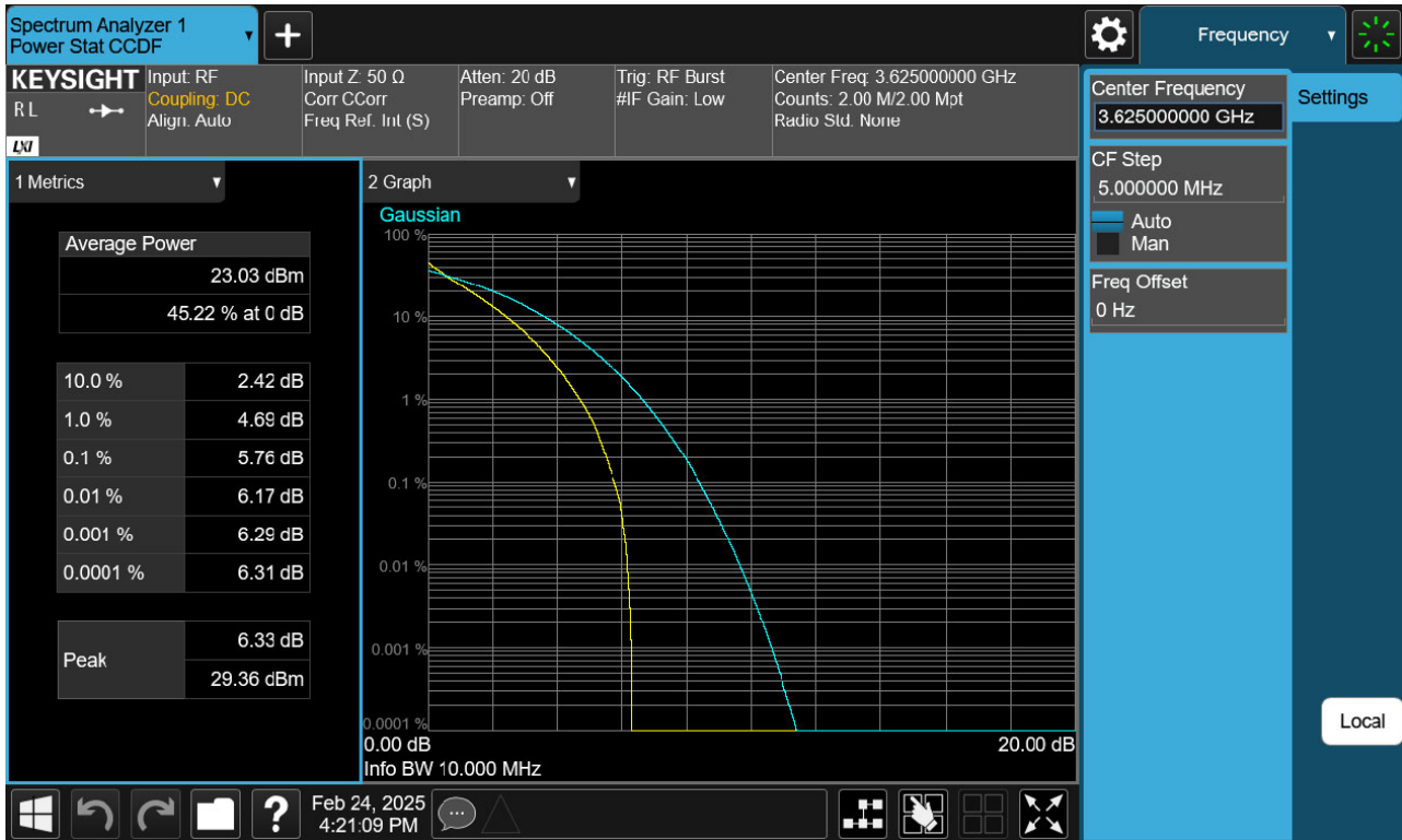
BAND 48. PAR Plot (10 M BW_Ch.55990_QPSK_RB50_0)
