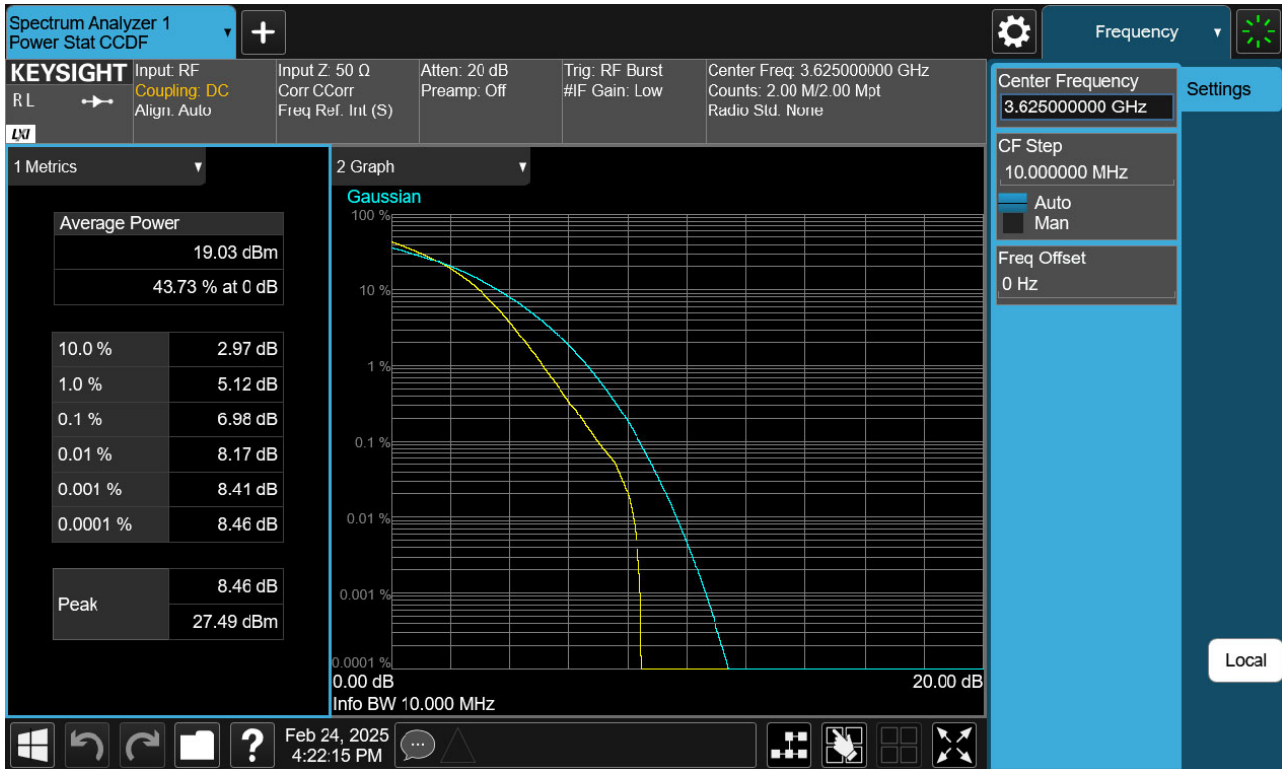
BAND 48. PAR Plot (10 M BW_Ch.55990_256QAM_RB50_0)
