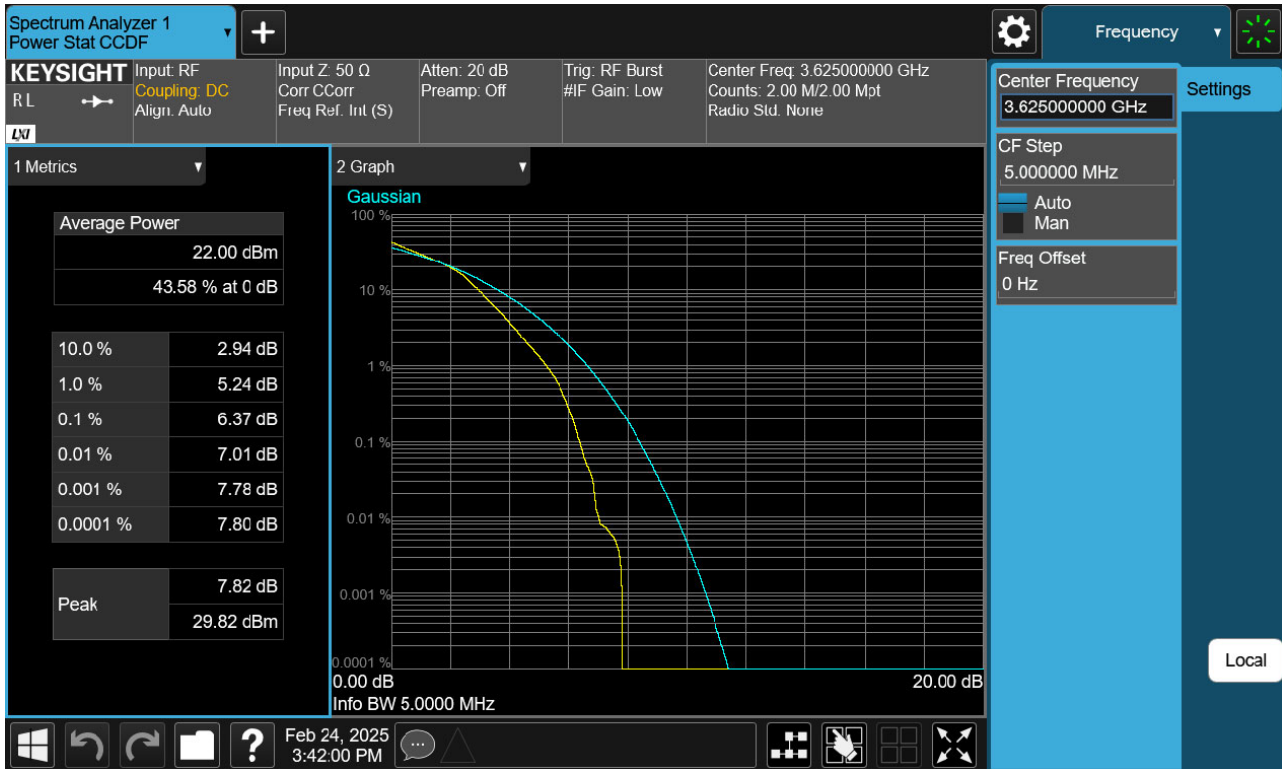
BAND 48. PAR Plot (5 M BW_Ch.55990_16QAM_RB25_0)
