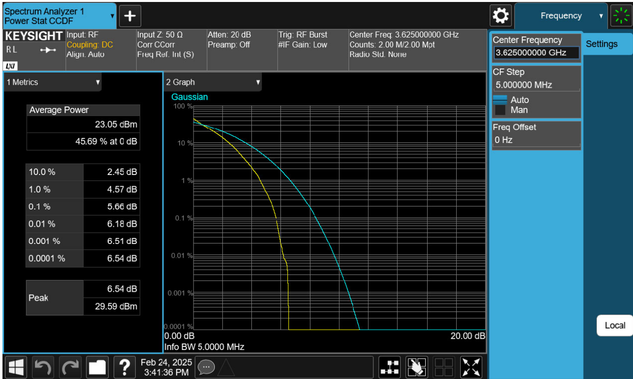
BAND 48. PAR Plot (5 M BW_Ch.55990_QPSK_RB25_0)
