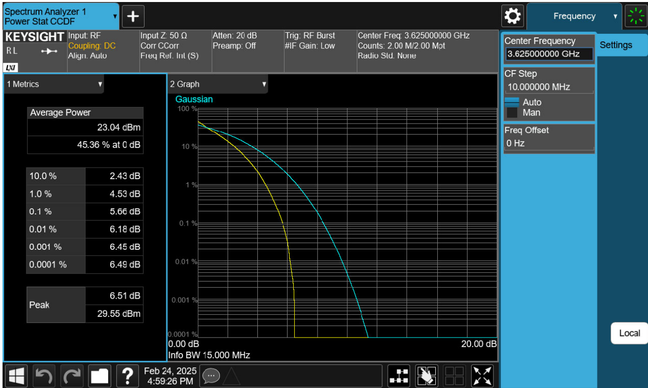
BAND 48. PAR Plot (15 M BW_Ch.55990_QPSK_RB75_0)
