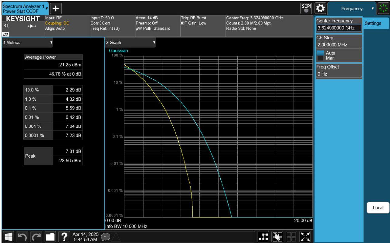
Sub6 n48. PAR Plot (10 MHz Ch. 641666 QPSK RB 24)
