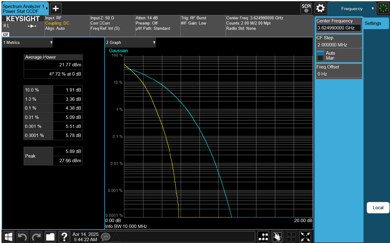
Sub6 n48. PAR Plot (10 MHz Ch. 641666 BPSK RB 24)
