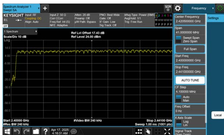
Dual ANT.2 \pi/4 DQPSK (2.4 GHz - 2.441 GHz)
