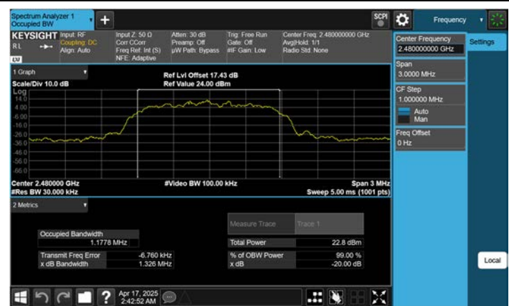
ANT. 2 \pi/4 DQPSK 20 dB BW & 99% OBW (Ch. 78)
