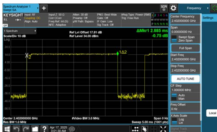
Dual ANT.1 \pi/4 DQPSK : Dwell Time(Ch. 0)
