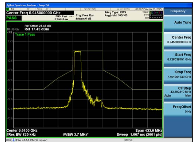
802.11be EHT80M Ch.199(6945 MHz) 996 Tones 67 RU
