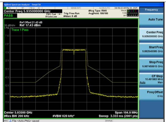
802.11be EHT20M Ch.2(5935 MHz) 242 Tones 61 RU
