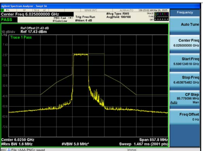
802.11be EHT160M Ch.Ch.15(6025 MHz) 996 Tones 67 RU
