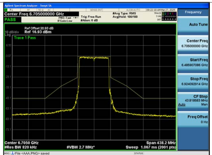
802.11be EHT80M Ch.151(6705 MHz) 996 Tones 67 RU
