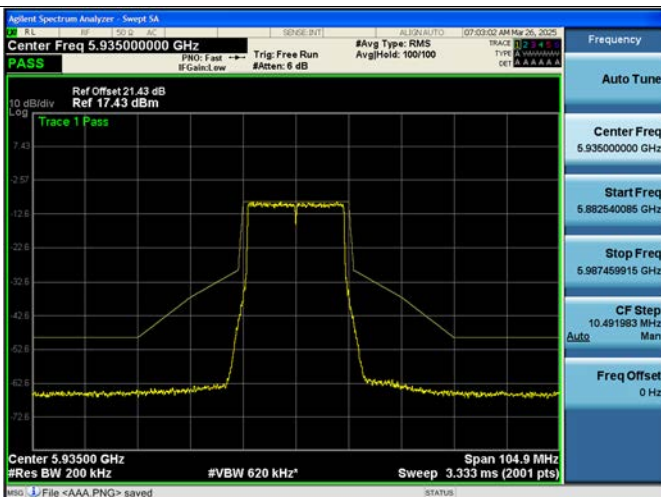
802.11be EHT20M Ch.2(5935 MHz) SU
