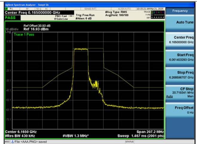
802.11be EHT40M Ch.43(6165 MHz) SU
