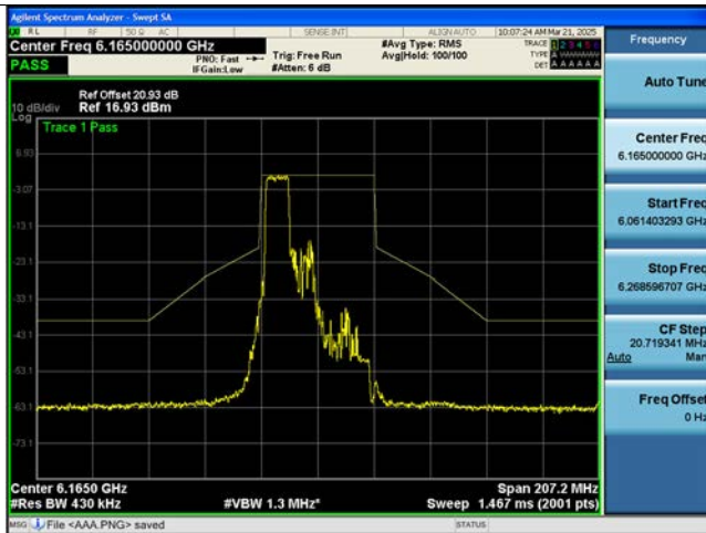
802.11be EHT40M Ch.43(6165 MHz) 484 Tones 65 RU
