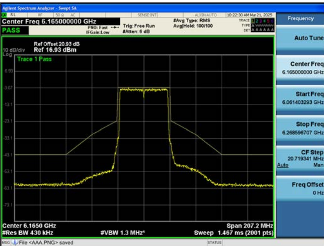
802.11be EHT40M Ch.43(6165 MHz) SU
