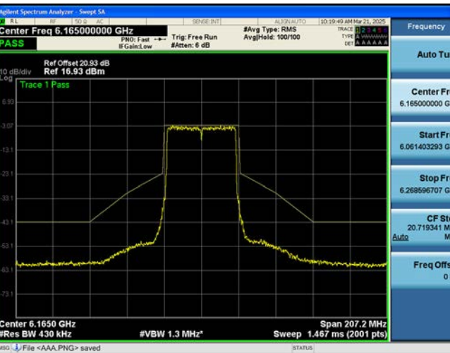
802.11be EHT40M Ch.43(6165 MHz) 484 Tones 65 RU
