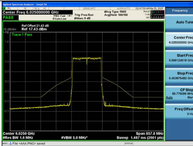
Bandwidth 160M, Ch. Ch.15(6025 MHz) SU
