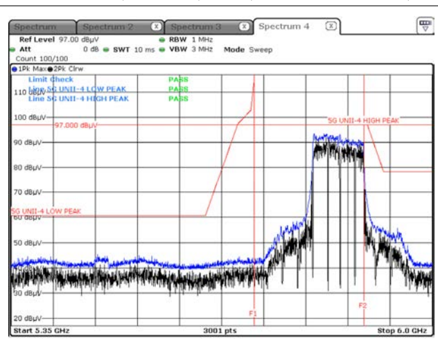
Peak result (802.11be(EHT80) Ch.171, 996T RU 67)
