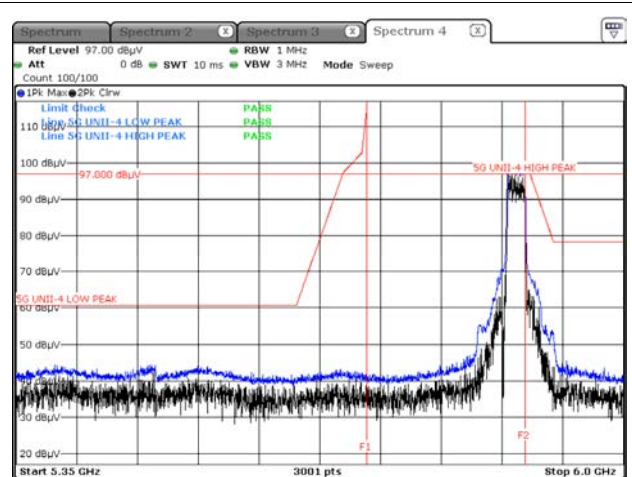
Peak result (802.11be(EHT20) Ch.177, 242T RU 61)
