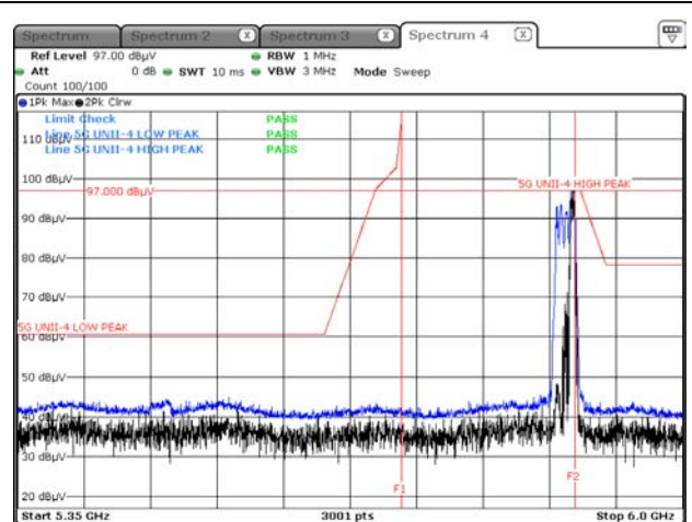
Peak result (802.11be(EHT20) Ch.177, 52T RU 40)
