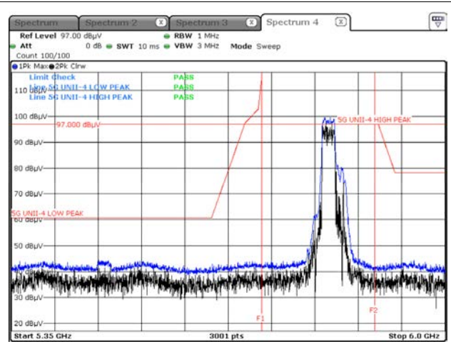
Peak result (802.11be(EHT40) Ch.167, 242T RU 61)
