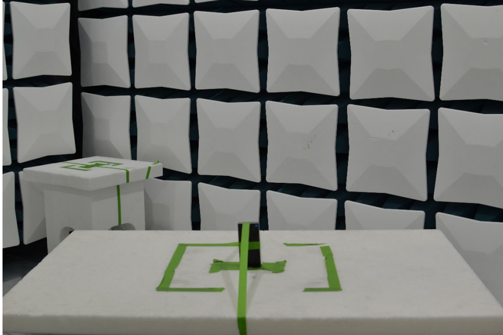
Figure 29. Test Setup – Y – WPT – 30MHz-18GHz
