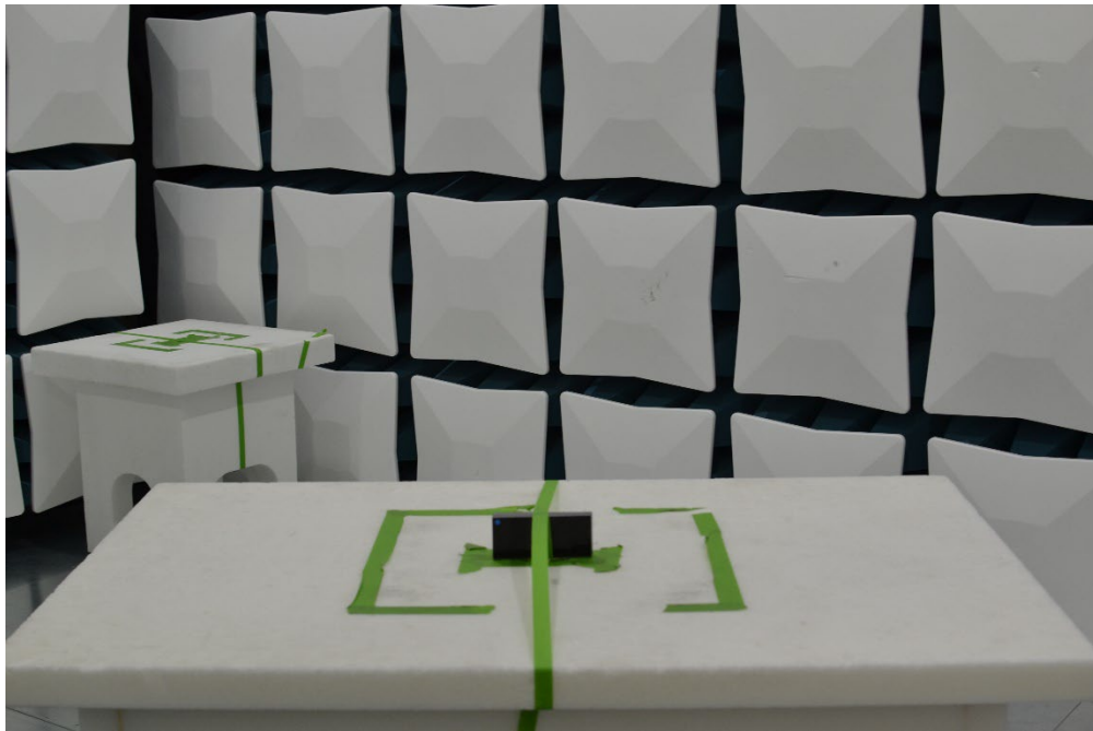
Figure 28. Test Setup – Y – WPT – 30MHz-18GHz
