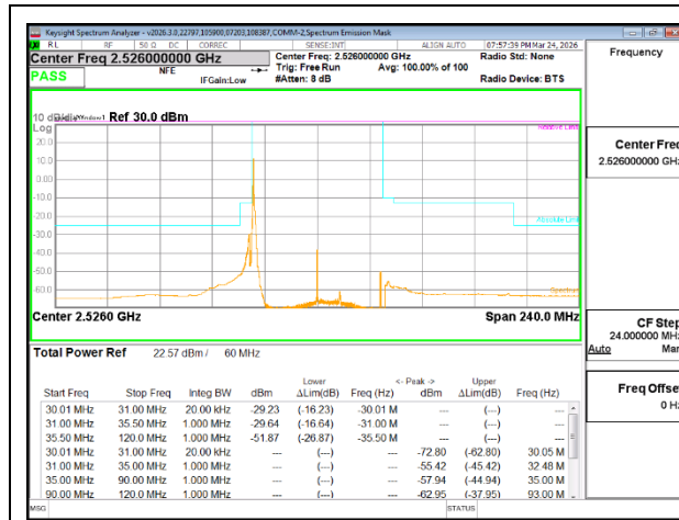
5G NR n41 60MHz BPSK Low Channel RB1-1
