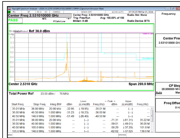
5G NR n41 70MHz BPSK Low Channel RB1-1
