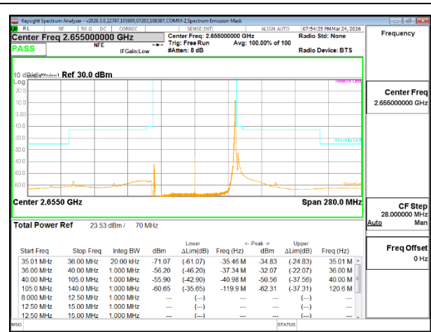
5G NR n41 70MHz BPSK High Channel RB1-187
