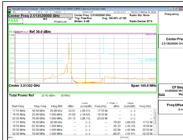
5G NR n41 35MHz BPSK Low Channel RB1-1
