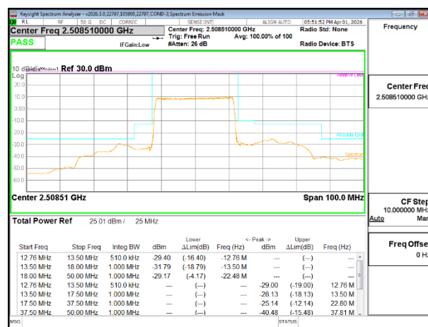
5G NR n41 25MHz BPSK Low Channel RB64-0
