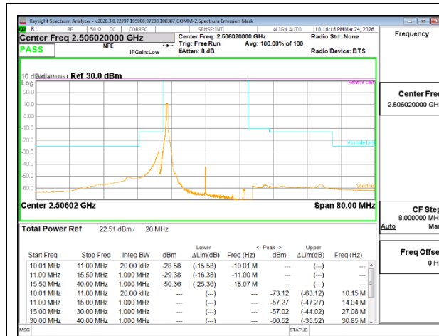
5G NR n41 20MHz BPSK Low Channel RB1-1
