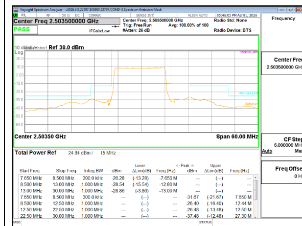
5G NR n41 15MHz BPSK Low Channel RB36-0
