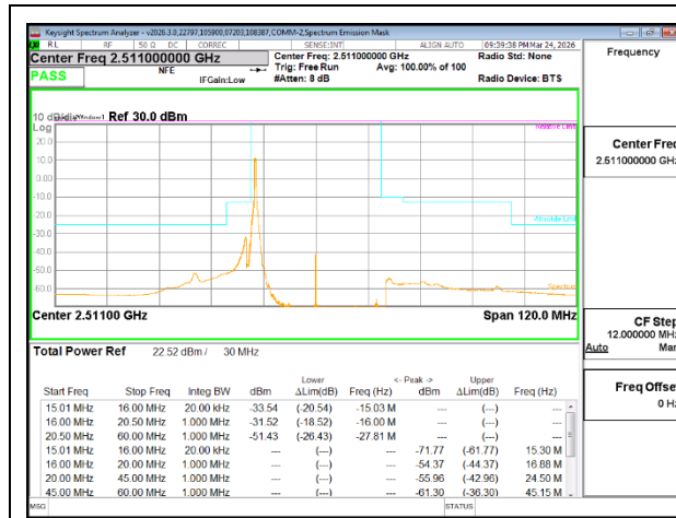
5G NR n41 30MHz BPSK Low Channel RB1-1
