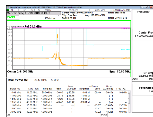
5G NR n7 20MHz BPSK Low Channel RB1-1
