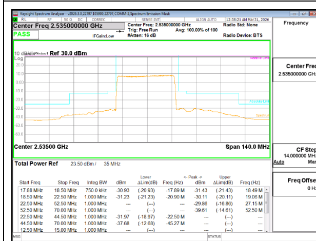
5G NR n7 35MHz BPSK Middle Channel RB180-0
