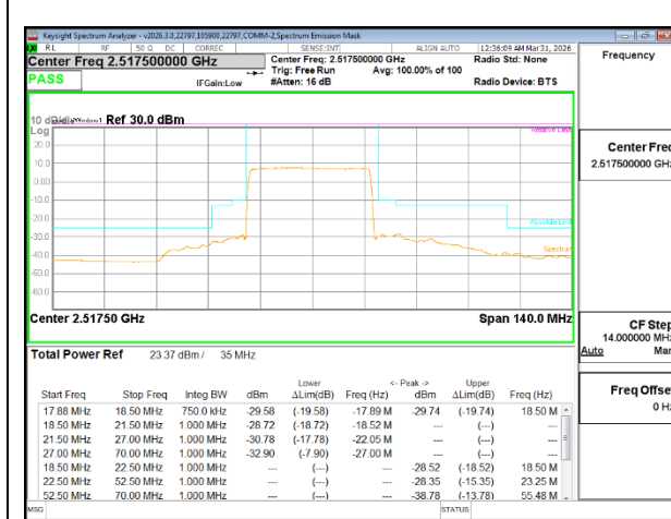
5G NR n7 35MHz BPSK Low Channel RB180-0
