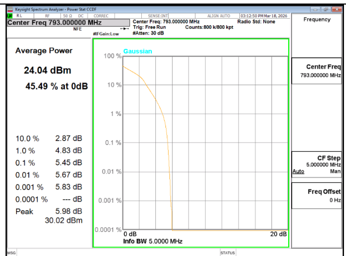
B14 5.0M 16QAM 25-0RB
