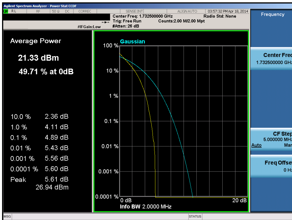
Plot 6-207. PAR Plot (Band 4 – 1.4MHz QPSK – RB Size 6)
