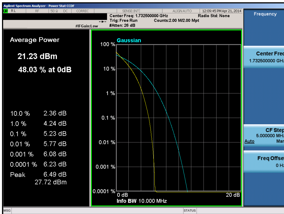
Plot 6-213. PAR Plot (Band 4 – 10.0MHz QPSK – RB Size 50)
