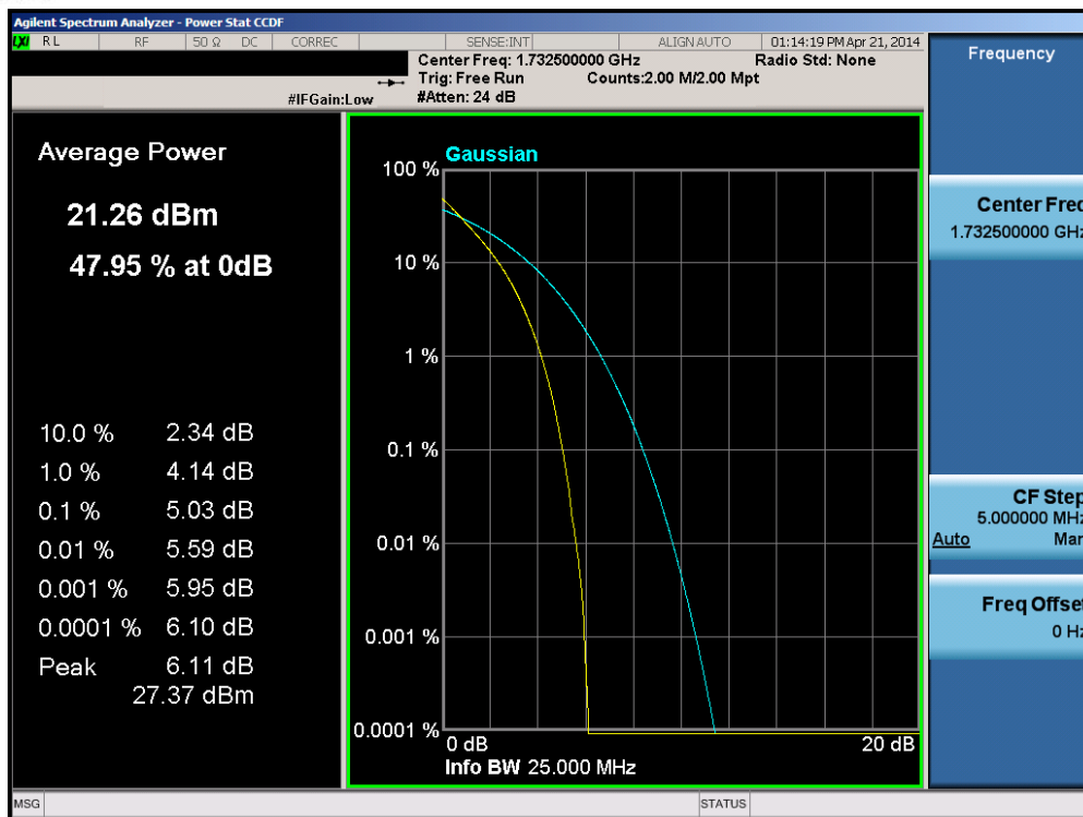
Plot 6-217. PAR Plot (Band 4 – 20.0MHz QPSK – RB Size 100)
