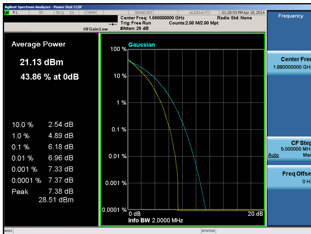
Plot 6-219. PAR Plot (Band 2 – 1.4MHz QPSK – RB Size 6)
