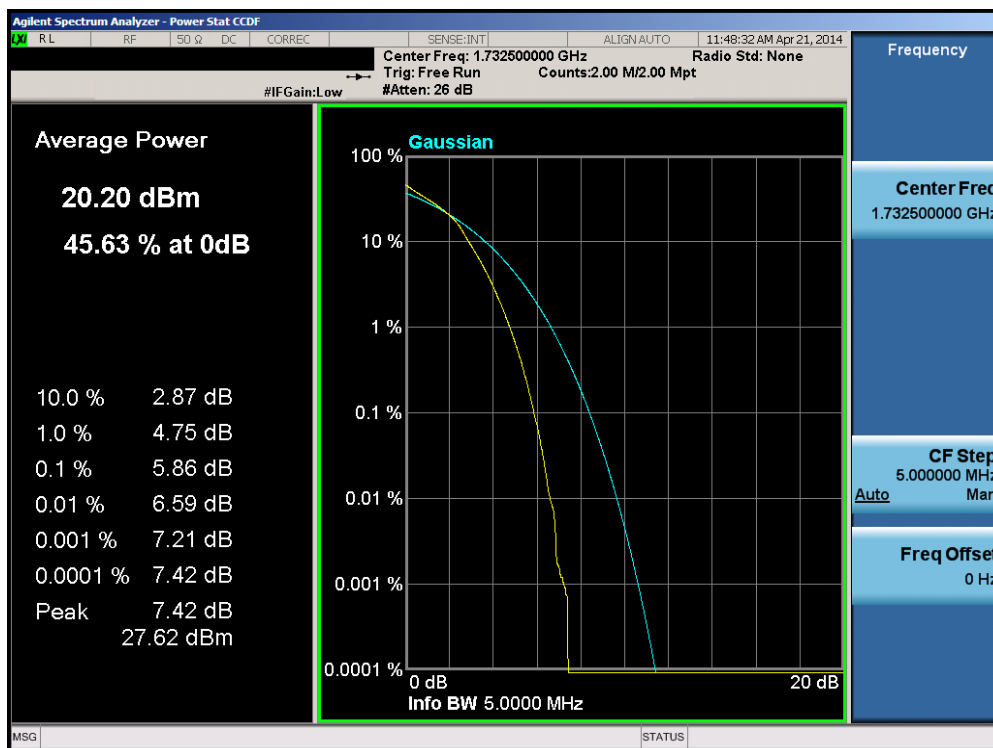
Plot 6-212. PAR Plot (Band 4 – 5.0MHz 16-QAM – RB Size 25)
