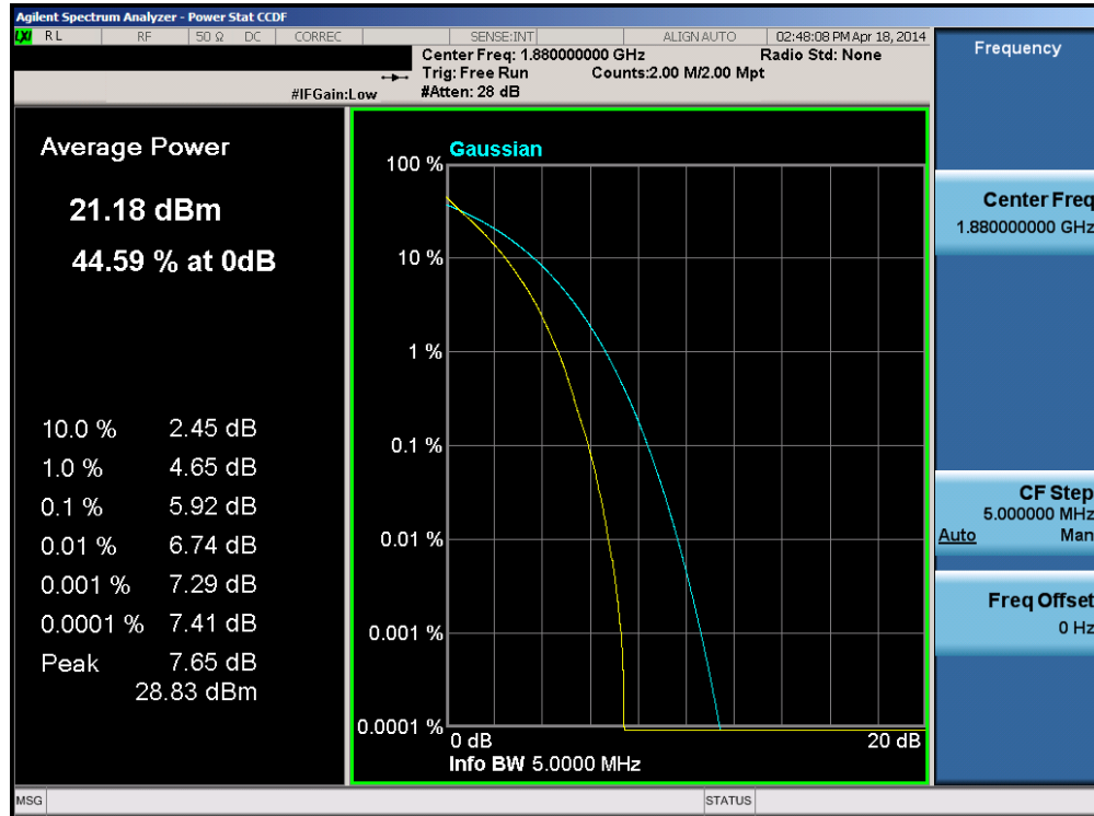
Plot 6-223. PAR Plot (Band 2 - 5.0MHz QPSK - RB Size 25)
