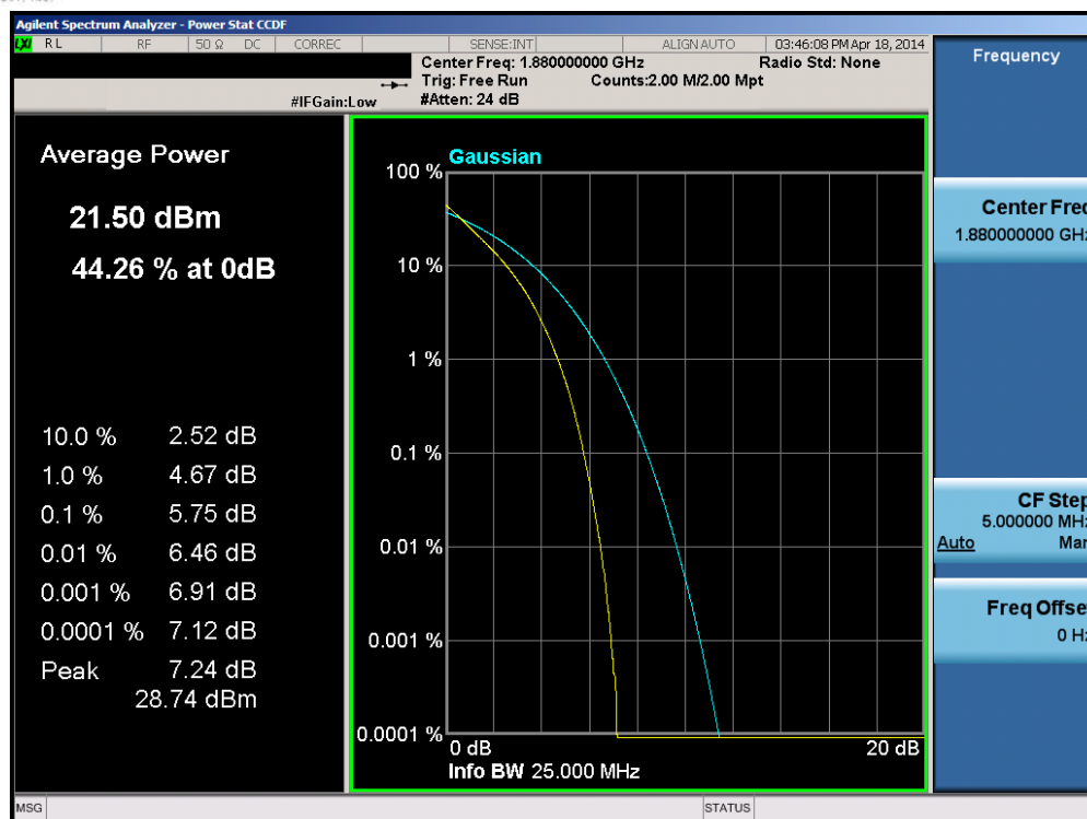
Plot 6-229. PAR Plot (Band 2 – 20.0MHz QPSK – RB Size 100)
