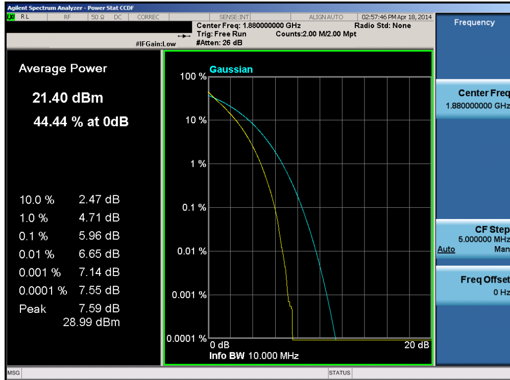
Plot 6-225. PAR Plot (Band 2 – 10.0MHz QPSK – RB Size 50)
