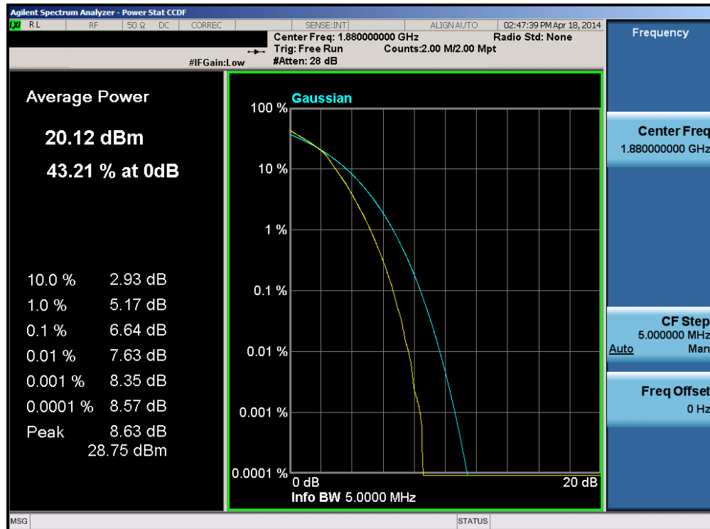
Plot 6-224. PAR Plot (Band 2 - 5.0MHz 16-QAM - RB Size 25)
