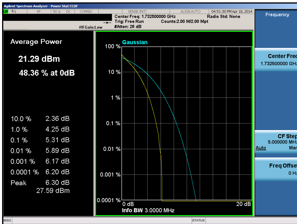
Plot 6-209. PAR Plot (Band 4 – 3.0MHz QPSK – RB Size 15)
