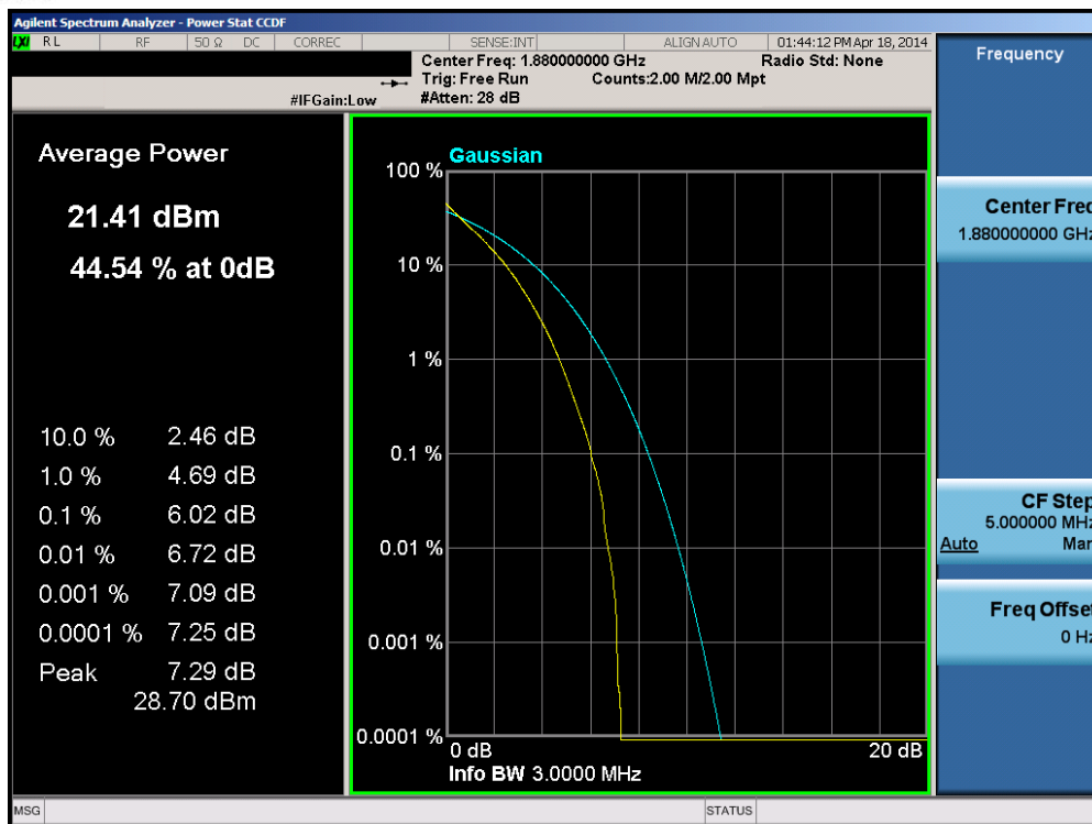
Plot 6-221. PAR Plot (Band 2 – 3.0MHz QPSK – RB Size 15)
