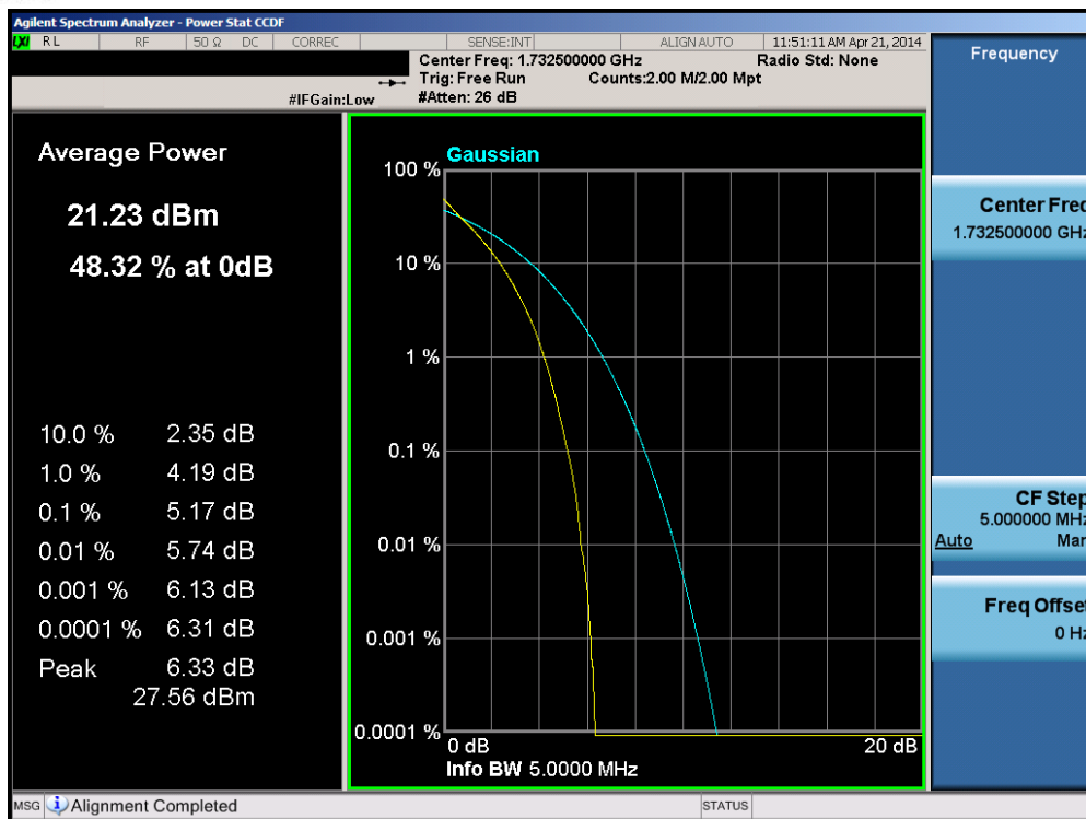
Plot 6-211. PAR Plot (Band 4 – 5.0MHz QPSK – RB Size 25)
