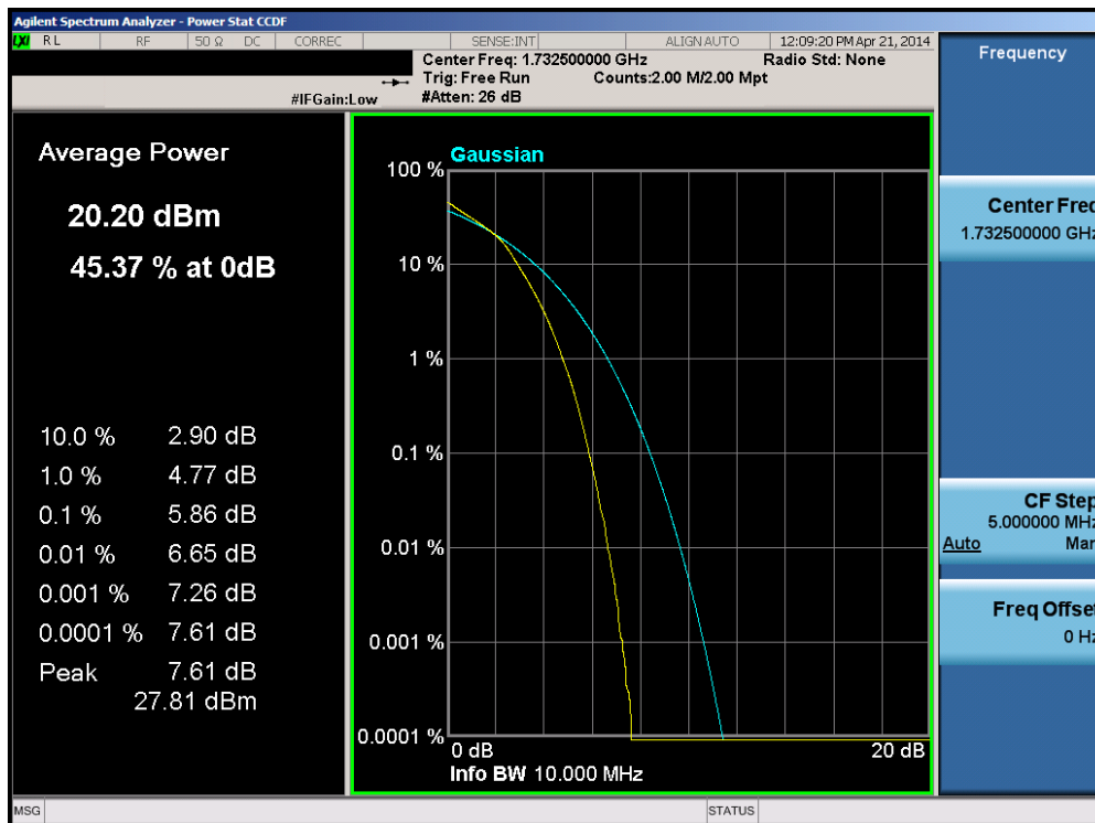
Plot 6-214. PAR Plot (Band 4 – 10.0MHz 16-QAM – RB Size 50)
