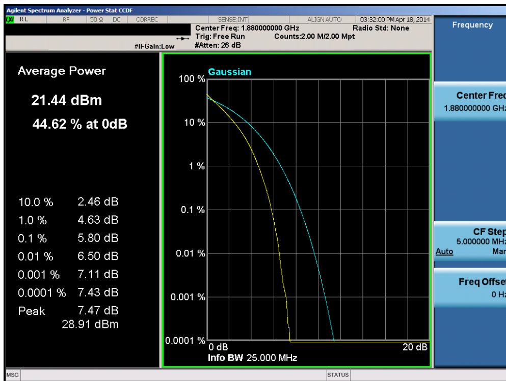
Plot 6-227. PAR Plot (Band 2 – 15.0MHz QPSK – RB Size 75)
