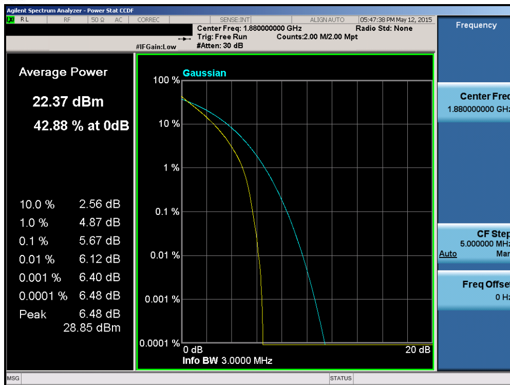
Plot 6-184. PAR Plot (Band 2/25 – 3.0MHz QPSK – RB Size 15)
