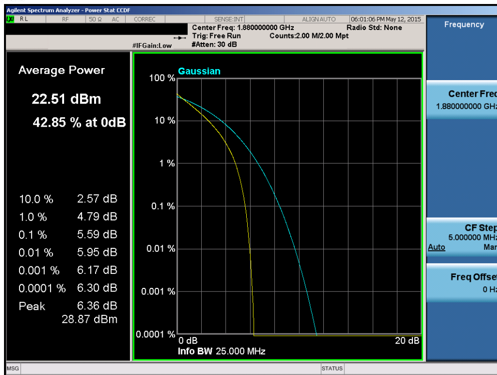
Plot 6-190. PAR Plot (Band 2/25 – 15.0MHz QPSK – RB Size 75)
