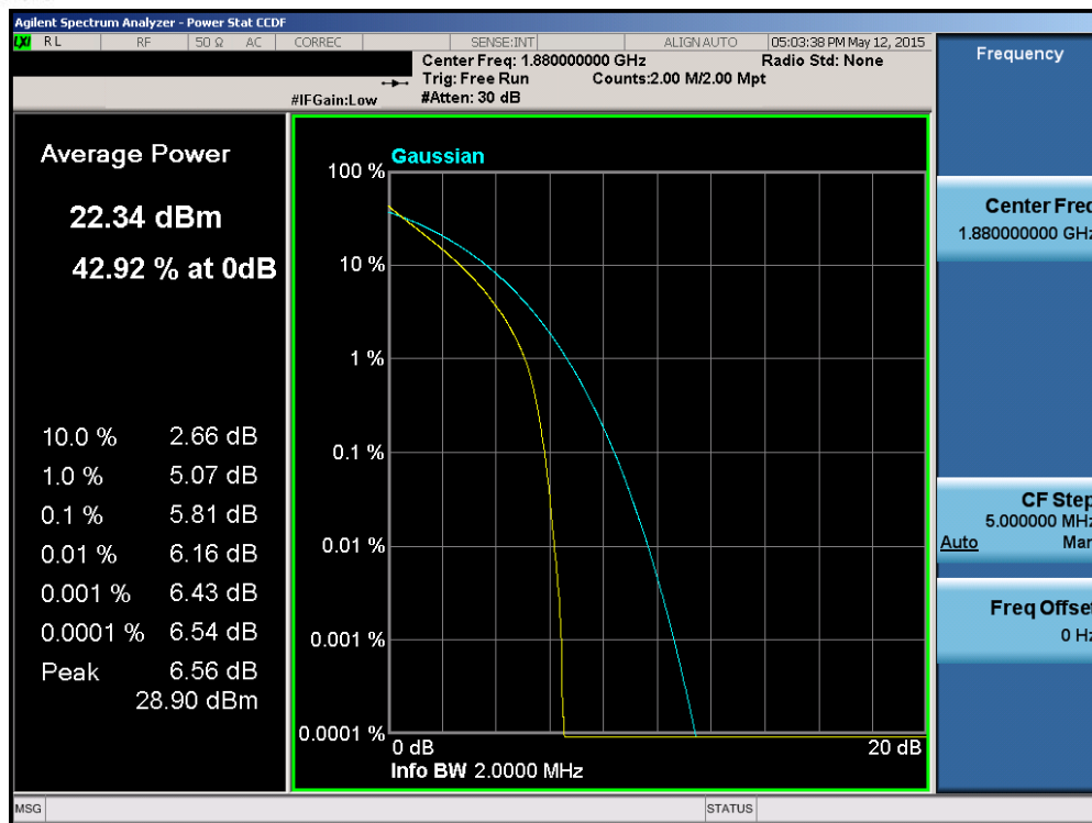
Plot 6-182. PAR Plot (Band 2/25 – 1.4MHz QPSK – RB Size 6)
