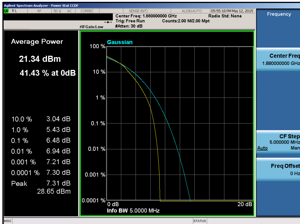
Plot 6-187. PAR Plot (Band 2/25 – 5.0MHz 16-QAM – RB Size 25)
