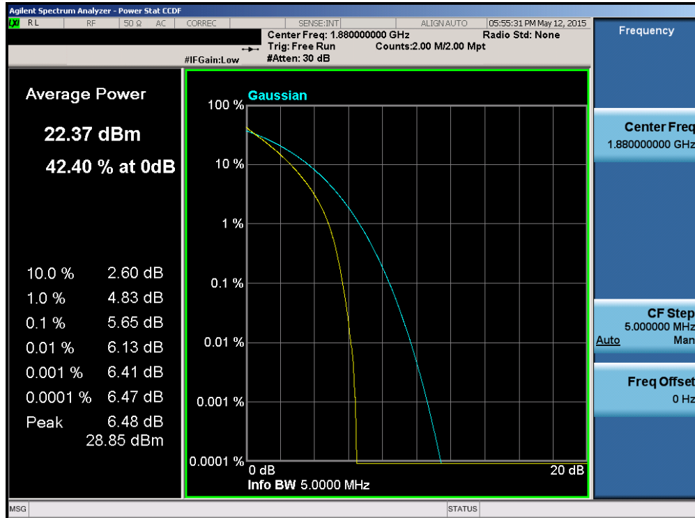
Plot 6-186. PAR Plot (Band 2/25 – 5.0MHz QPSK – RB Size 25)
