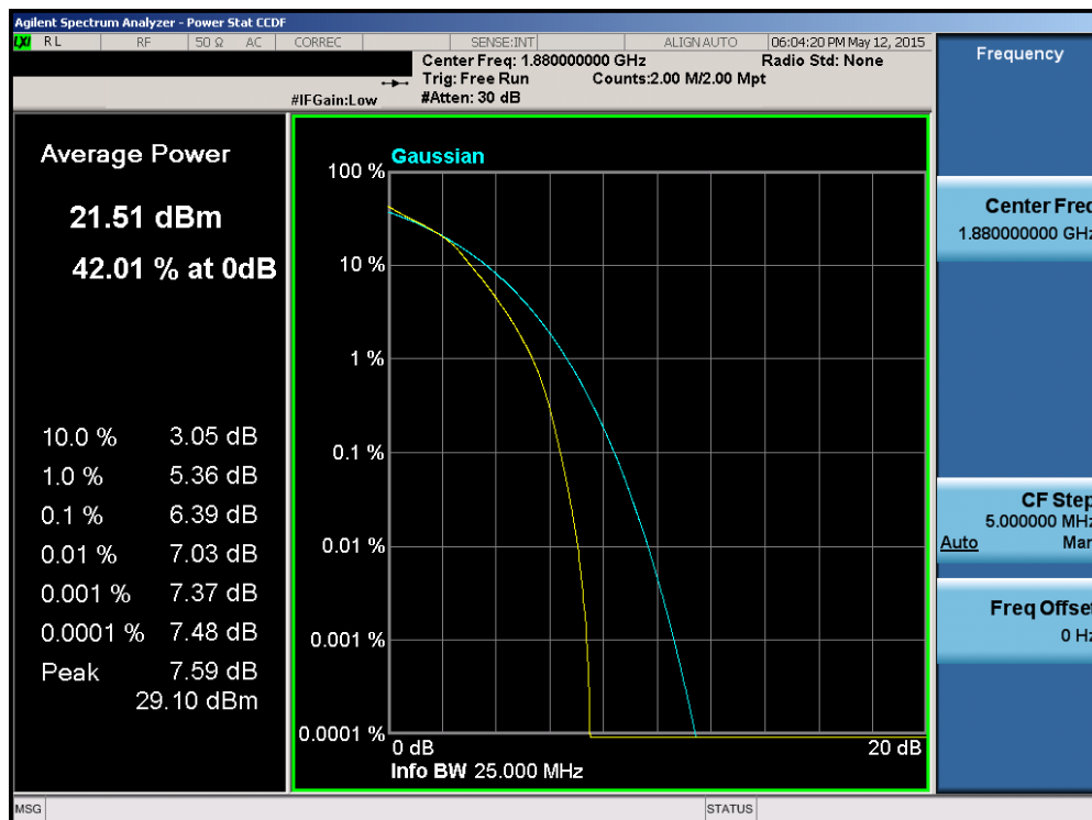
Plot 6-193. PAR Plot (Band 2/25 – 20.0MHz 16-QAM – RB Size 100)
