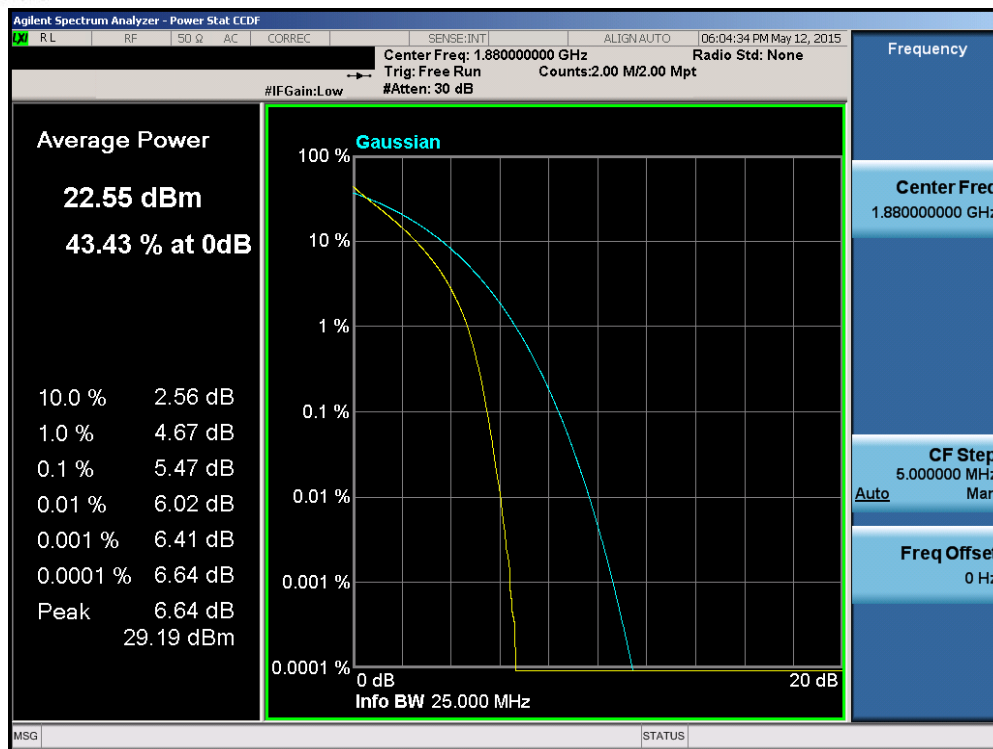
Plot 6-192. PAR Plot (Band 2/25 – 20.0MHz QPSK – RB Size 100)
