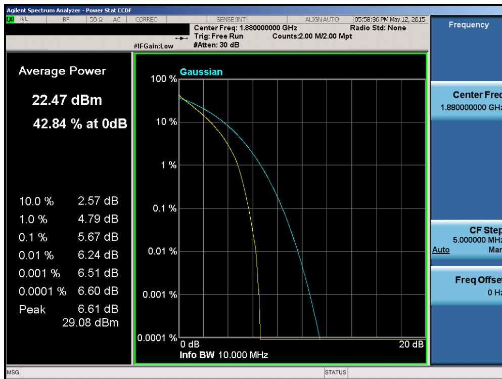
Plot 6-188. PAR Plot (Band 2/25 – 10.0MHz QPSK – RB Size 50)
