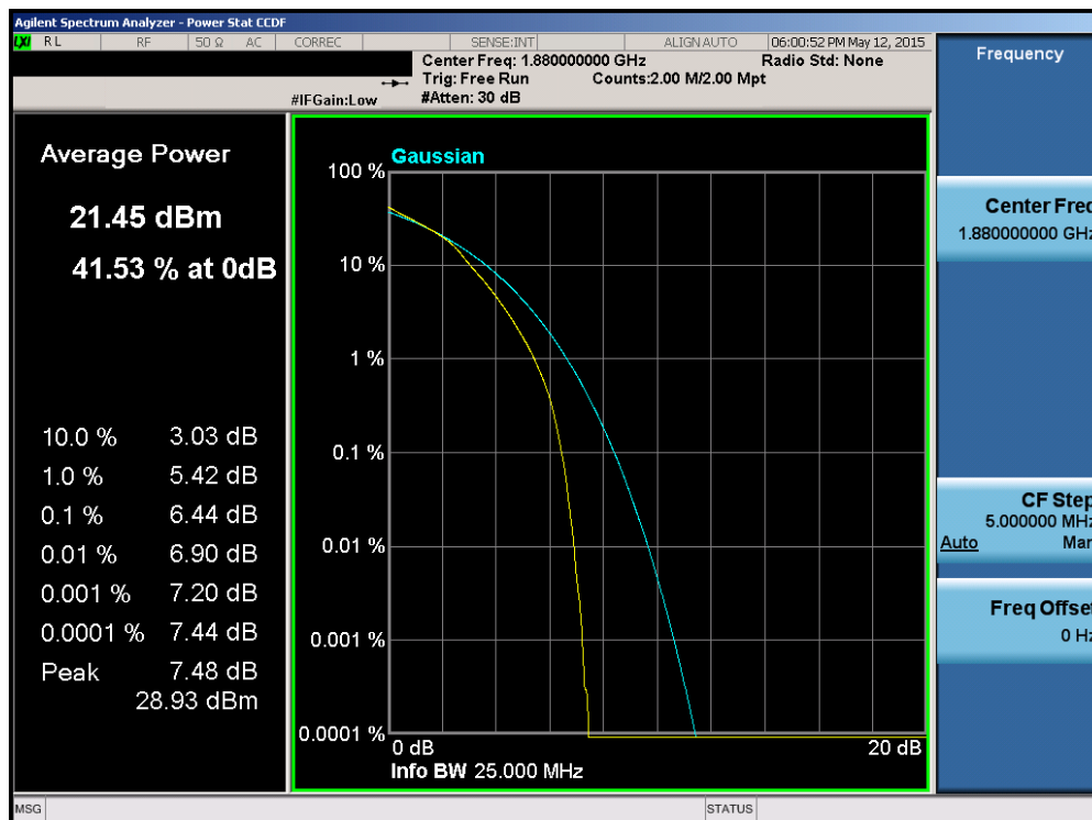
Plot 6-191. PAR Plot (Band 2/25 – 15.0MHz 16-QAM – RB Size 75)
