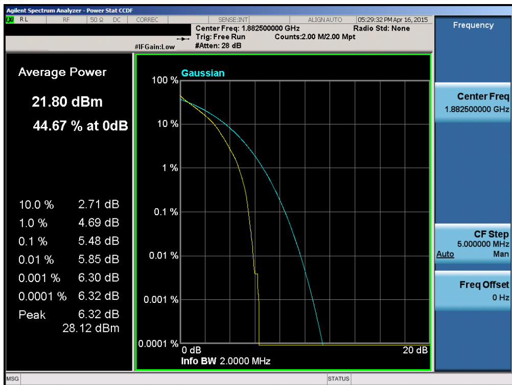
Plot 6-153. PAR Plot (Band 25 – 1.4MHz QPSK – RB Size 6)
