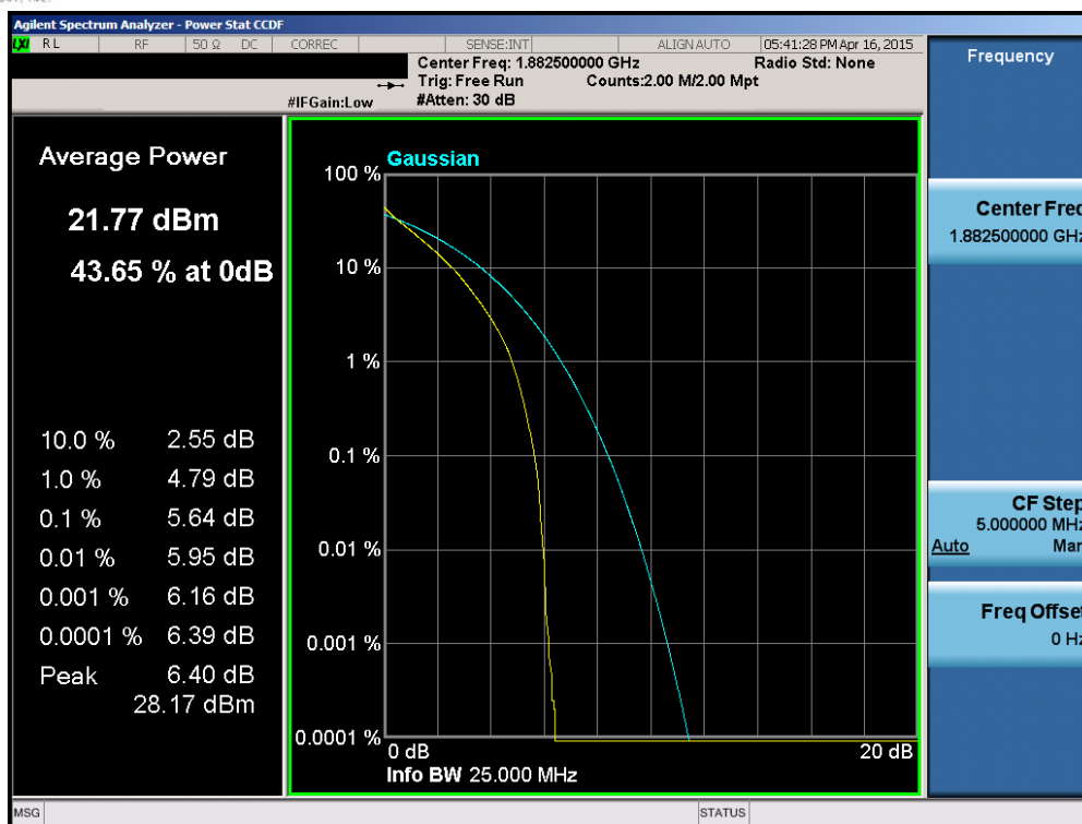
Plot 6-161. PAR Plot (Band 25 – 15.0MHz QPSK – RB Size 75)
