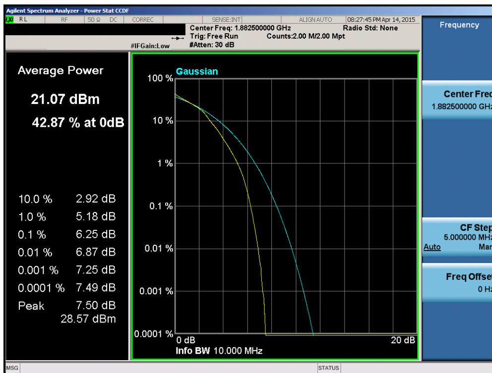
Plot 6-160. PAR Plot (Band 25 – 10.0MHz 16-QAM – RB Size 50)
