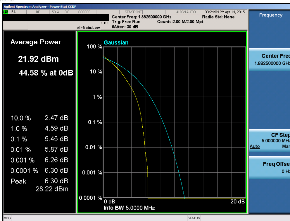
Plot 6-157. PAR Plot (Band 25 – 5.0MHz QPSK – RB Size 25)
