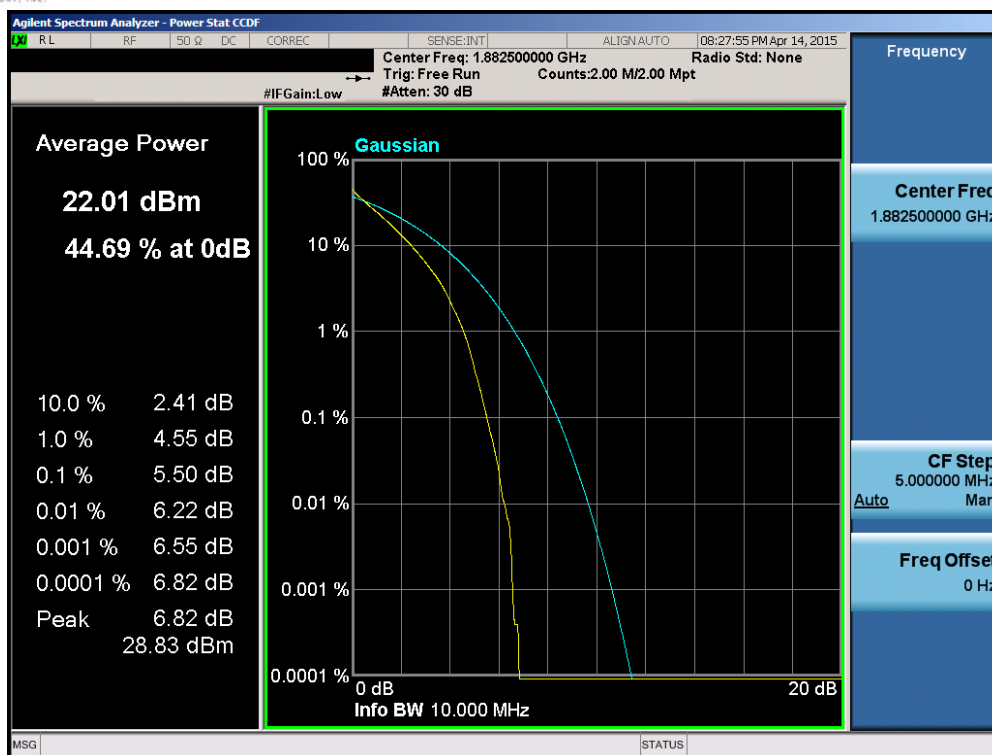
Plot 6-159. PAR Plot (Band 25 – 10.0MHz QPSK – RB Size 50)
