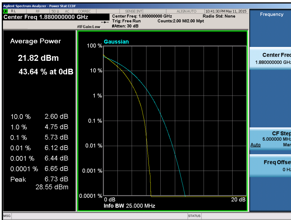
Plot 6-147. PAR Plot (Band 2 – 15.0MHz QPSK – RB Size 75)
