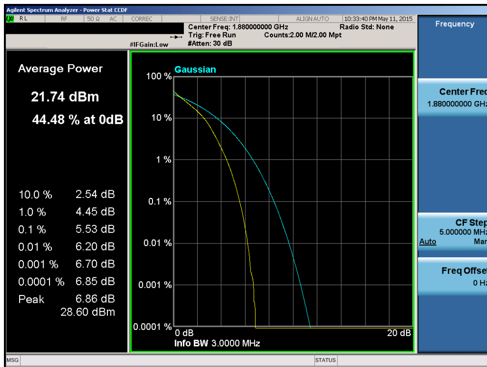
Plot 6-141. PAR Plot (Band 2 – 3.0MHz QPSK – RB Size 15)
