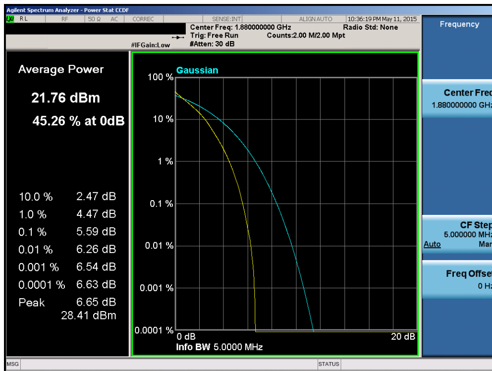
Plot 6-143. PAR Plot (Band 2 – 5.0MHz QPSK – RB Size 25)
