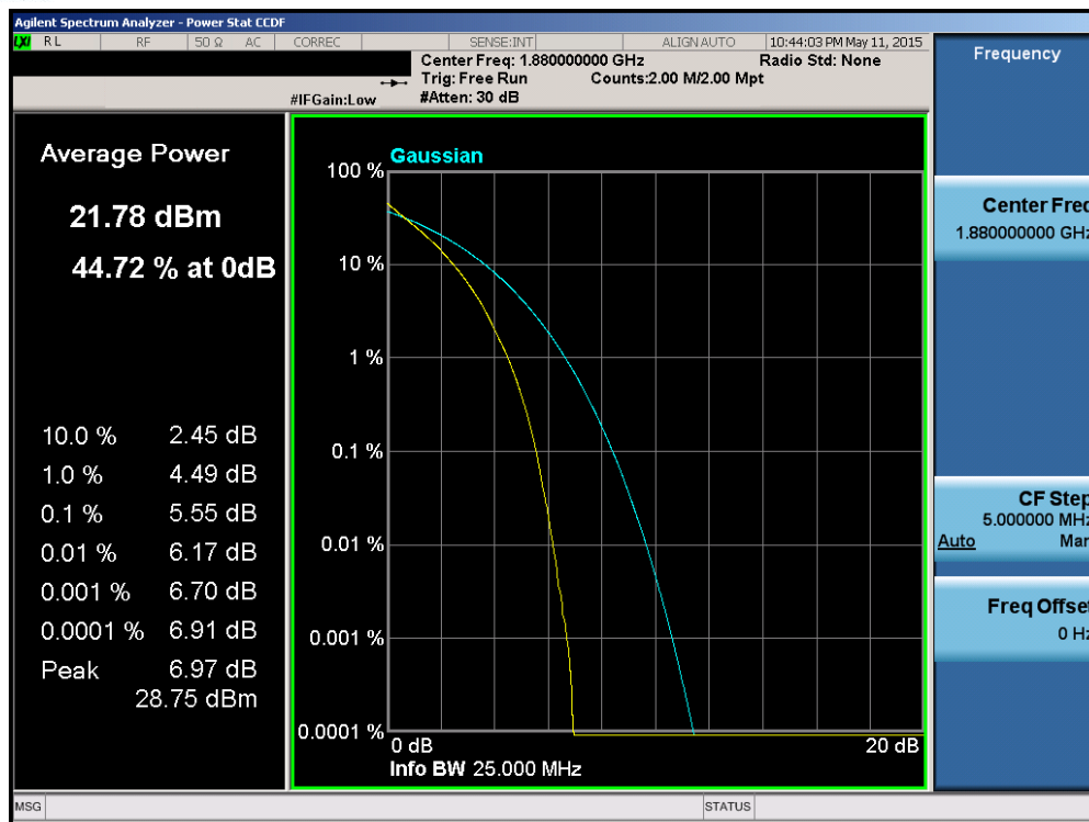
Plot 6-149. PAR Plot (Band 2 – 20.0MHz QPSK – RB Size 100)
