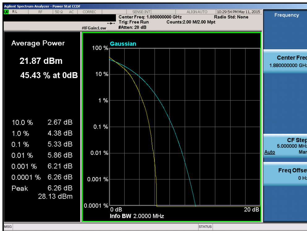
Plot 6-139. PAR Plot (Band 2 – 1.4MHz QPSK – RB Size 6)
