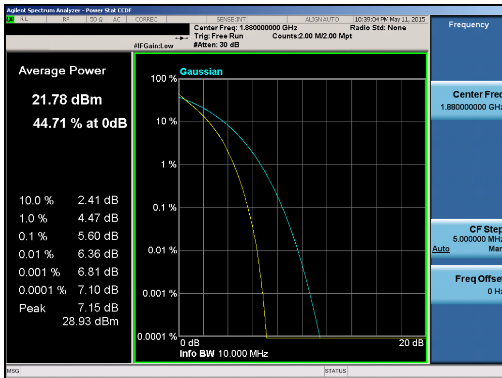
Plot 6-145. PAR Plot (Band 2 – 10.0MHz QPSK – RB Size 50)
