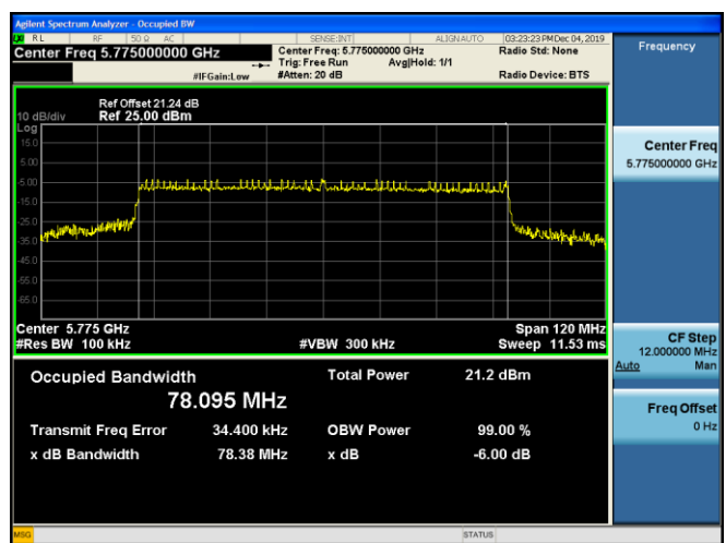
802.11ac(VHT80) (CH.155)
