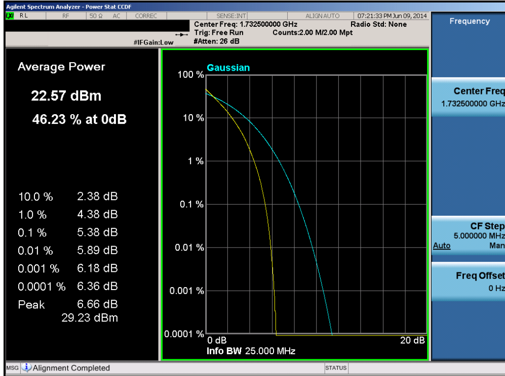
Plot 6-223. PAR Plot (Band 4 – 20.0MHz QPSK – RB Size 100)
