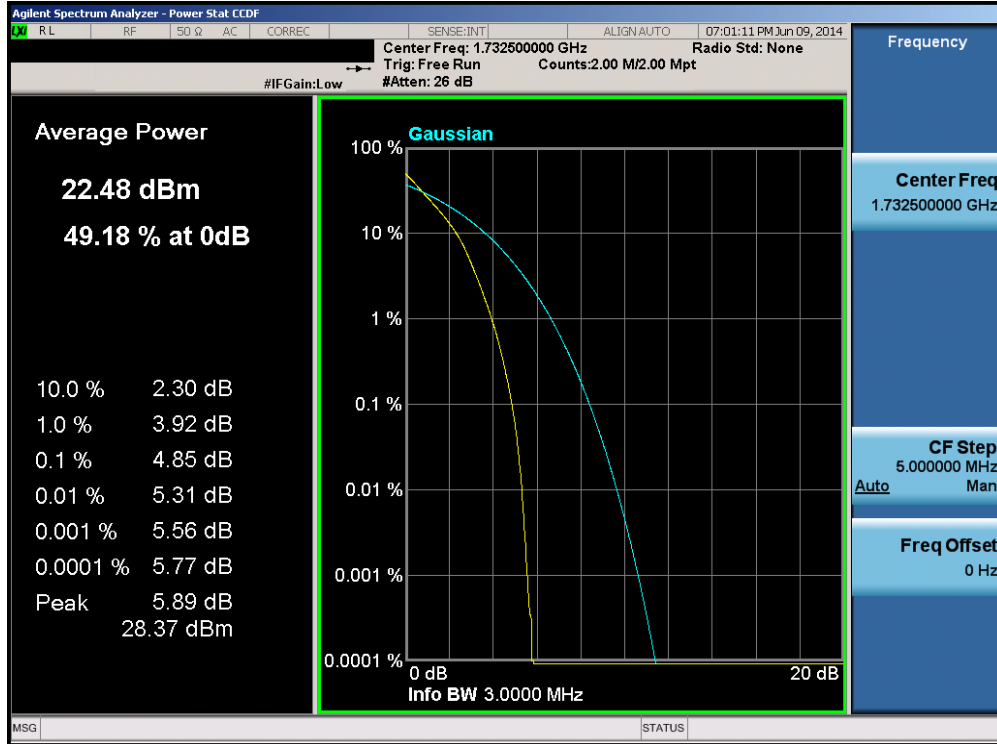
Plot 6-215. PAR Plot (Band 4 – 3.0MHz QPSK – RB Size 15)
