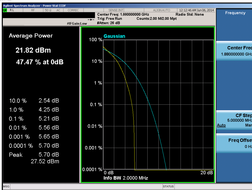
Plot 6-225. PAR Plot (Band 2 – 1.4MHz QPSK – RB Size 6)
