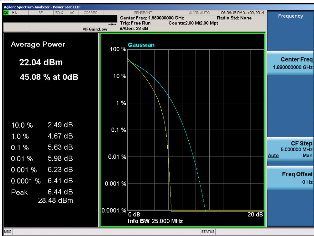
Plot 6-233. PAR Plot (Band 2 – 15.0MHz QPSK – RB Size 75)
