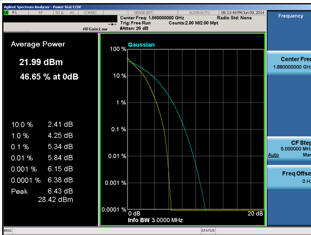
Plot 6-227. PAR Plot (Band 2 – 3.0MHz QPSK – RB Size 15)
