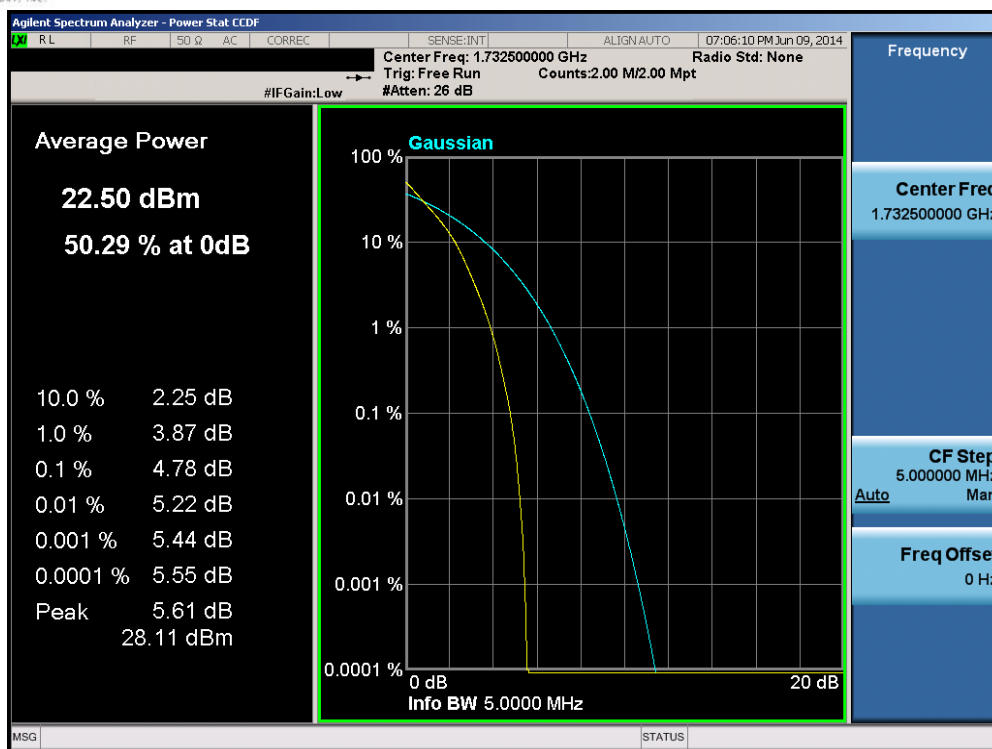
Plot 6-217. PAR Plot (Band 4 – 5.0MHz QPSK – RB Size 25)
