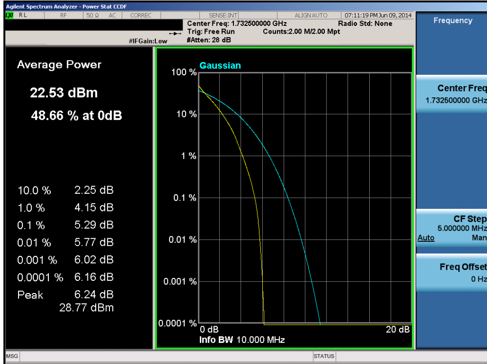
Plot 6-219. PAR Plot (Band 4 – 10.0MHz QPSK – RB Size 50)
