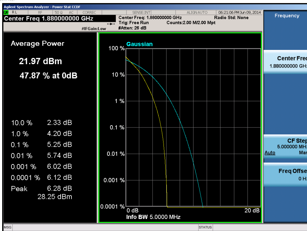
Plot 6-229. PAR Plot (Band 2 – 5.0MHz QPSK – RB Size 25)
