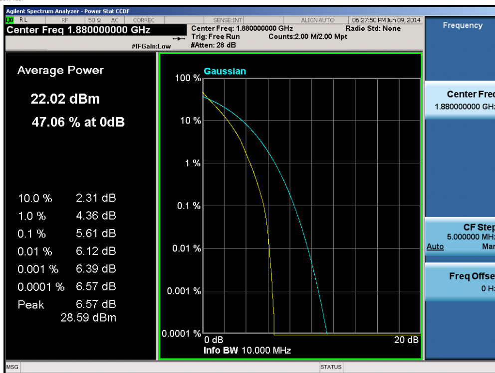
Plot 6-231. PAR Plot (Band 2 – 10.0MHz QPSK – RB Size 50)
