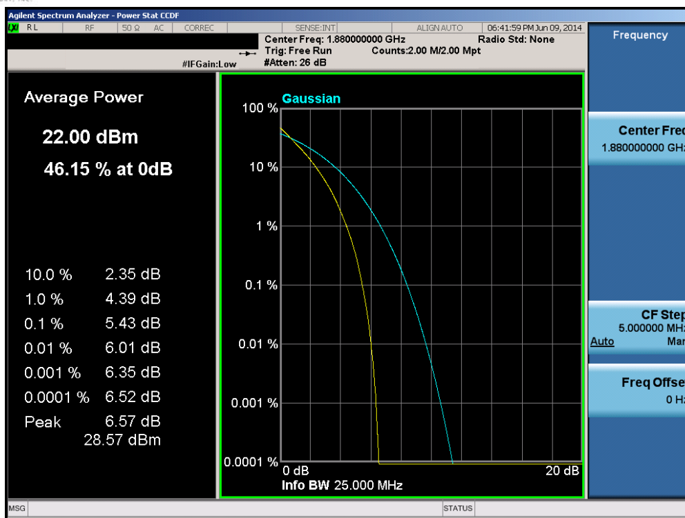
Plot 6-235. PAR Plot (Band 2 – 20.0MHz QPSK – RB Size 100)
