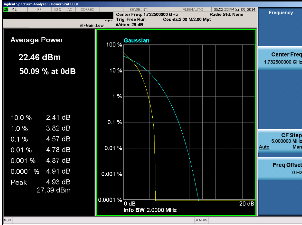
Plot 6-213. PAR Plot (Band 4 – 1.4MHz QPSK – RB Size 6)
