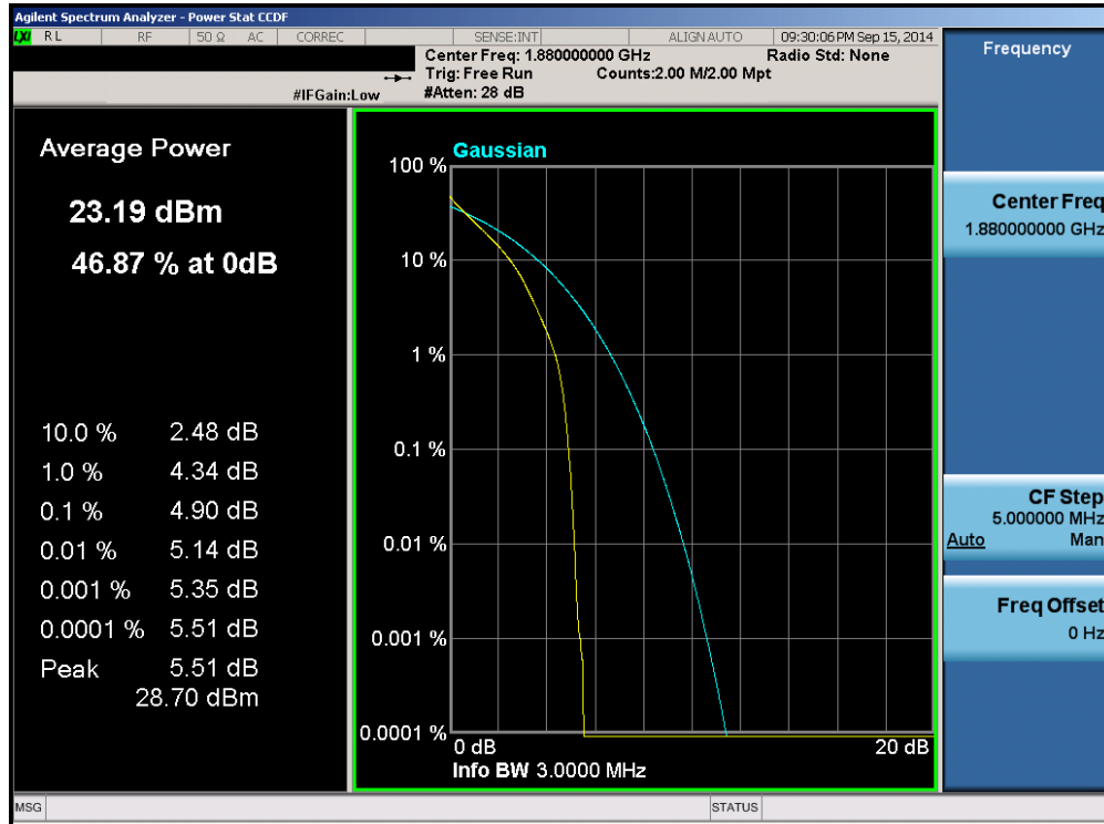
Plot 6-73. PAR Plot (Band 2 – 3.0MHz QPSK – RB Size 15)
