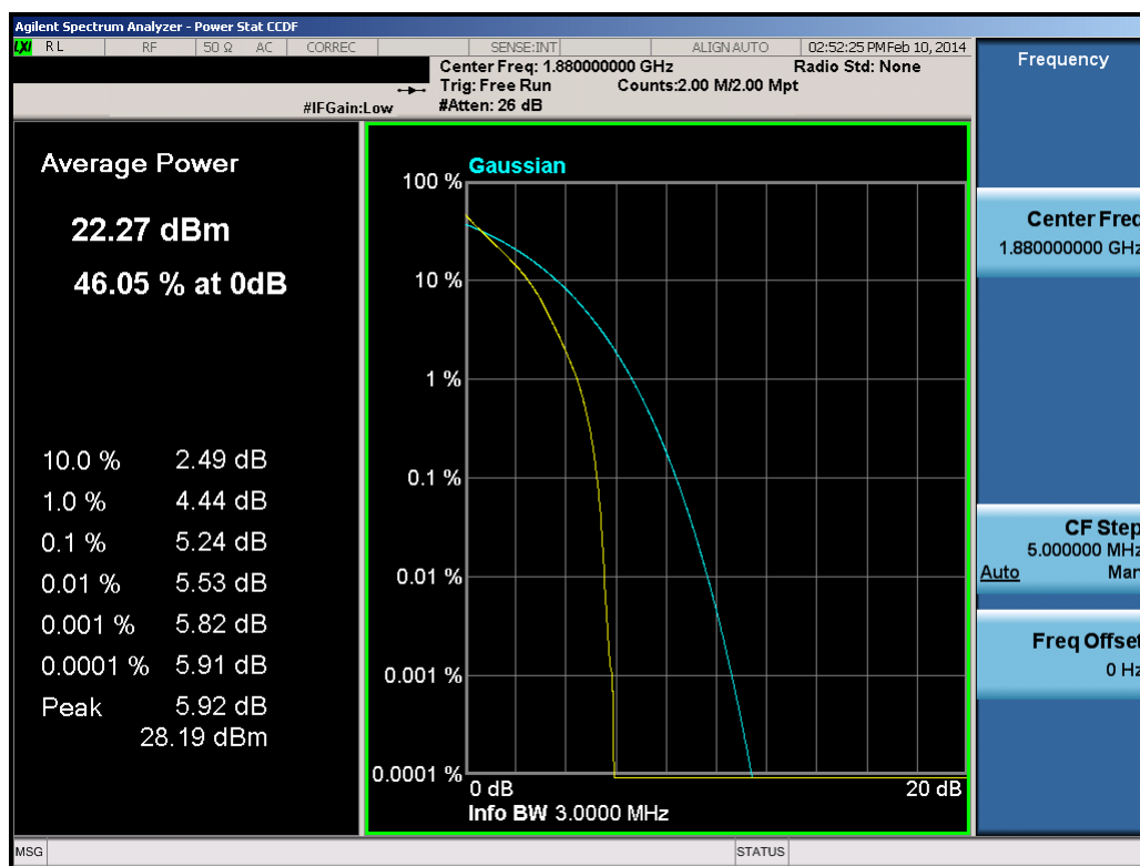
Plot 8-27. PAR Plot (3.0MHz QPSK – RB Size 15)
