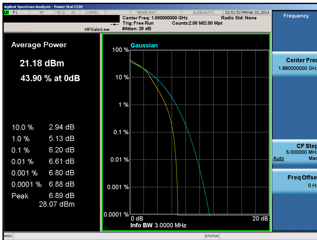
Plot 8-28. PAR Plot (3.0MHz 16-QAM - RB Size 15)
