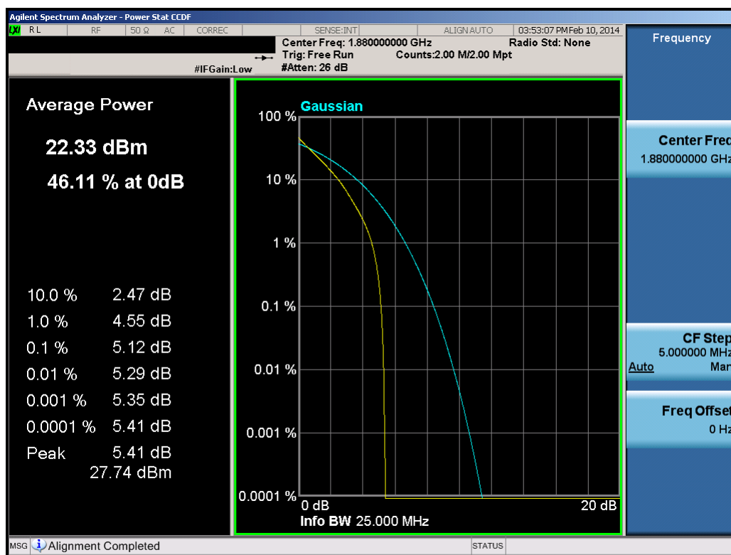
Plot 8-69. PAR Plot (15.0MHz QPSK – RB Size 75)
