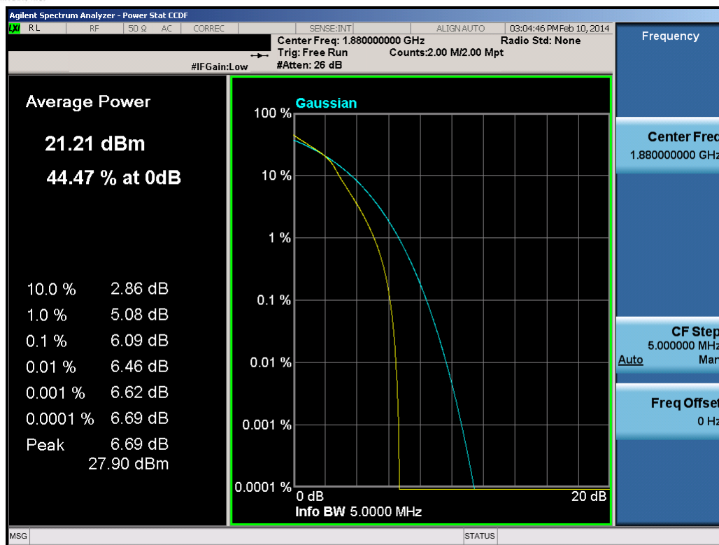
Plot 8-42. PAR Plot (5.0MHz 16-QAM - RB Size 25)
