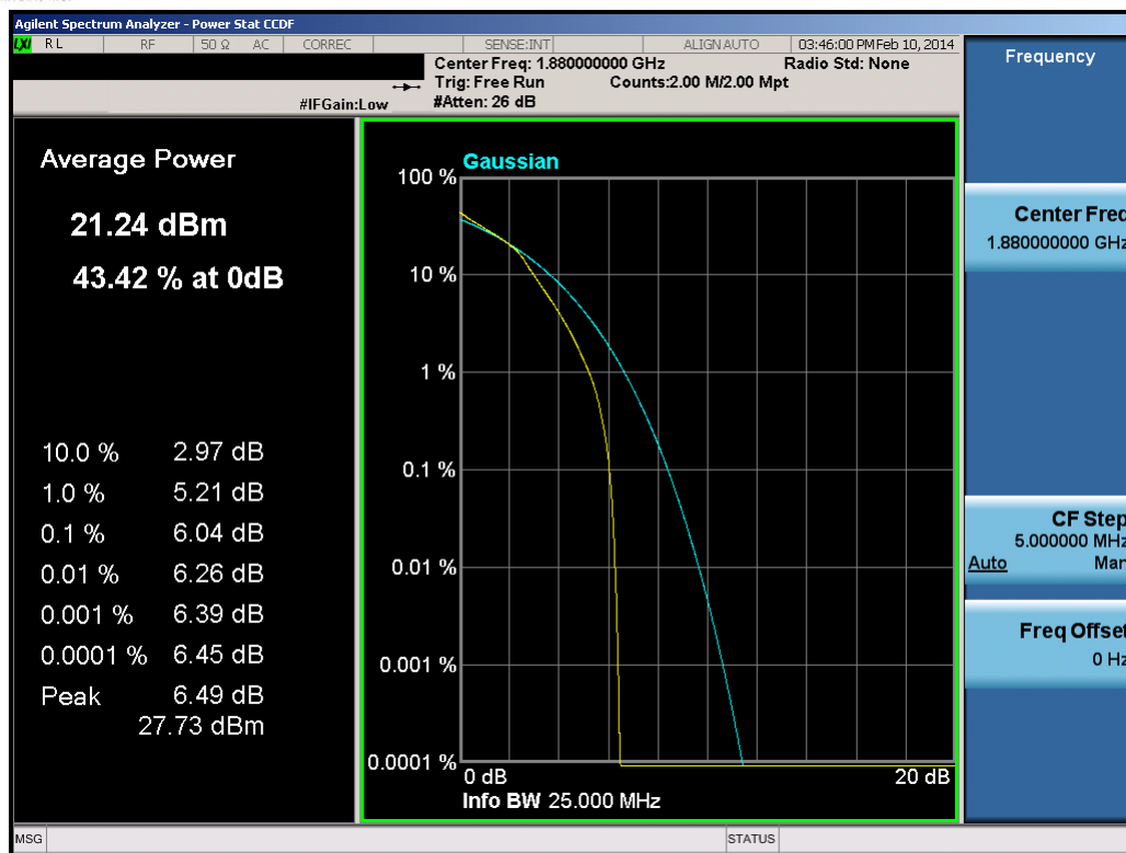
Plot 8-70. PAR Plot (15.0MHz 16-QAM – RB Size 75)
