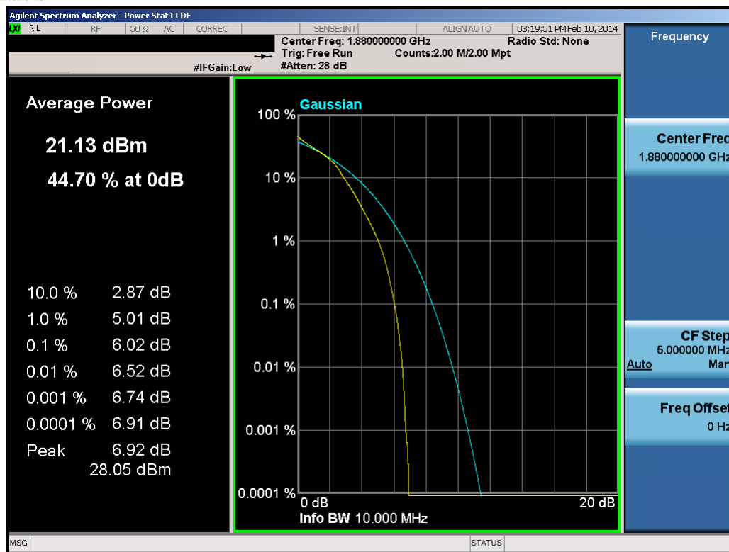
Plot 8-56. PAR Plot (10.0MHz 16-QAM – RB Size 50)
