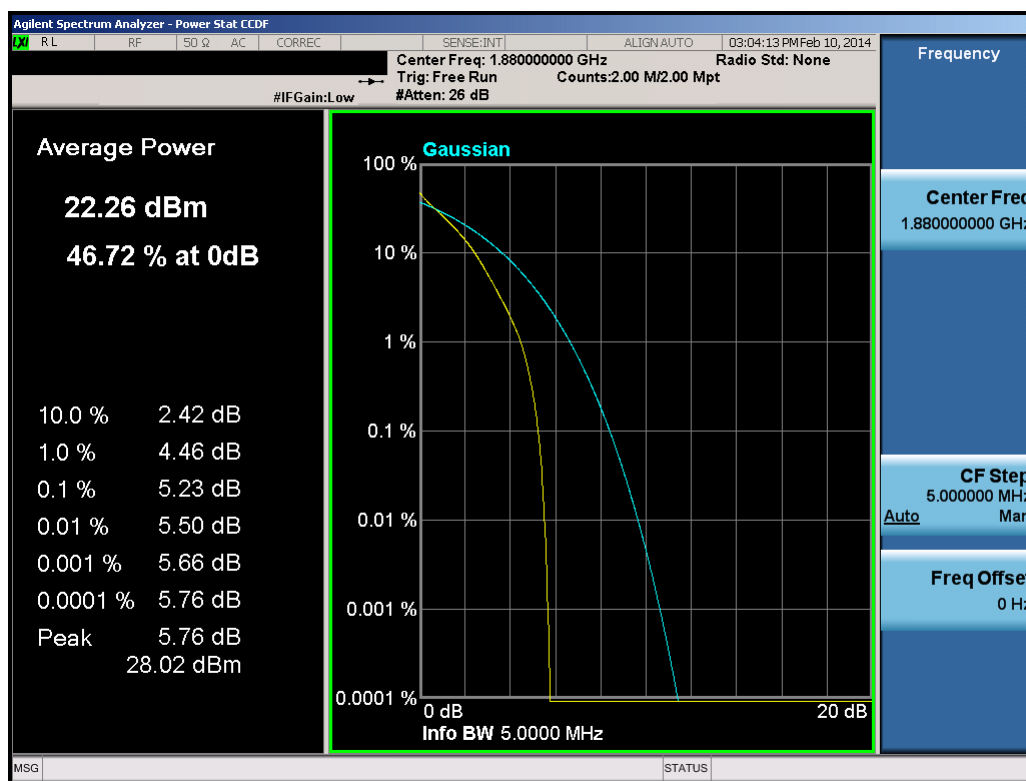
Plot 8-41. PAR Plot (5.0MHz QPSK – RB Size 25)
