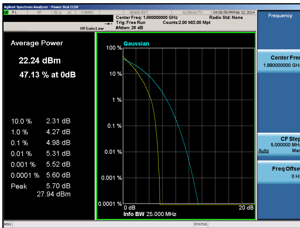
Plot 8-83. PAR Plot (20.0MHz QPSK – RB Size 100)
