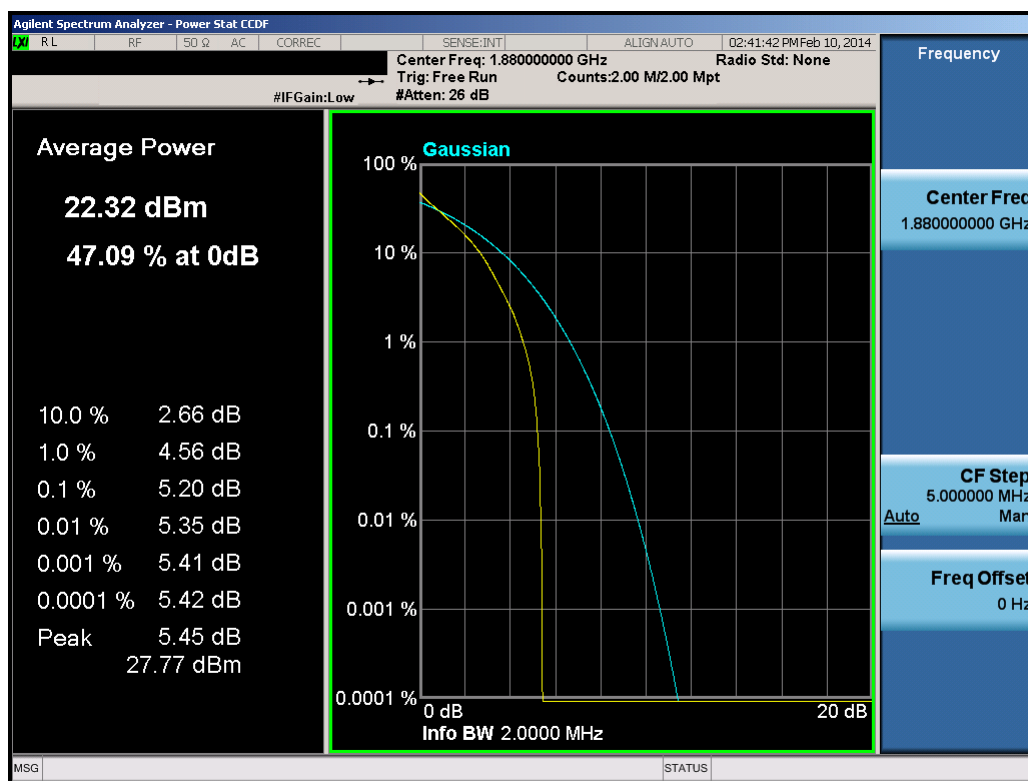
Plot 8-13. PAR Plot (1.4MHz QPSK – RB Size 6)
