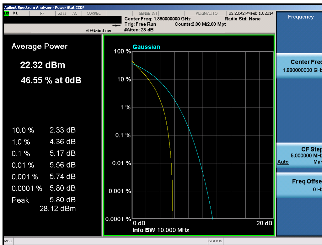
Plot 8-55. PAR Plot (10.0MHz QPSK – RB Size 50)
