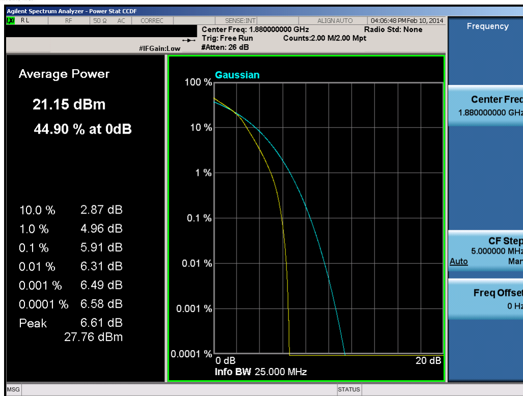
Plot 8-84. PAR Plot (20.0MHz 16-QAM - RB Size 100)
