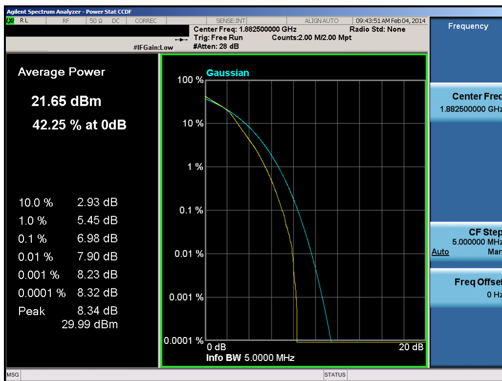
Plot 8-22. PAR Plot (5.0MHz 16-QAM – RB Size 25)
