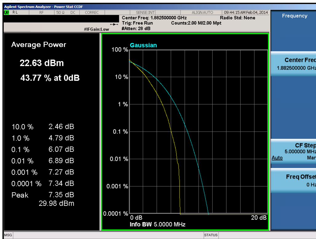
Plot 8-21. PAR Plot (5.0MHz QPSK – RB Size 25)
