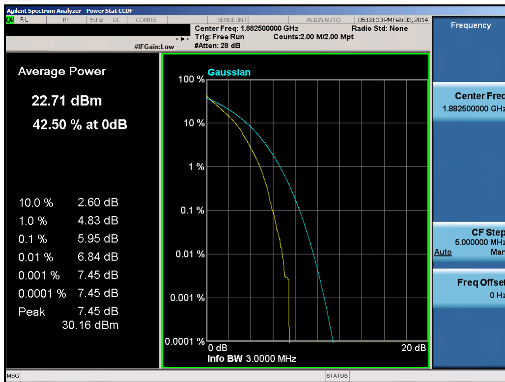
Plot 8-13. PAR Plot (3.0MHz QPSK – RB Size 15)
