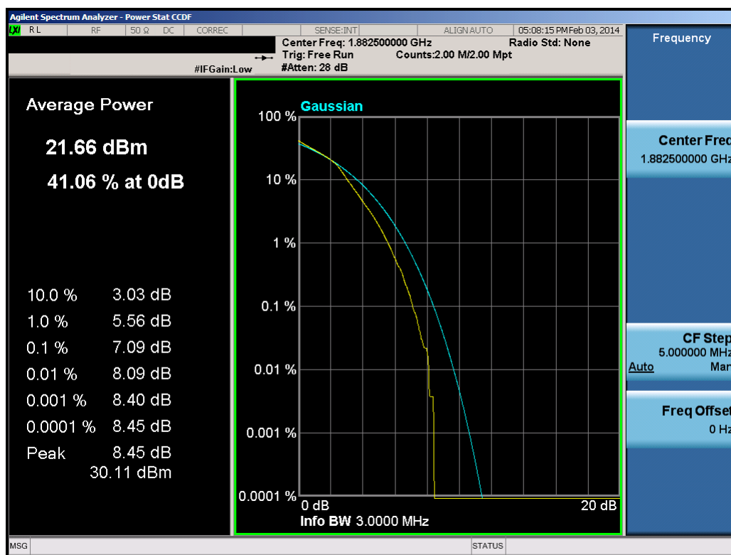
Plot 8-14. PAR Plot (3.0MHz 16-QAM – RB Size 15)
