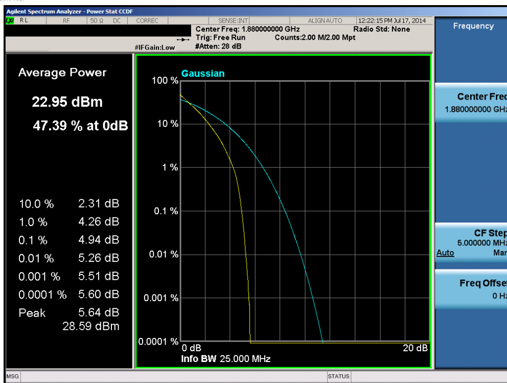
Plot 6-51. PAR Plot (Band 2 – 20.0MHz QPSK – RB Size 100)
