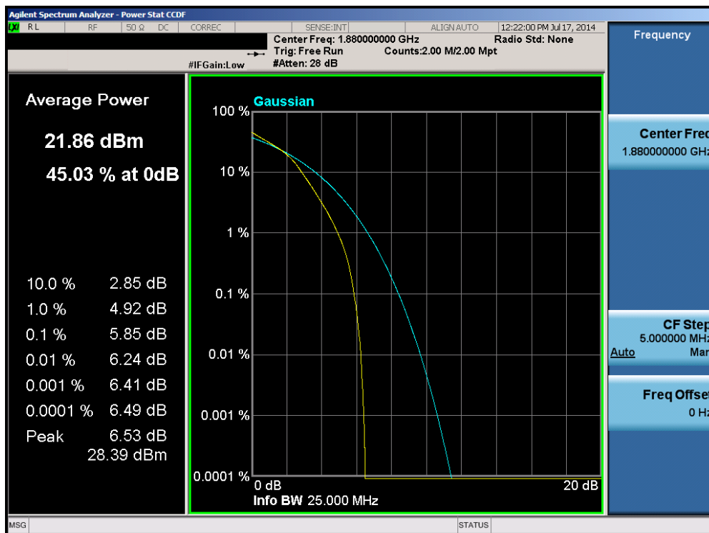
Plot 6-52. PAR Plot (Band 2 – 20.0MHz 16-QAM – RB Size 100)
