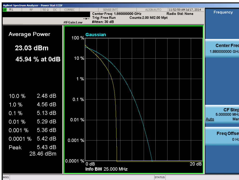
Plot 6-49. PAR Plot (Band 2 – 15.0MHz QPSK – RB Size 75)
