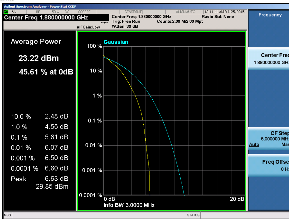
Plot 6-179. PAR Plot (Band 2 – 3.0MHz QPSK – RB Size 15)
