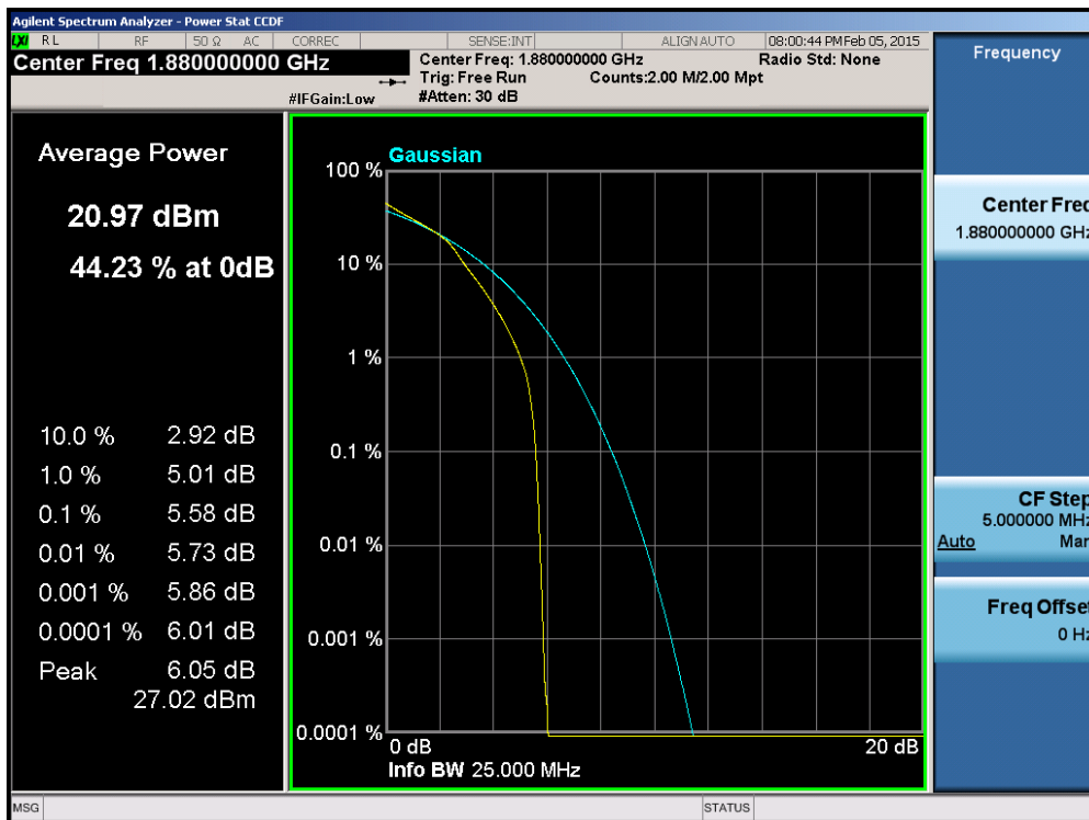
Plot 6-186. PAR Plot (Band 2 – 15.0MHz 16-QAM – RB Size 75)
