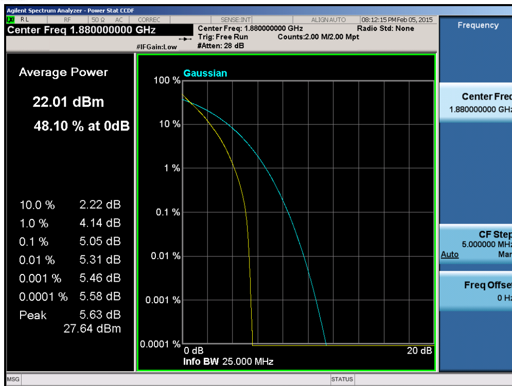
Plot 6-187. PAR Plot (Band 2 – 20.0MHz QPSK – RB Size 100)
