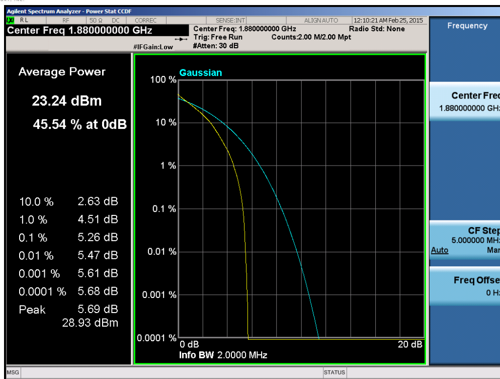
Plot 6-177. PAR Plot (Band 2 – 1.4MHz QPSK – RB Size 6)
