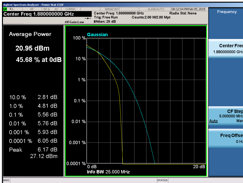
Plot 6-188. PAR Plot (Band 2 – 20.0MHz 16-QAM – RB Size 100)
