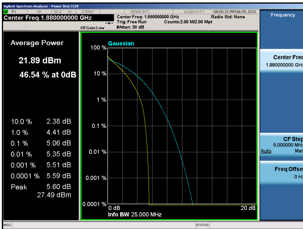
Plot 6-185. PAR Plot (Band 2 – 15.0MHz QPSK – RB Size 75)
