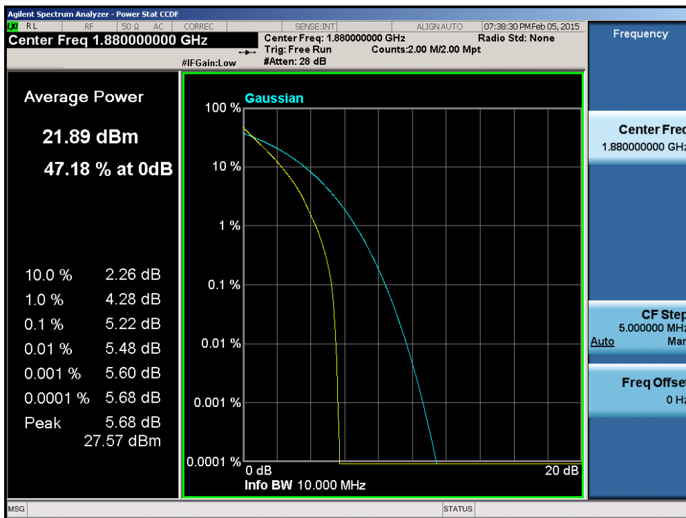
Plot 6-183. PAR Plot (Band 2 – 10.0MHz QPSK – RB Size 50)
