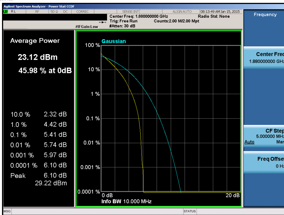
Plot 6-165. PAR Plot (Band 2 – 10.0MHz QPSK – RB Size 50)
