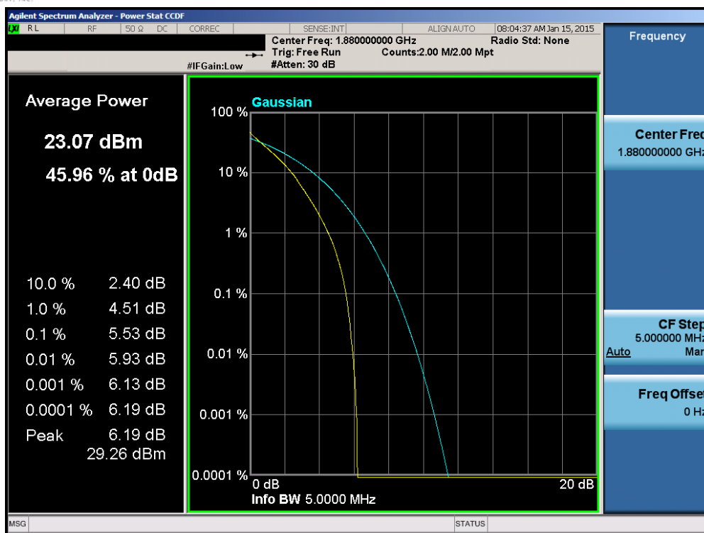
Plot 6-163. PAR Plot (Band 2 – 5.0MHz QPSK – RB Size 25)
