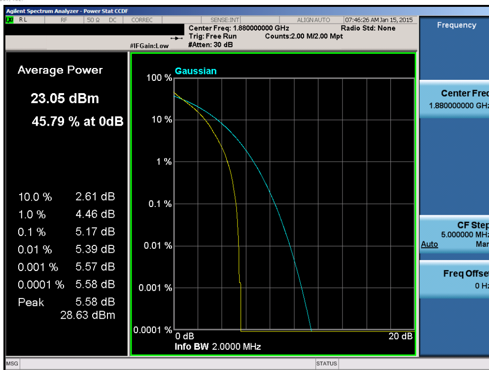
Plot 6-159. PAR Plot (Band 2 – 1.4MHz QPSK – RB Size 6)
