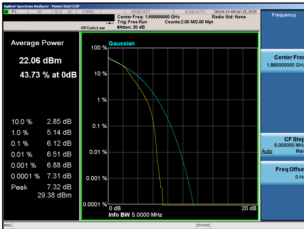
Plot 6-164. PAR Plot (Band 2 – 5.0MHz 16-QAM – RB Size 25)
