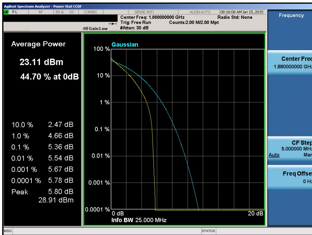
Plot 6-167. PAR Plot (Band 2 – 15.0MHz QPSK – RB Size 75)
