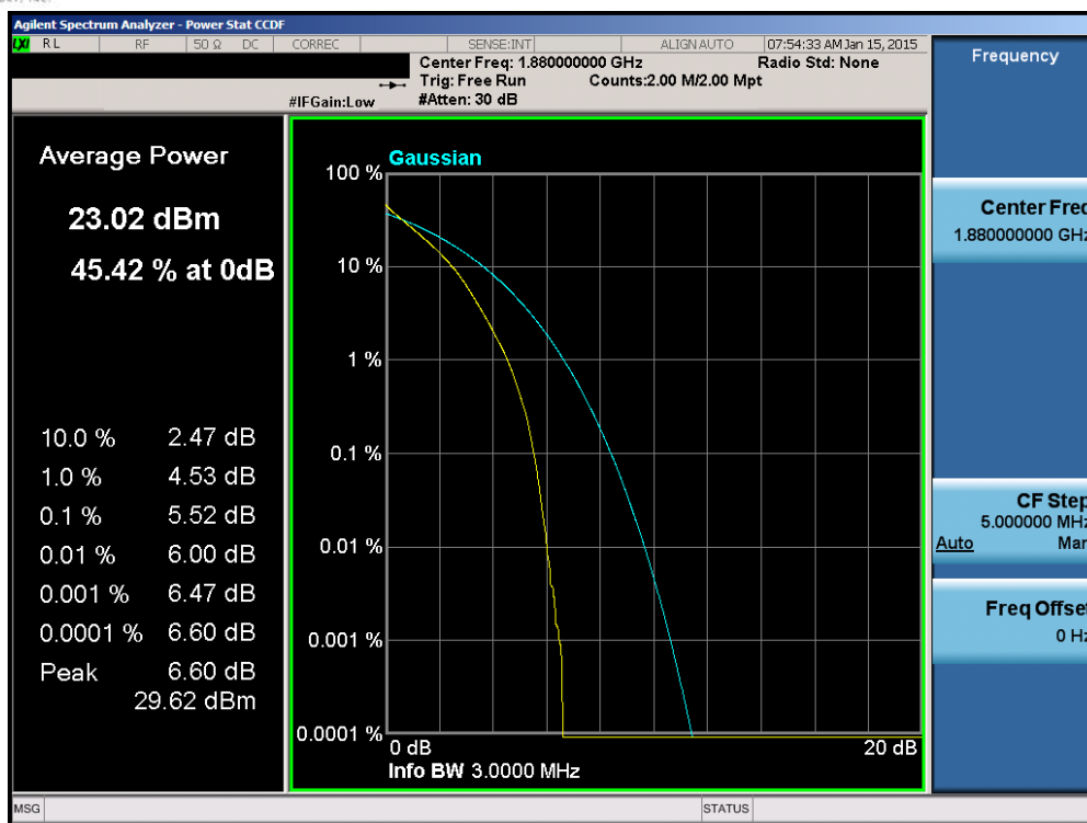
Plot 6-161. PAR Plot (Band 2 – 3.0MHz QPSK – RB Size 15)
