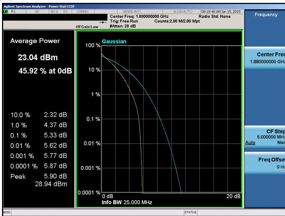
Plot 6-169. PAR Plot (Band 2 – 20.0MHz QPSK – RB Size 100)
