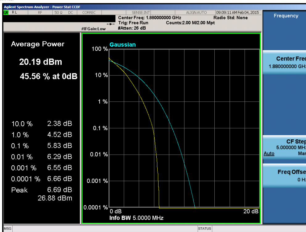
Plot 6-151. PAR Plot (Band 2 – 5.0MHz QPSK – RB Size 25)
