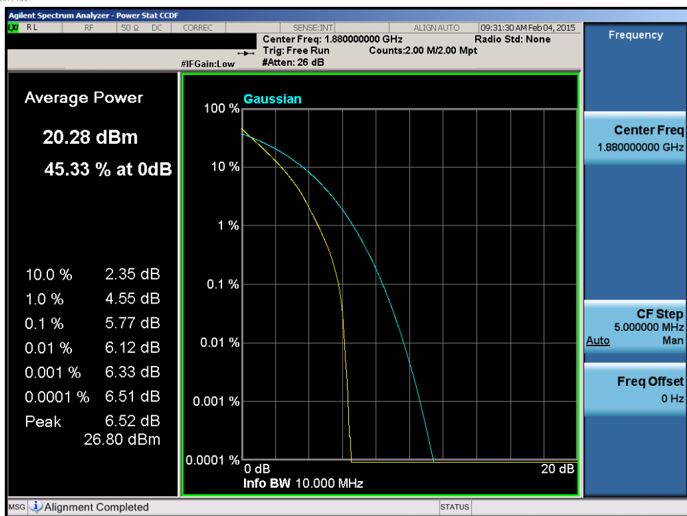
Plot 6-153. PAR Plot (Band 2 – 10.0MHz QPSK – RB Size 50)
