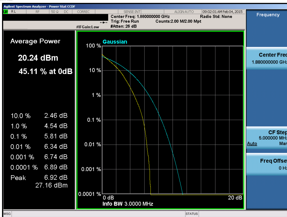
Plot 6-149. PAR Plot (Band 2 – 3.0MHz QPSK – RB Size 15)
