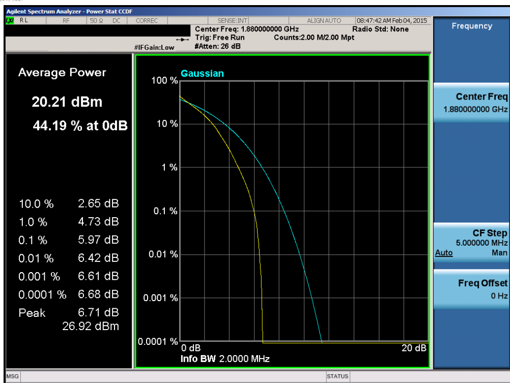
Plot 6-147. PAR Plot (Band 2 – 1.4MHz QPSK – RB Size 6)
