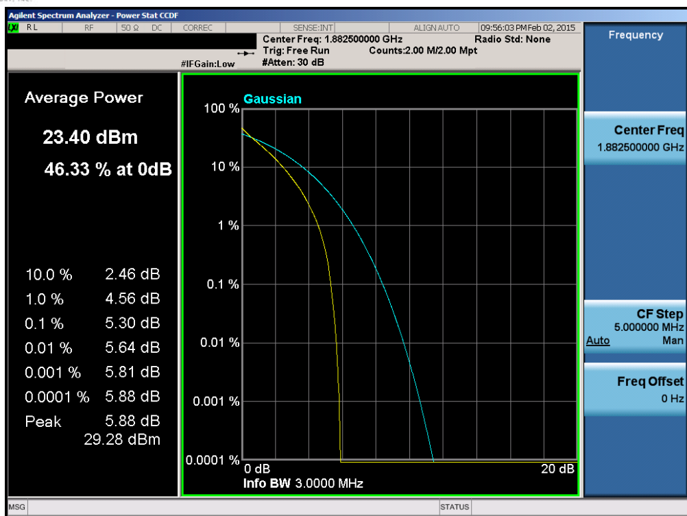
Plot 6-172. PAR Plot (Band 25 – 3.0MHz QPSK – RB Size 15)
