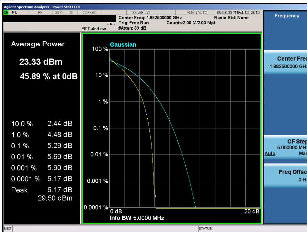
Plot 6-174. PAR Plot (Band 25 – 5.0MHz QPSK – RB Size 25)
