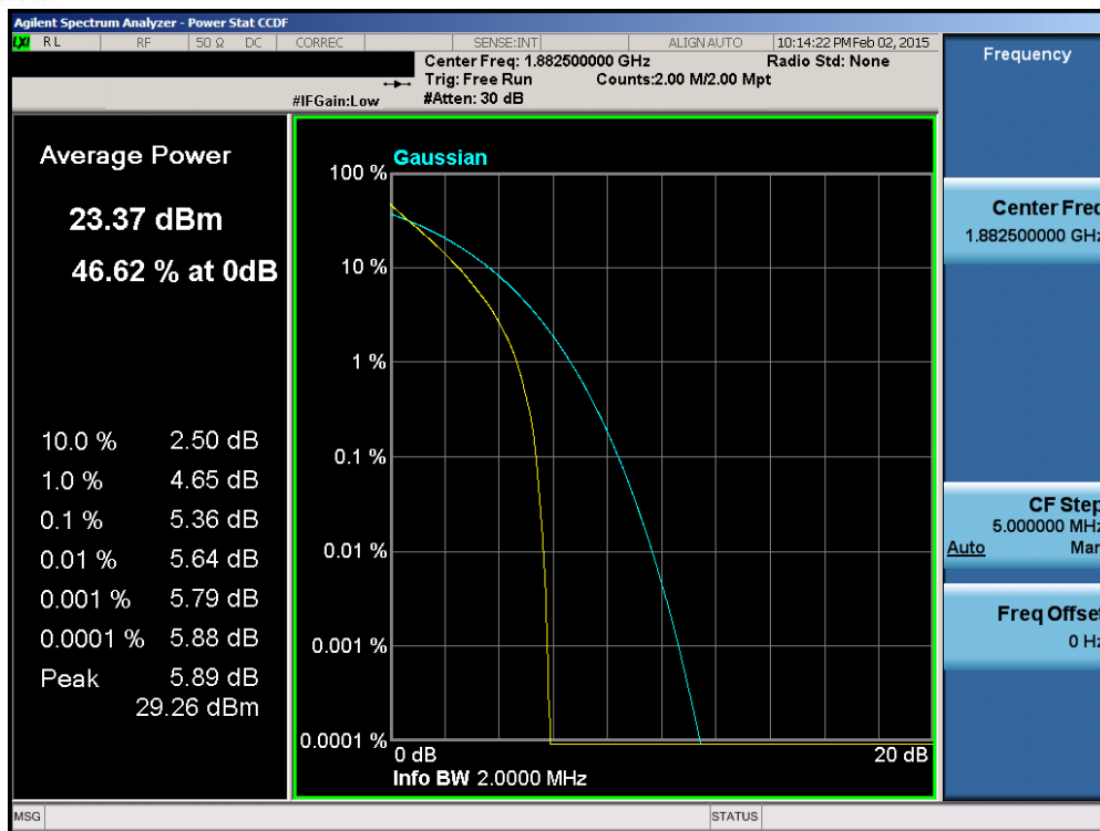
Plot 6-170. PAR Plot (Band 25 – 1.4MHz QPSK – RB Size 6)
