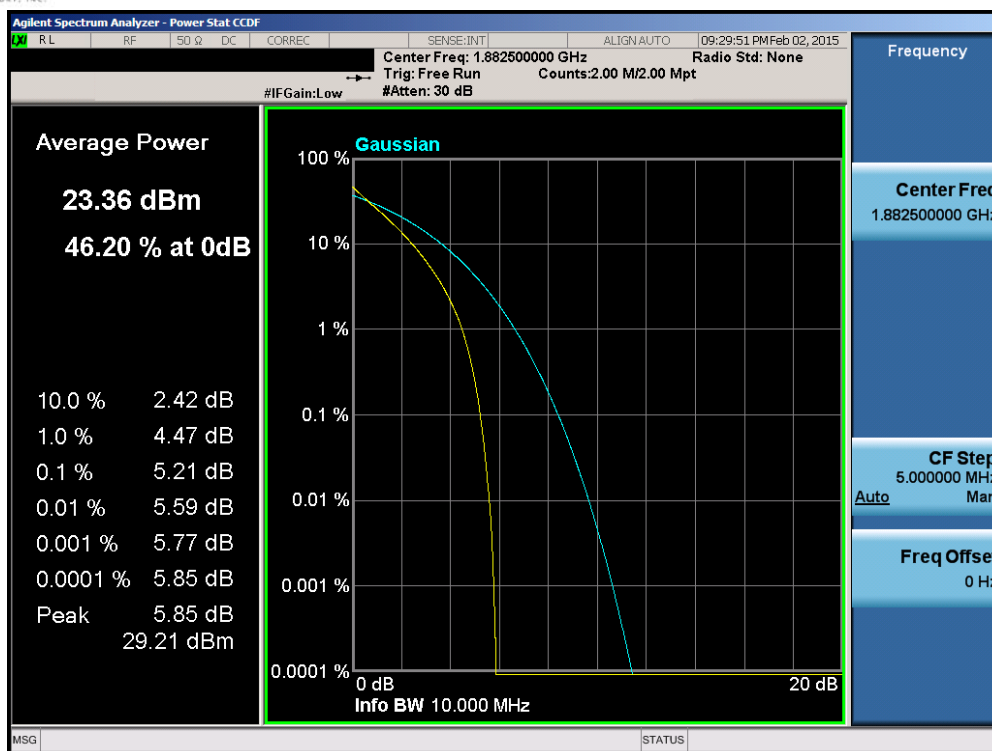
Plot 6-176. PAR Plot (Band 25 – 10.0MHz QPSK – RB Size 50)
