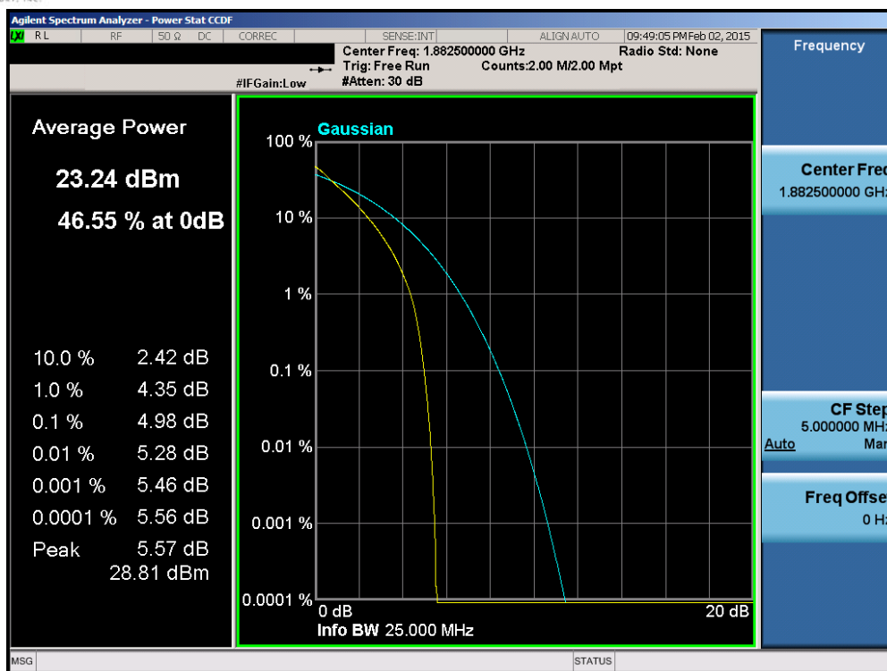
Plot 6-180. PAR Plot (Band 25 – 20.0MHz QPSK – RB Size 100)
