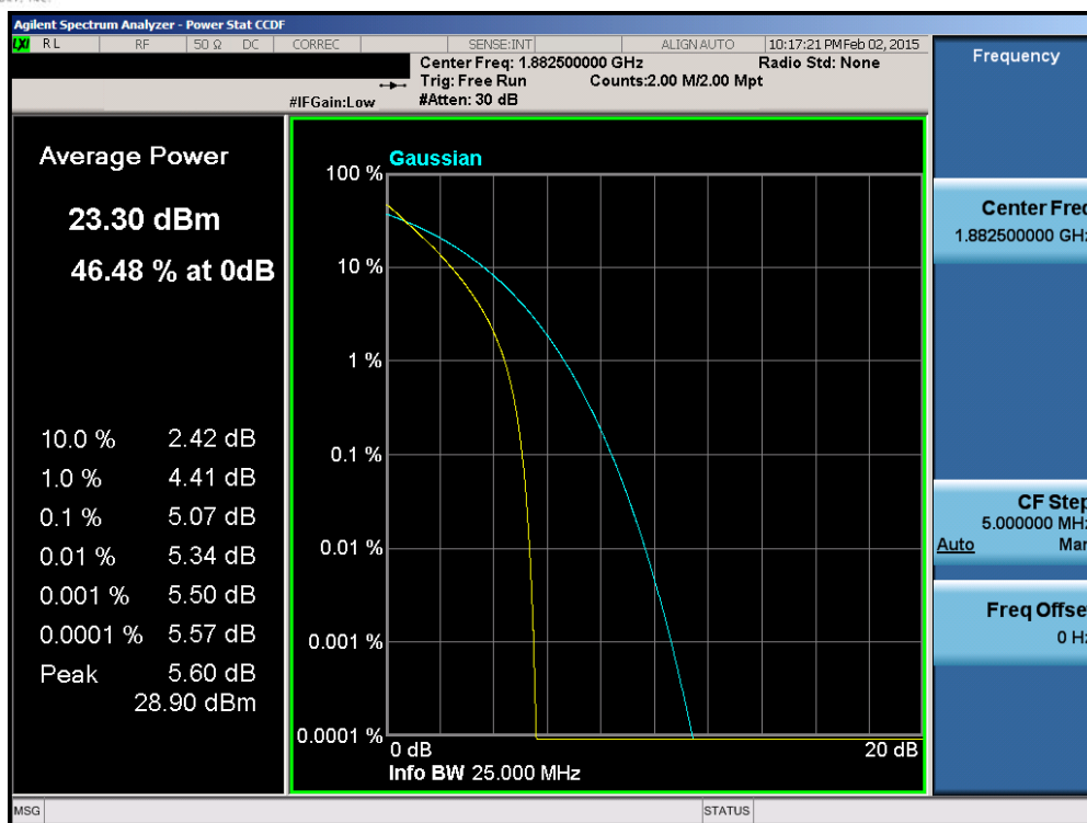
Plot 6-178. PAR Plot (Band 25 – 15.0MHz QPSK – RB Size 75)
