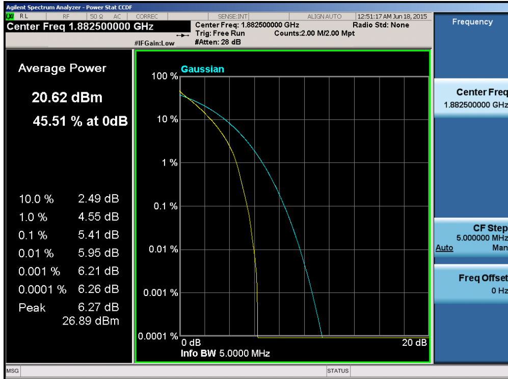
Plot 6-159. PAR Plot (Band 25/2 – 5.0MHz QPSK – RB Size 25)
