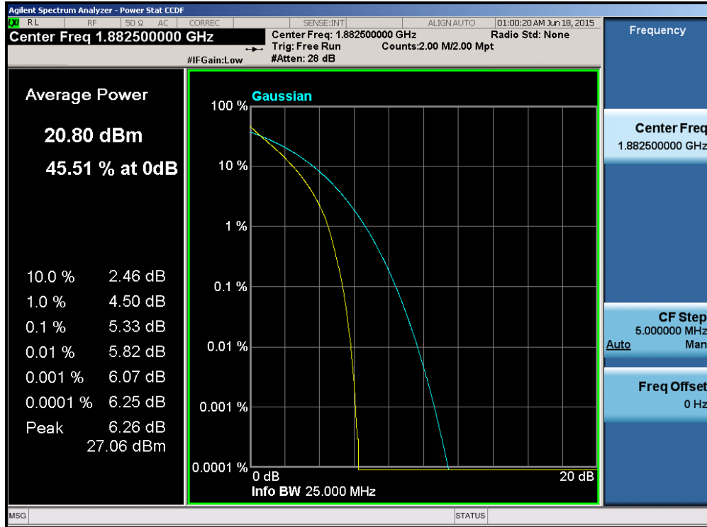
Plot 6-165. PAR Plot (Band 25/2 – 20.0MHz QPSK – RB Size 100)
