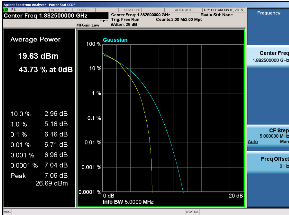
Plot 6-160. PAR Plot (Band 25/2 – 5.0MHz 16-QAM – RB Size 25)
