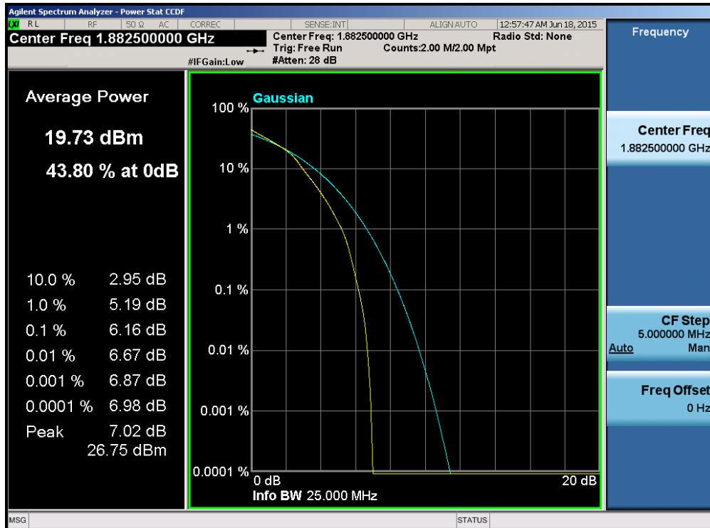
Plot 6-164. PAR Plot (Band 25/2 – 15.0MHz 16-QAM – RB Size 75)
