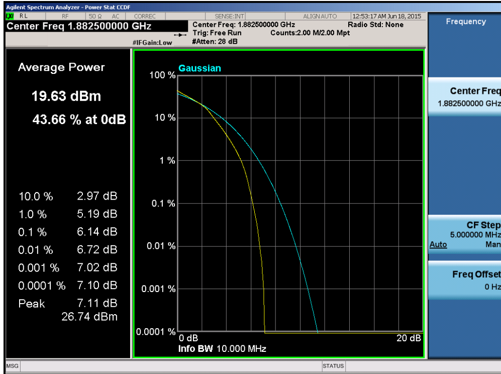
Plot 6-161. PAR Plot (Band 25/2 – 10.0MHz QPSK – RB Size 50)
