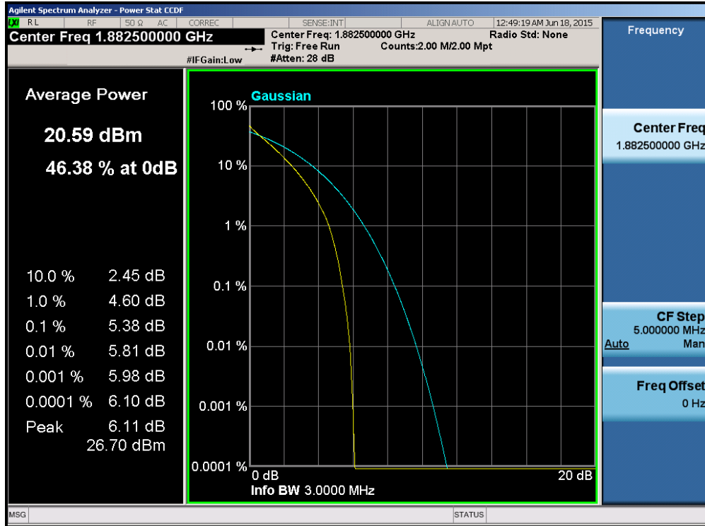
Plot 6-157. PAR Plot (Band 25/2 – 3.0MHz QPSK – RB Size 15)
