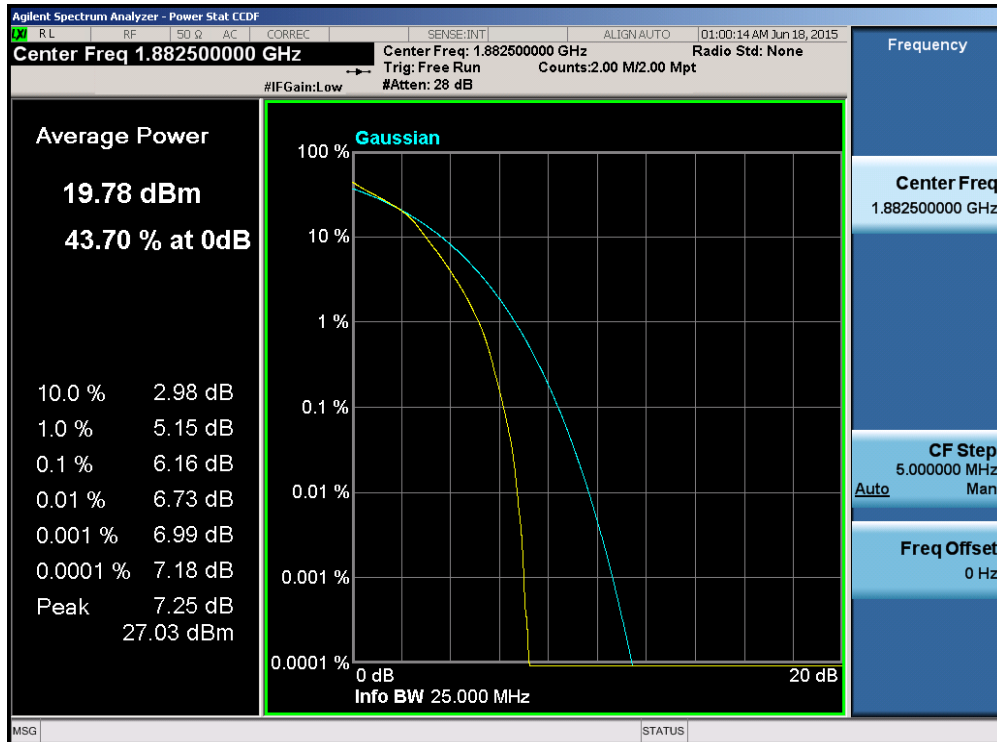
Plot 6-166. PAR Plot (Band 25/2 – 20.0MHz 16-QAM – RB Size 100)
