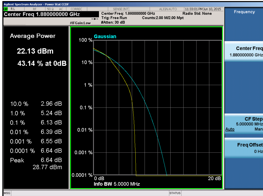
Plot 6-193. PAR Plot (Band 2 - 5.0MHz 16-QAM - RB Size 25)
