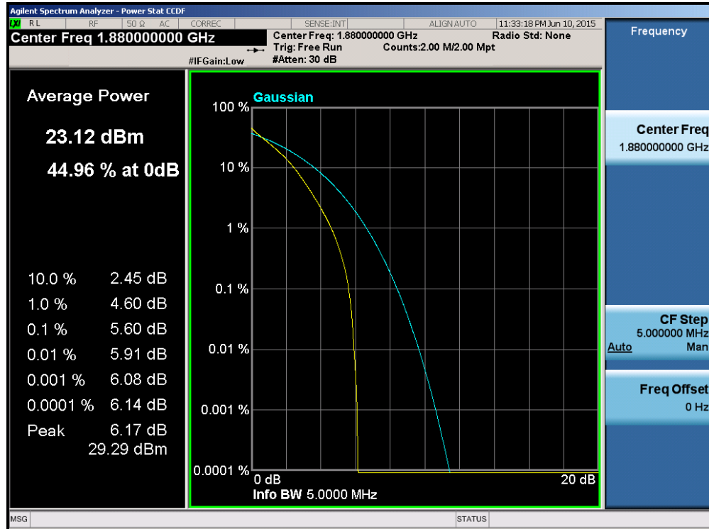
Plot 6-192. PAR Plot (Band 2 - 5.0MHz QPSK - RB Size 25)
