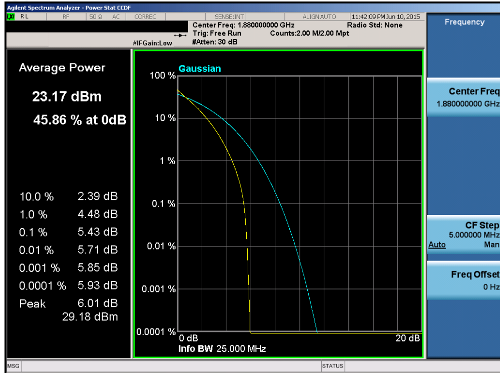
Plot 6-198. PAR Plot (Band 2 – 20.0MHz QPSK – RB Size 100)
