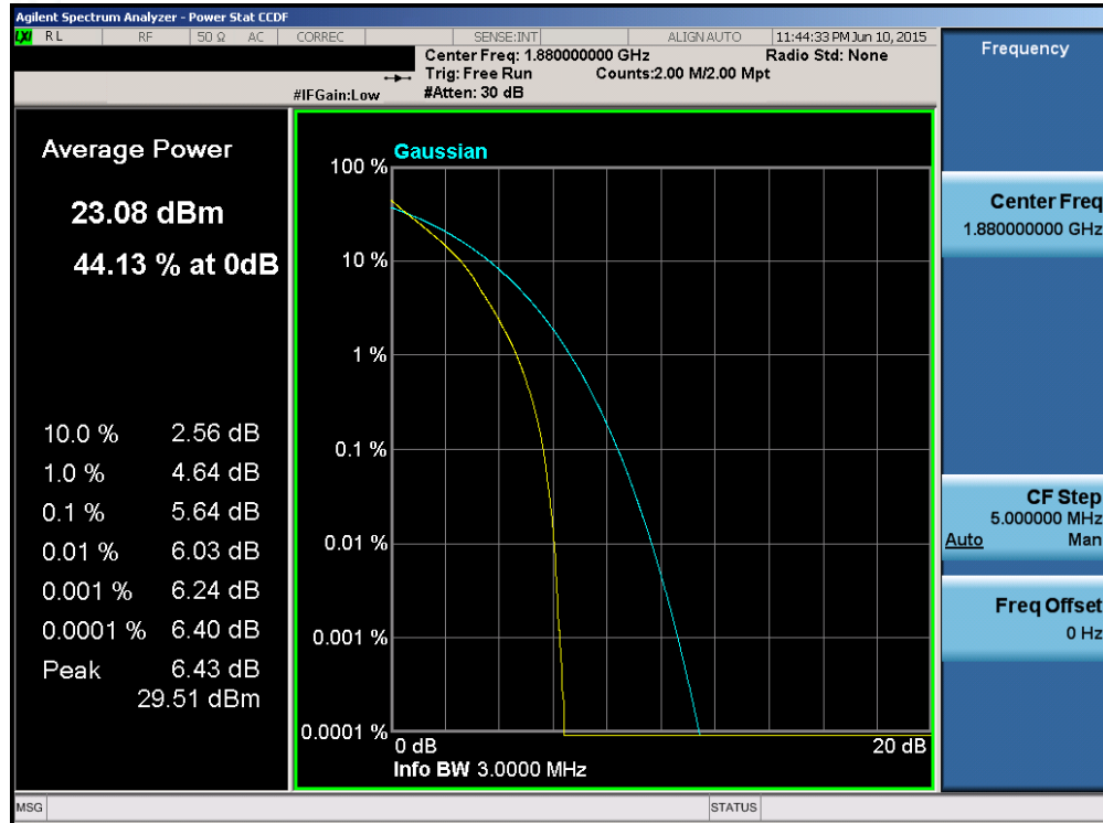
Plot 6-190. PAR Plot (Band 2 – 3.0MHz QPSK – RB Size 15)
