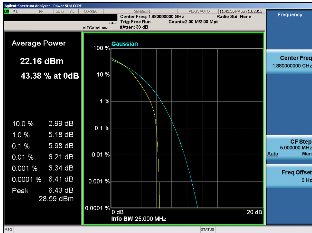
Plot 6-199. PAR Plot (Band 2 – 20.0MHz 16-QAM – RB Size 100)
