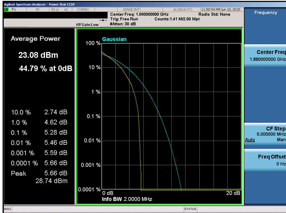
Plot 6-188. PAR Plot (Band 2 – 1.4MHz QPSK – RB Size 6)
