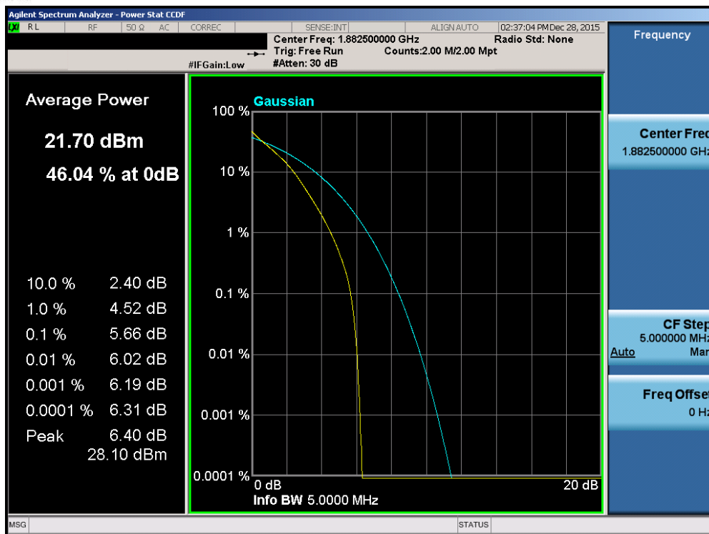
Plot 7-242. PAR Plot (Band 2/25 – 5.0MHz QPSK – RB Size 25)
