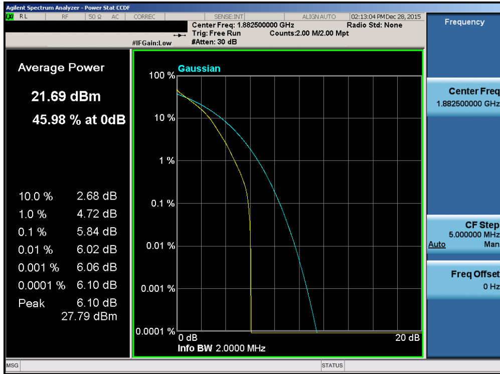
Plot 7-238. PAR Plot (Band 2/25 – 1.4MHz QPSK – RB Size 6)
