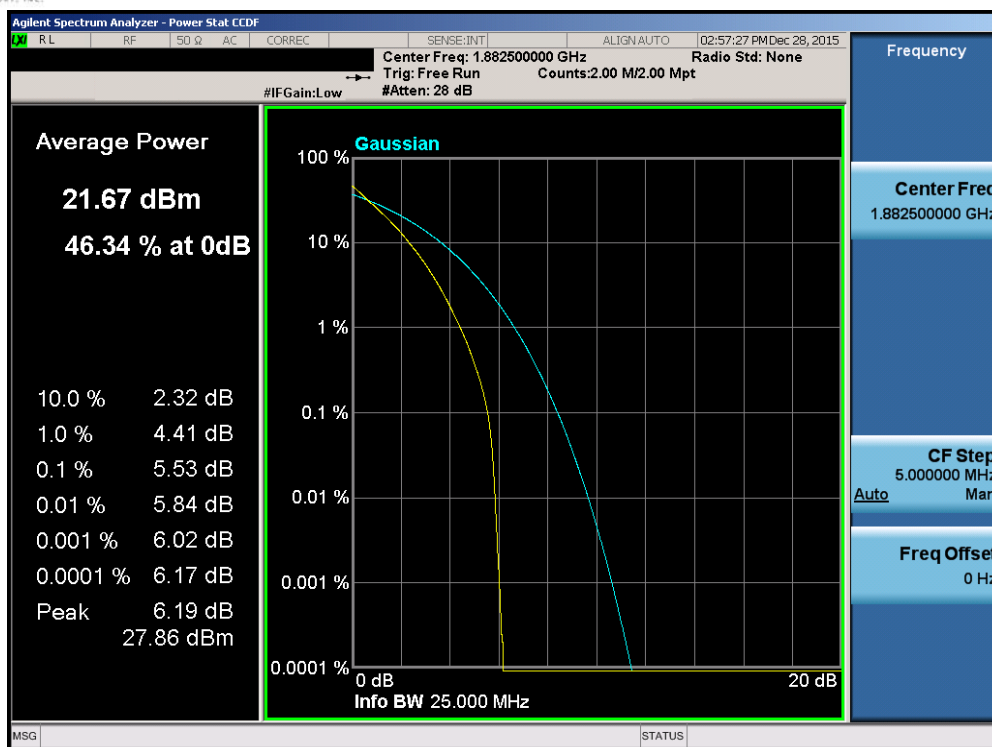
Plot 7-248. PAR Plot (Band 2/25 – 20.0MHz QPSK – RB Size 100)
