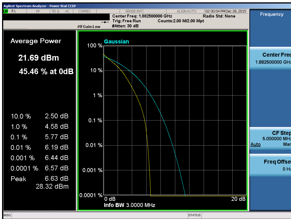
Plot 7-240. PAR Plot (Band 2/25 – 3.0MHz QPSK – RB Size 15)
