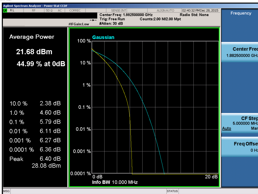
Plot 7-244. PAR Plot (Band 2/25 – 10.0MHz QPSK – RB Size 50)
