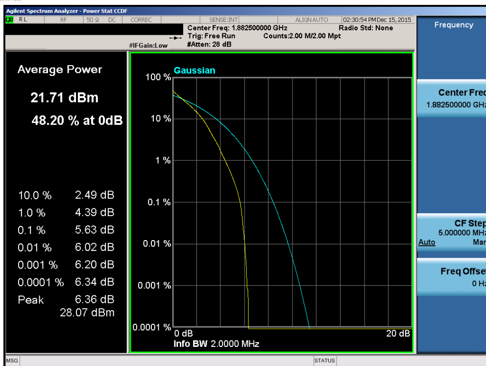
Plot 7-213. PAR Plot (Band2/25 – 1.4MHz QPSK – RB Size 6)
