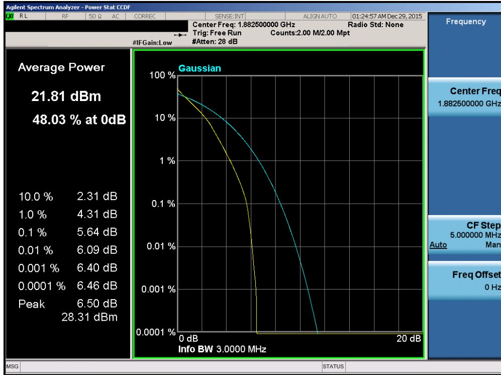
Plot 7-238. PAR Plot (Band 2/25 – 3.0MHz QPSK – RB Size 15)
