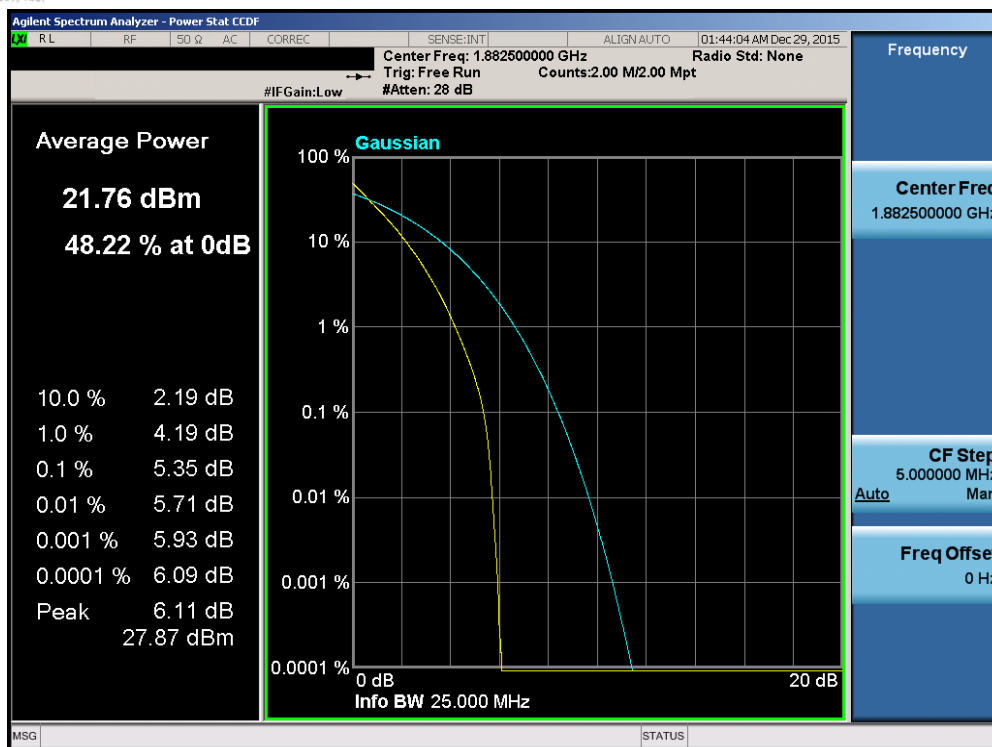
Plot 7-246. PAR Plot (Band 2/25 - 20.0MHz QPSK - RB Size 100)
