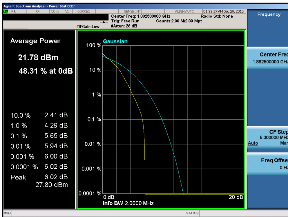
Plot 7-236. PAR Plot (Band 2/25 - 1.4MHz QPSK - RB Size 6)
