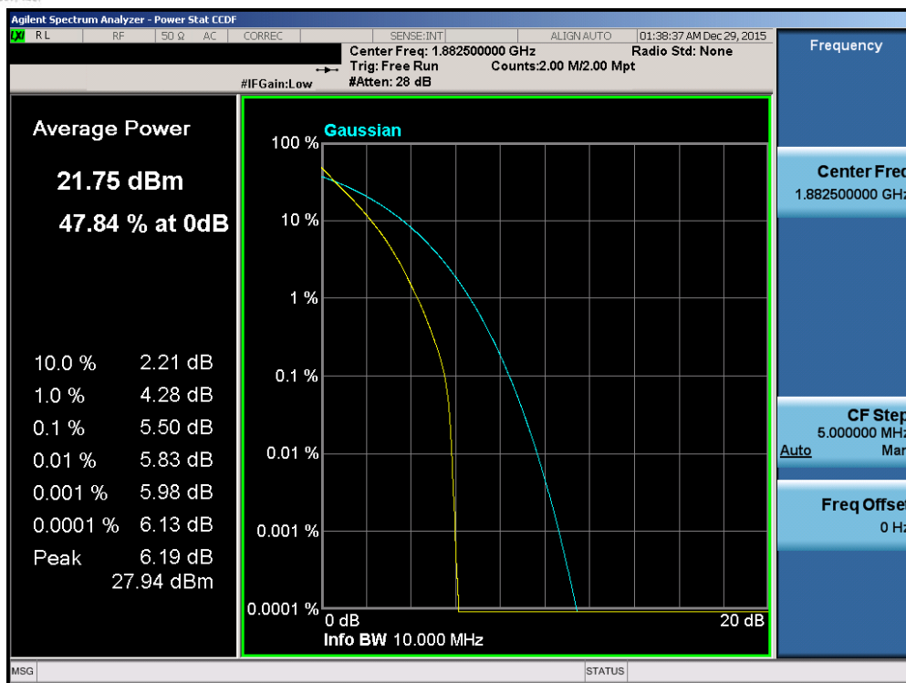
Plot 7-242. PAR Plot (Band 2/25 - 10.0MHz QPSK - RB Size 50)
