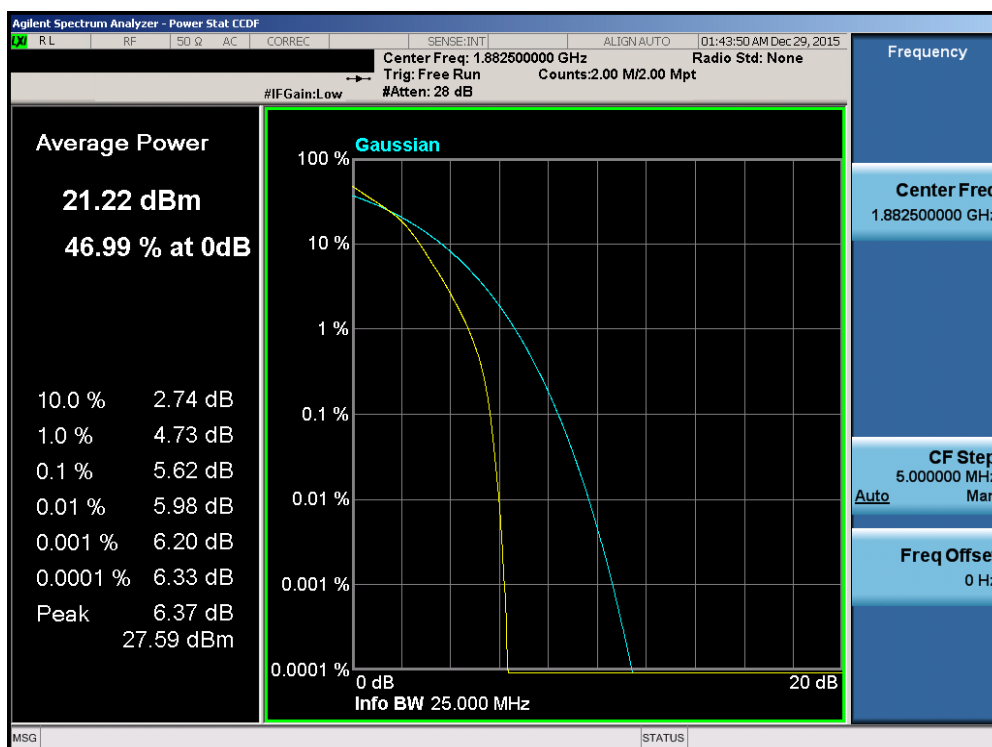
Plot 7-247. PAR Plot (Band 2/25 - 20.0MHz 16-QAM - RB Size 100)
