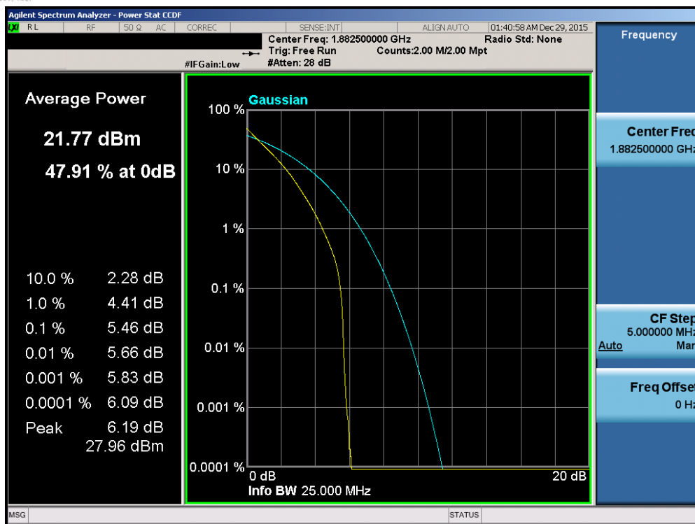
Plot 7-244. PAR Plot (Band 2/25 – 15.0MHz QPSK – RB Size 75)
