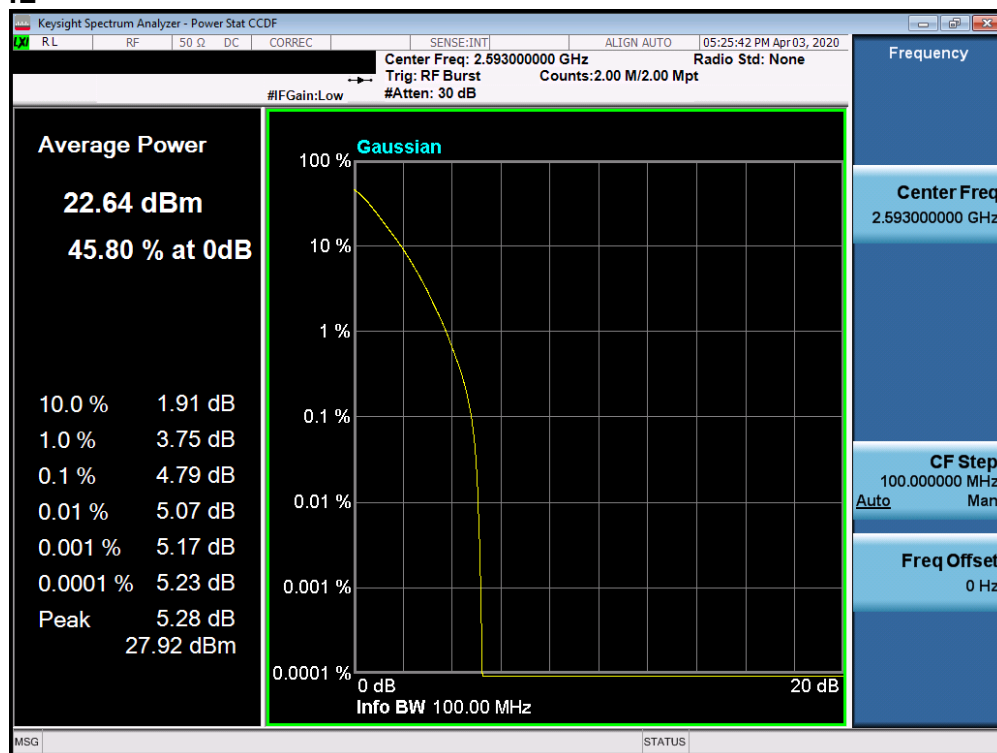
Plot 7-87. PAR Plot (Band n41 - 100.0MHz DFT-s-OFDM-BPSK - Full RB Configuration)
