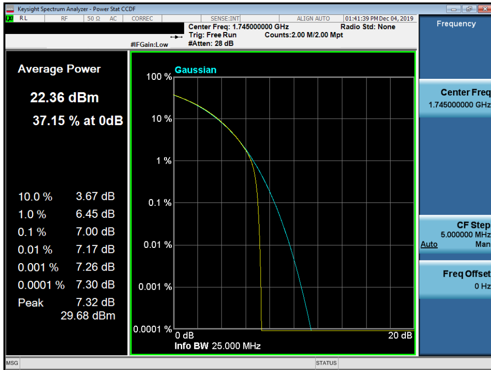
Plot 7-742. PAR Plot (Band n66 - 20.0MHz CP-OFDM-QPSK - Full RB Configuration)
