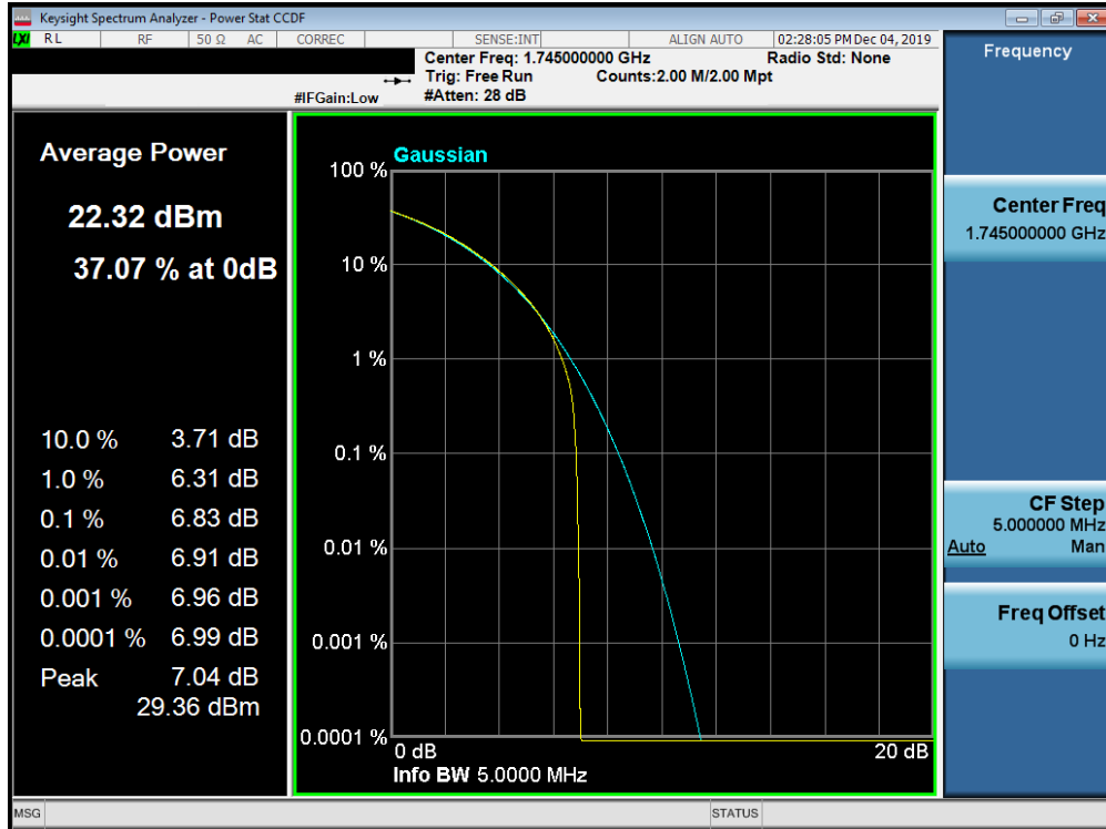
Plot 7-730. PAR Plot (Band n66 - 5.0MHz CP-OFDM-QPSK - Full RB Configuration)
