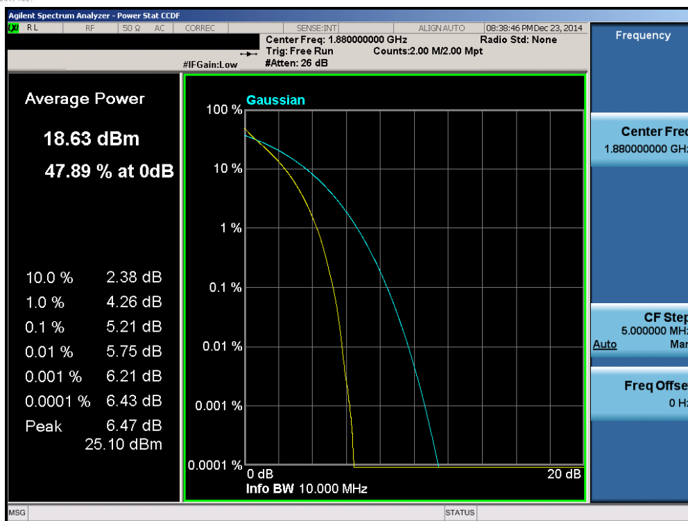
Plot 6-95. PAR Plot (Band 2 – 10.0MHz QPSK – RB Size 50)
