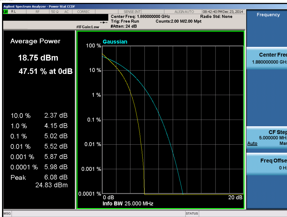
Plot 6-97. PAR Plot (Band 2 – 15.0MHz QPSK – RB Size 75)
