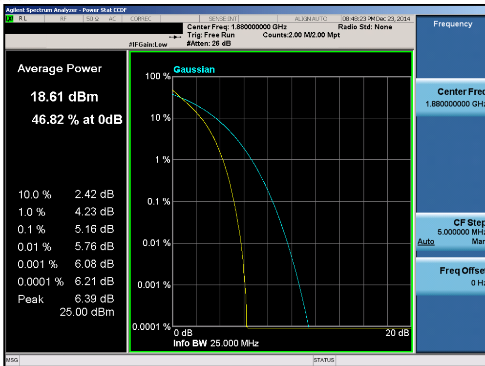
Plot 6-99. PAR Plot (Band 2 – 20.0MHz QPSK – RB Size 100)
