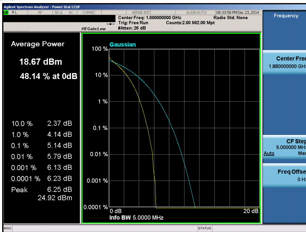
Plot 6-93. PAR Plot (Band 2 – 5.0MHz QPSK – RB Size 25)
