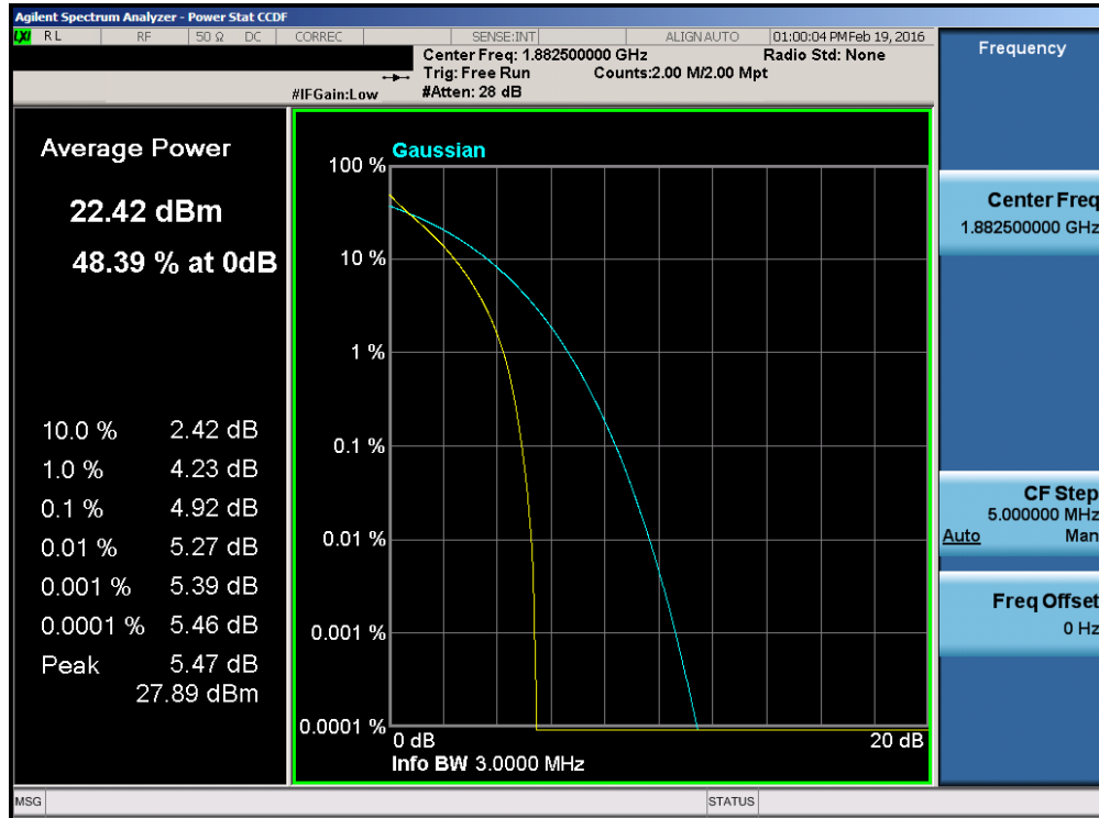
Plot 7-102. PAR Plot (Band 25 – 3.0MHz QPSK – RB Size 15)
