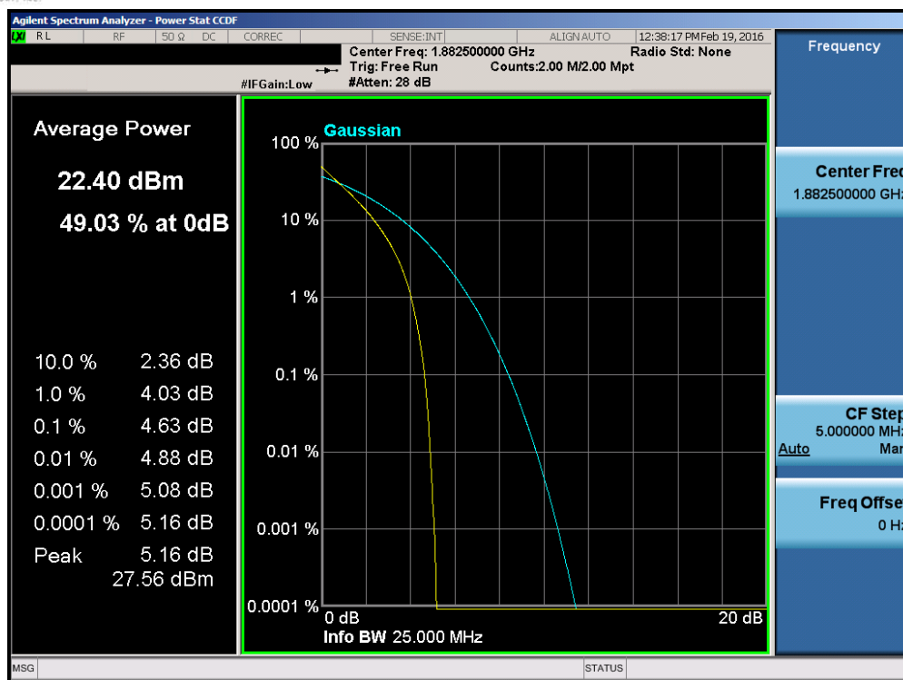
Plot 7-108. PAR Plot (Band 25 – 15.0MHz QPSK – RB Size 75)
