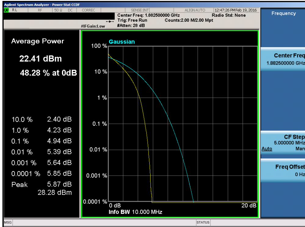
Plot 7-106. PAR Plot (Band 25 – 10.0MHz QPSK – RB Size 50)
