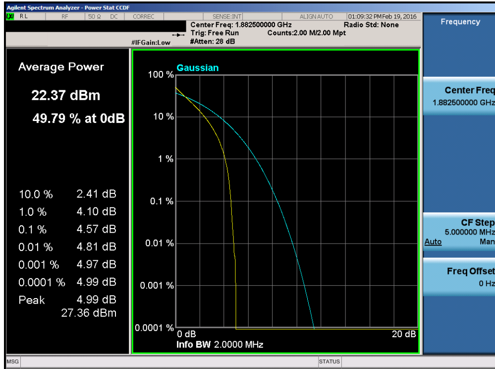
Plot 7-100. PAR Plot (Band 25 – 1.4MHz QPSK – RB Size 6)
