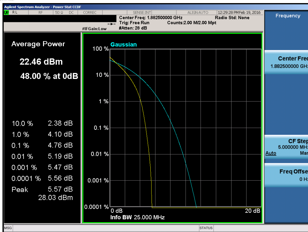
Plot 7-110. PAR Plot (Band 25 – 20.0MHz QPSK – RB Size 100)
