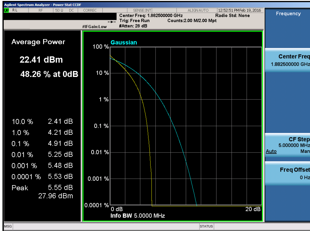
Plot 7-104. PAR Plot (Band 25 – 5.0MHz QPSK – RB Size 25)
