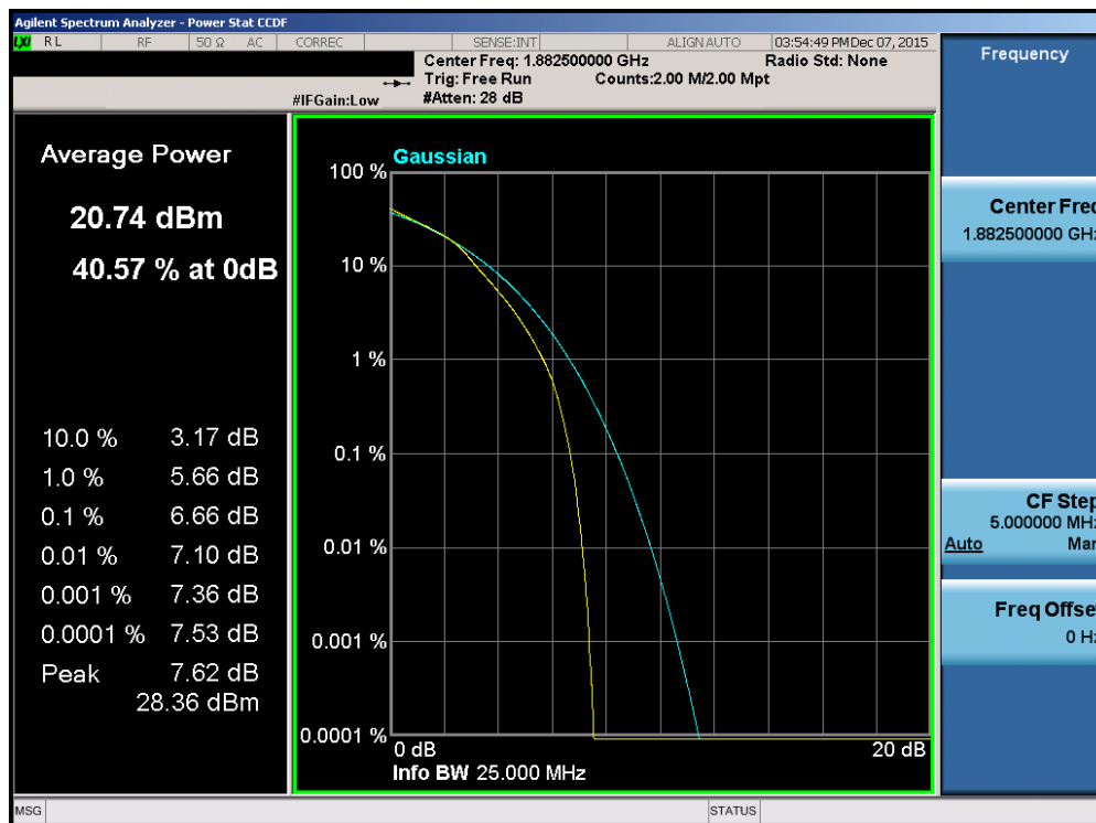
Plot 7-193. PAR Plot (Band 2/25 – 15.0MHz 16-QAM – RB Size 75)
