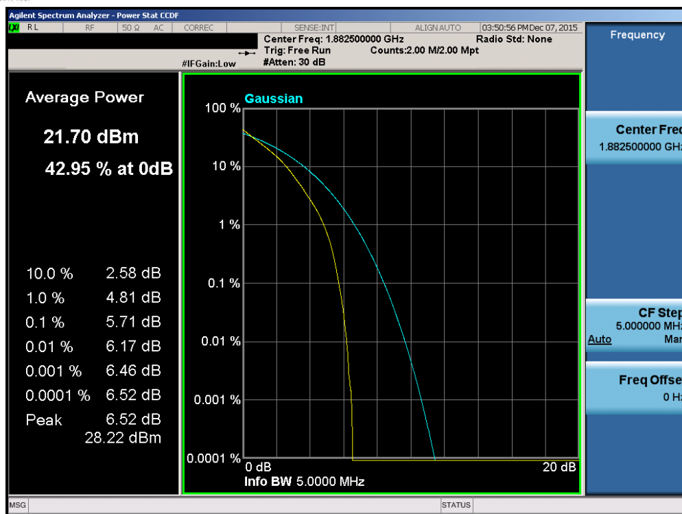
Plot 7-188. PAR Plot (Band 2/25 – 5.0MHz QPSK – RB Size 25)
