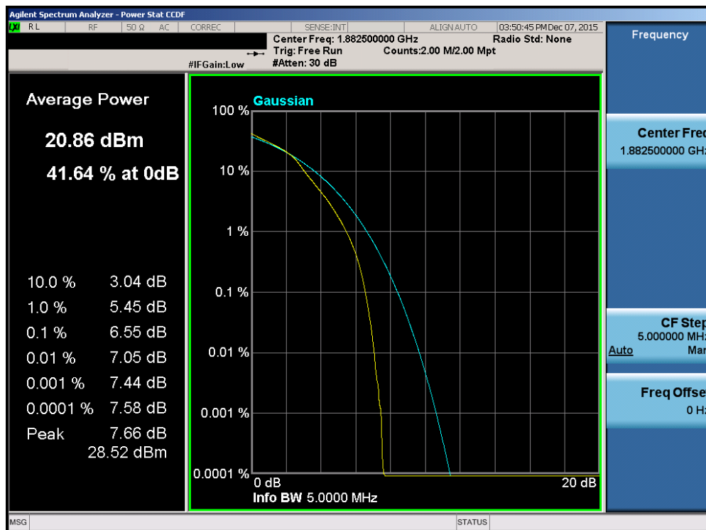
Plot 7-189. PAR Plot (Band 2/25 – 5.0MHz 16-QAM – RB Size 25)
