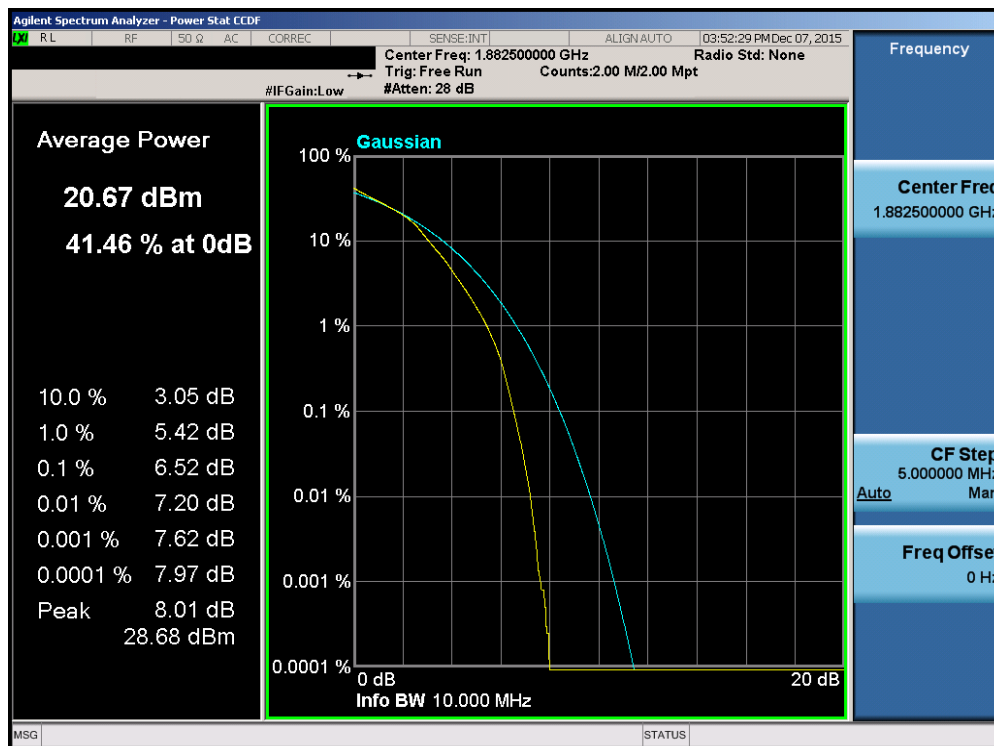
Plot 7-191. PAR Plot (Band 2/25 – 10.0MHz 16-QAM – RB Size 50)
