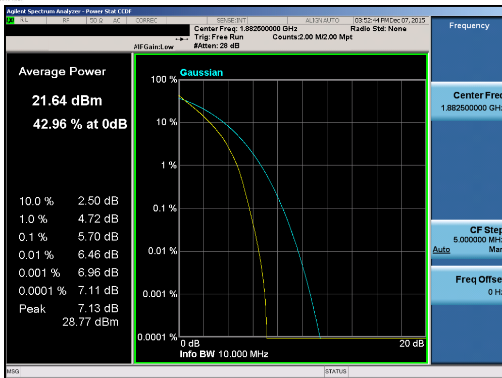
Plot 7-190. PAR Plot (Band 2/25 – 10.0MHz QPSK – RB Size 50)
