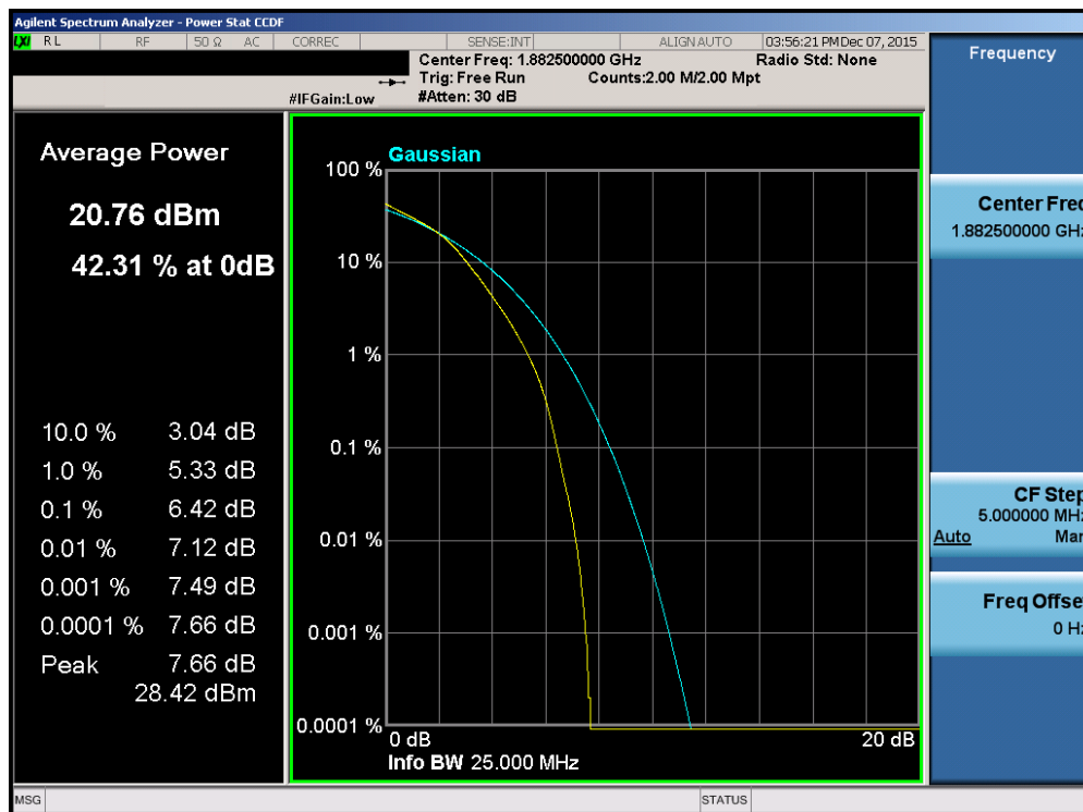
Plot 7-195. PAR Plot (Band 2/25 – 20.0MHz 16-QAM – RB Size 100)
