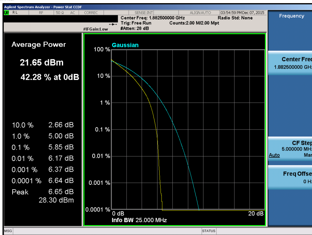
Plot 7-192. PAR Plot (Band 2/25 – 15.0MHz QPSK – RB Size 75)
