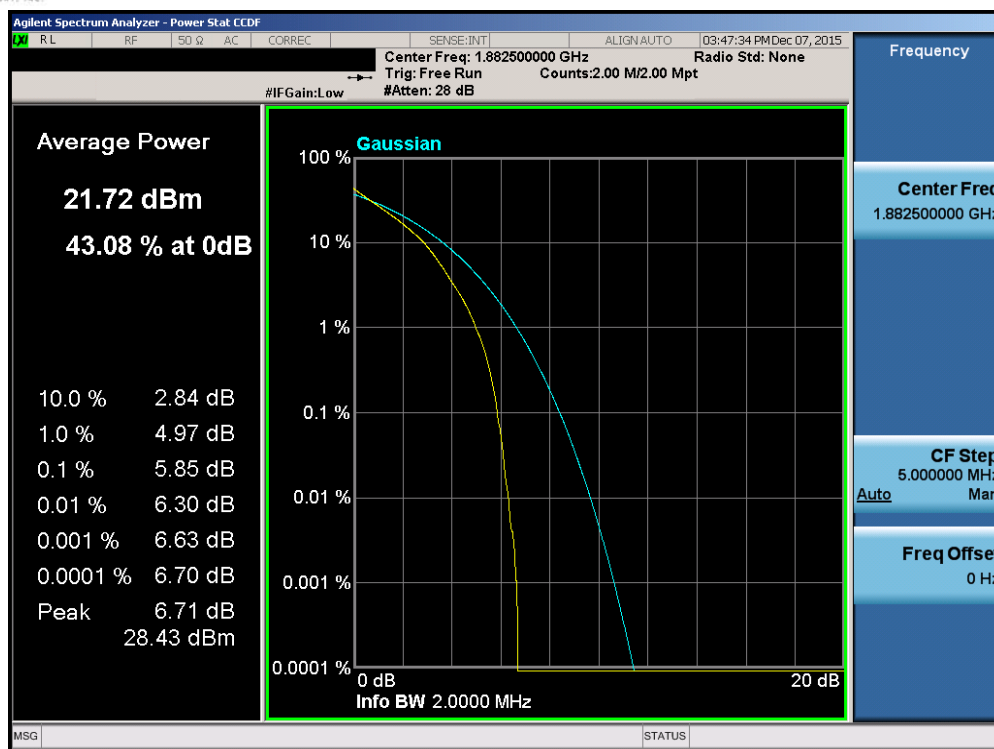
Plot 7-184. PAR Plot (Band 2/25 – 1.4MHz QPSK – RB Size 6)
