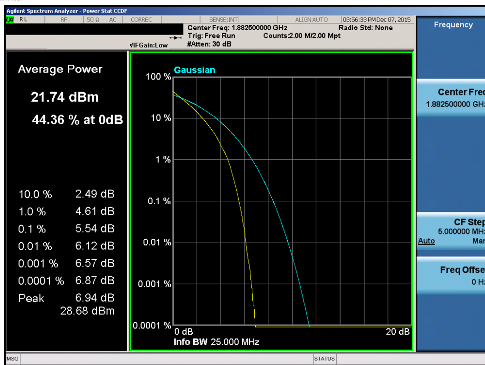
Plot 7-194. PAR Plot (Band 2/25 – 20.0MHz QPSK – RB Size 100)
